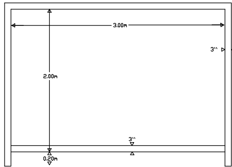
DET. EQUIP. FUTEBOL ESCALA.....1/25
