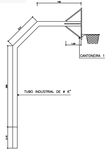
DET. DA ESTRUTURA DE FERRO DA TABELA ESCALA.....1/25
