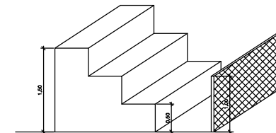
DET. ARQUIBANCADE E ALAMBRADO ESCALA 1/75
