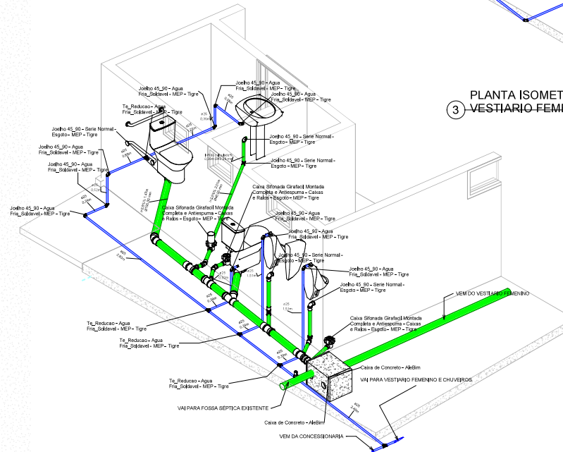
PLANTA ISOMETRICA
