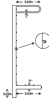
DET. EQUIP. FUTEBOL ESCALA.....1/25
