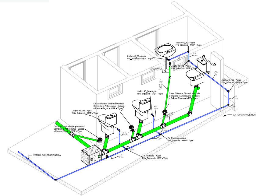
3 PLANTA ISOMETRICA VESTIÁRIO FEMENINO
