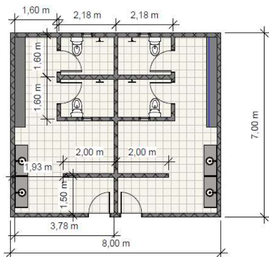
VESTIÁRIOS E BANHEIROS
