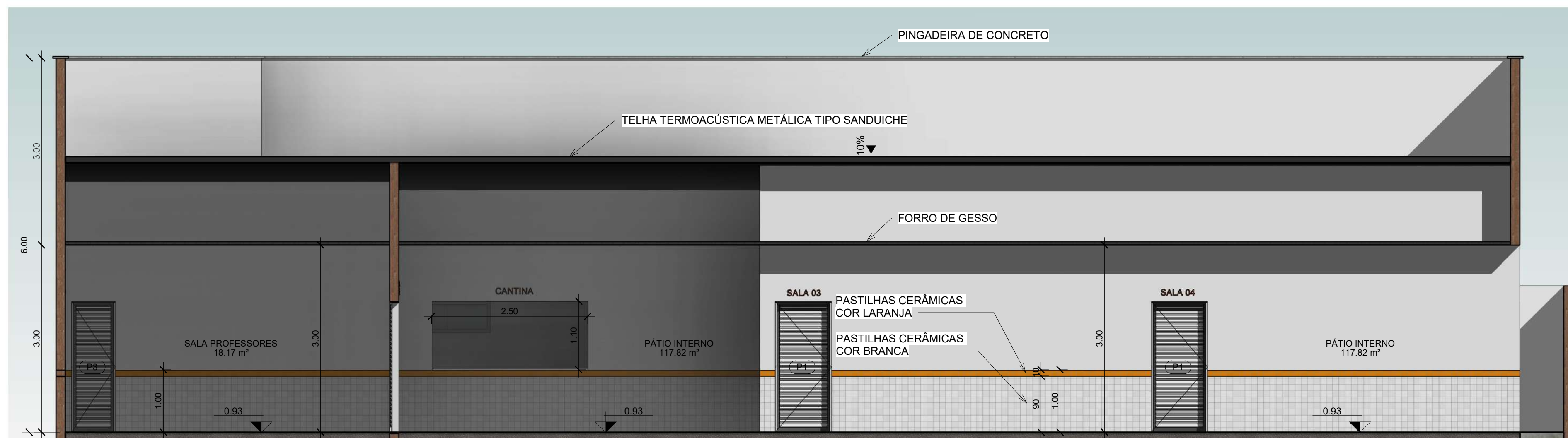
1 CORTE A-A 1 : 50
