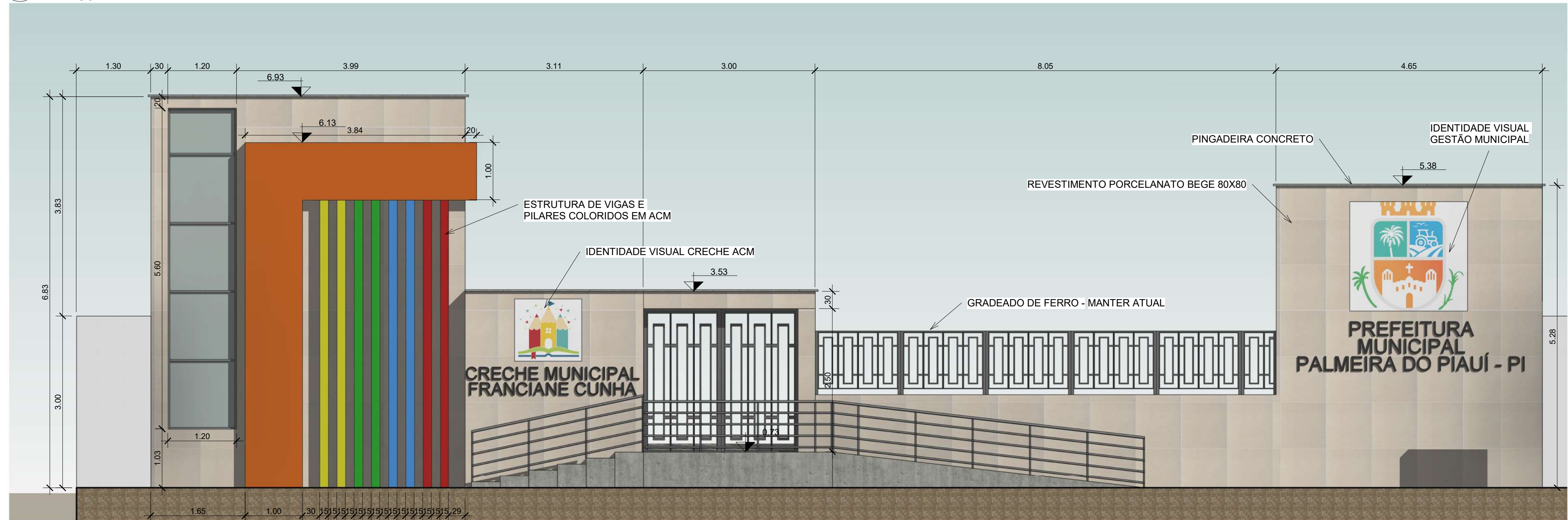
2 FACHADA EXTERNA - MURO 1 : 50
