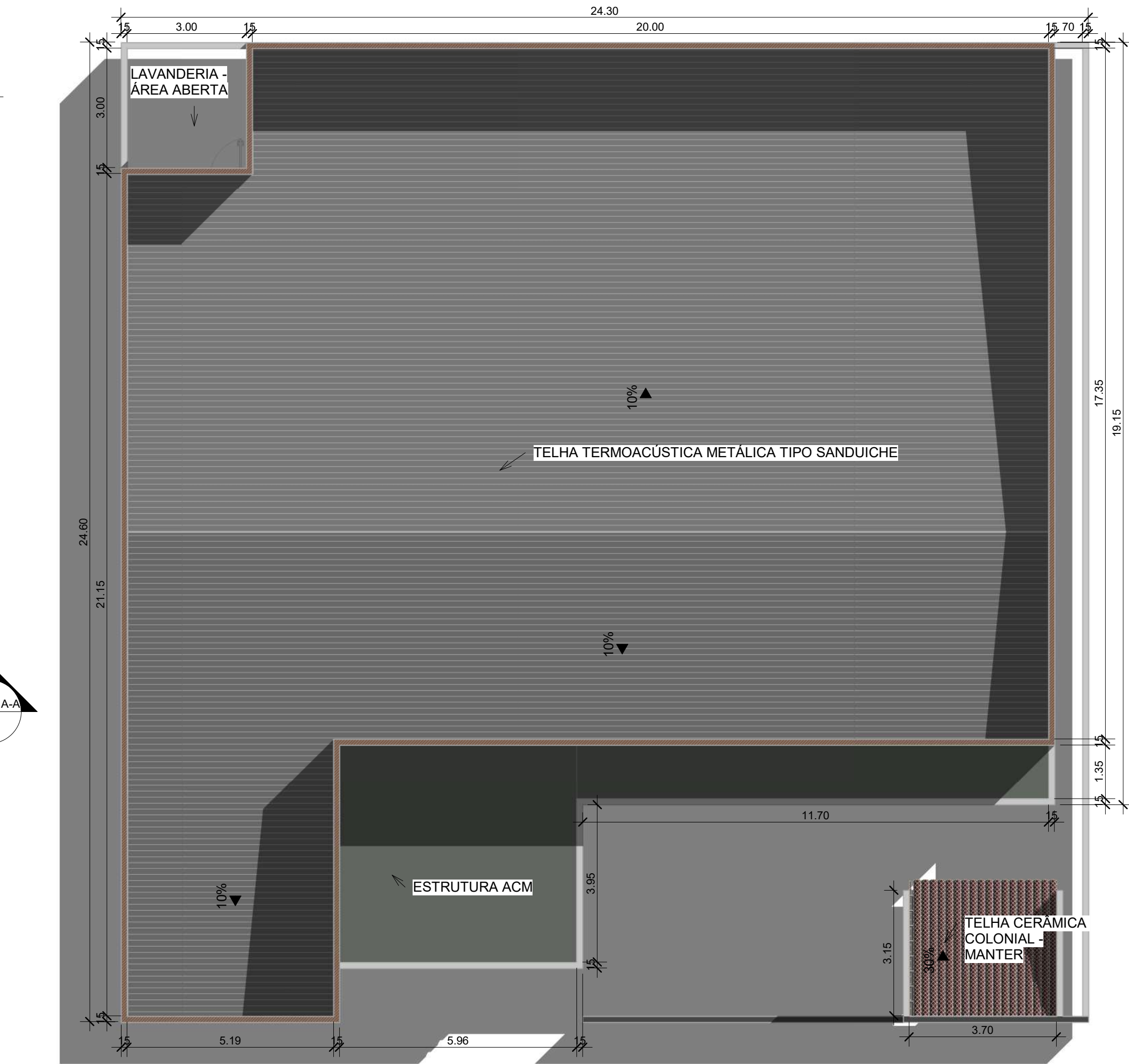
2 PLANTA COBERTURA 1 : 100
