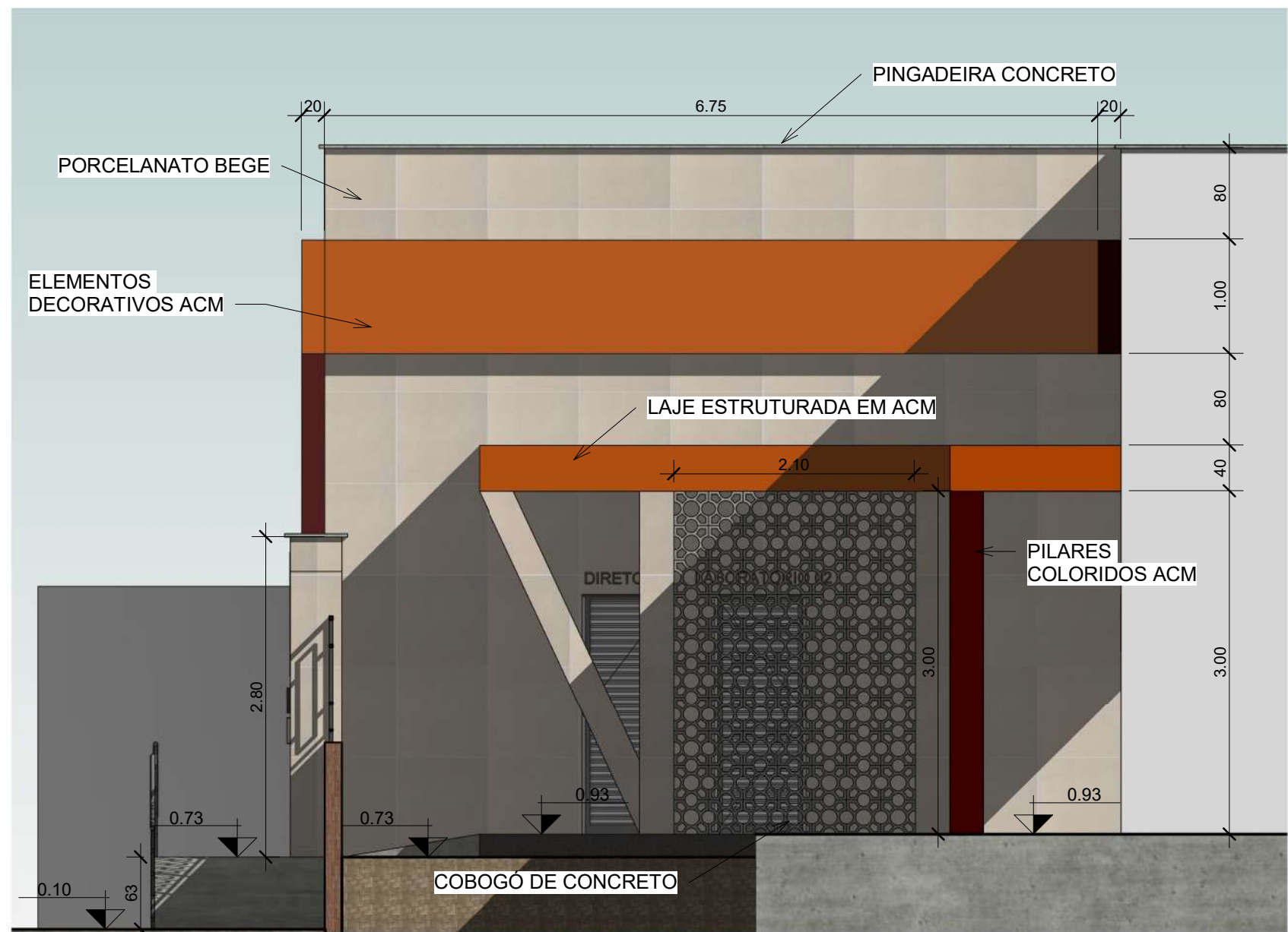
1 VISTA LATERAL FACHADA 1 : 50
