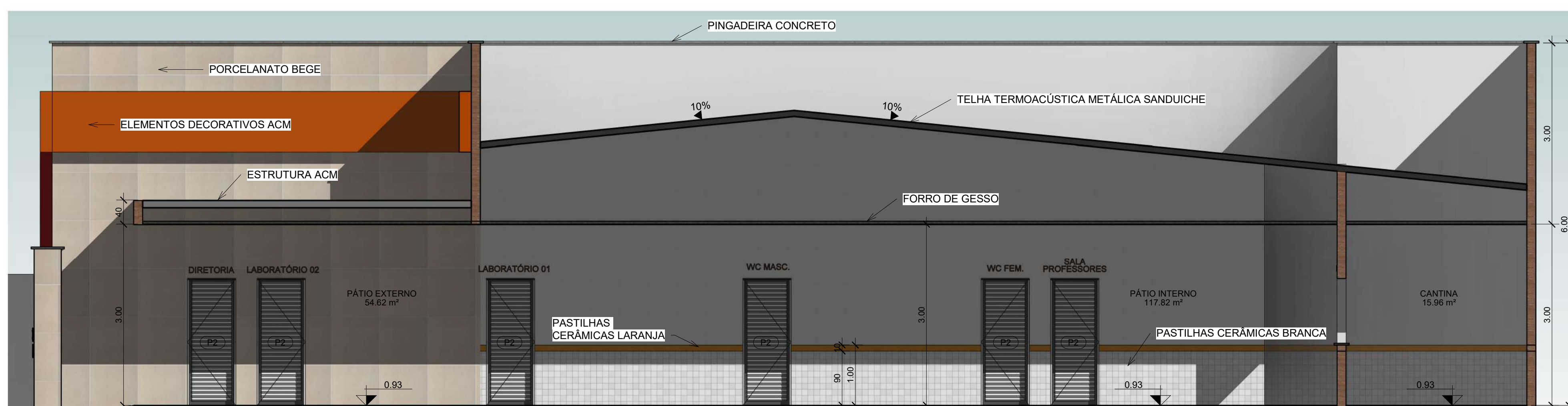
2 CORTE B-B 1 : 50
