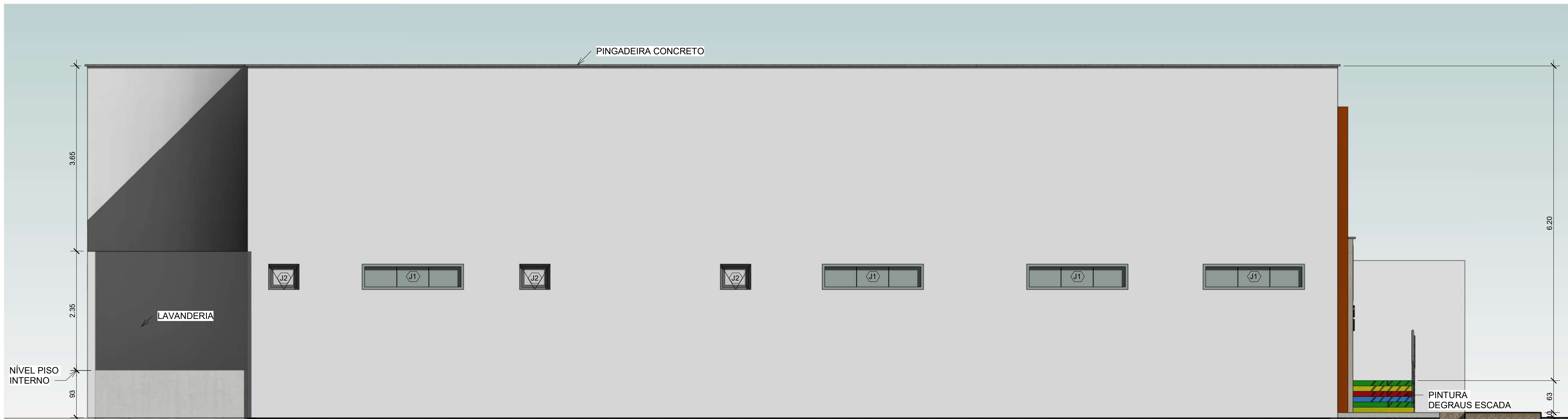
4 LATERAL ESQUERDA 1 : 50
