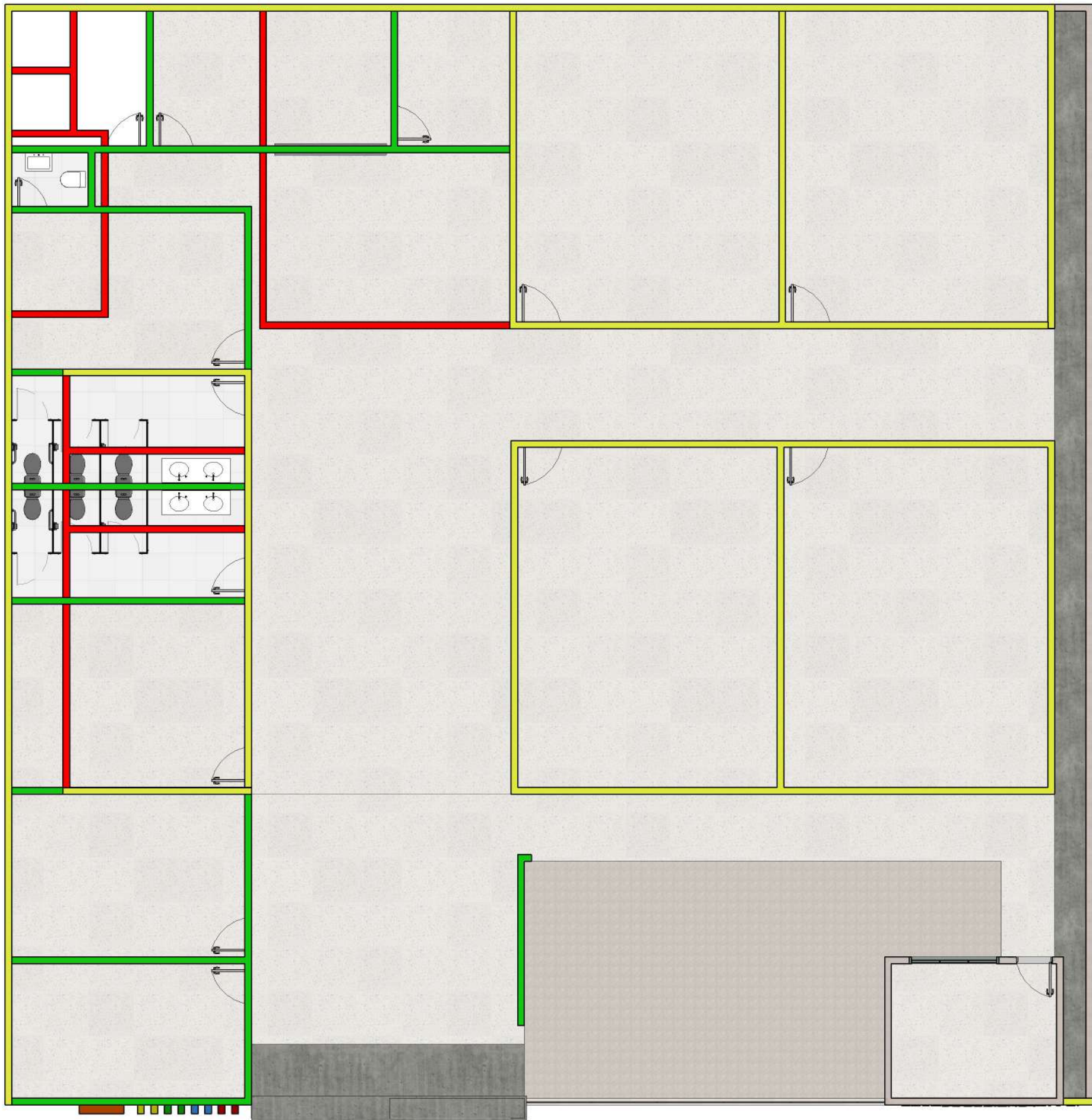
2 PLANTA CONSTRUÇÃO E DEMOLIÇÃO 1 : 100
