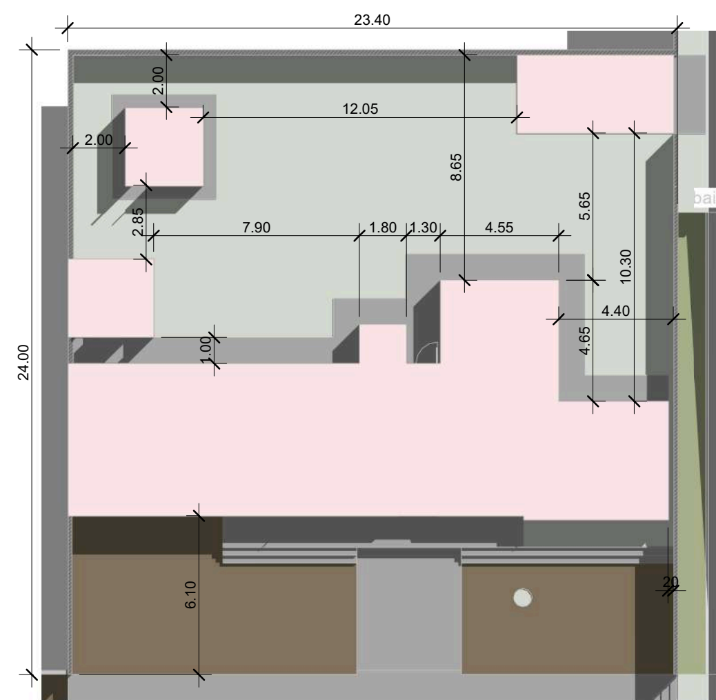
11 PLANTA DE LOCAÇÃO 1 : 200
