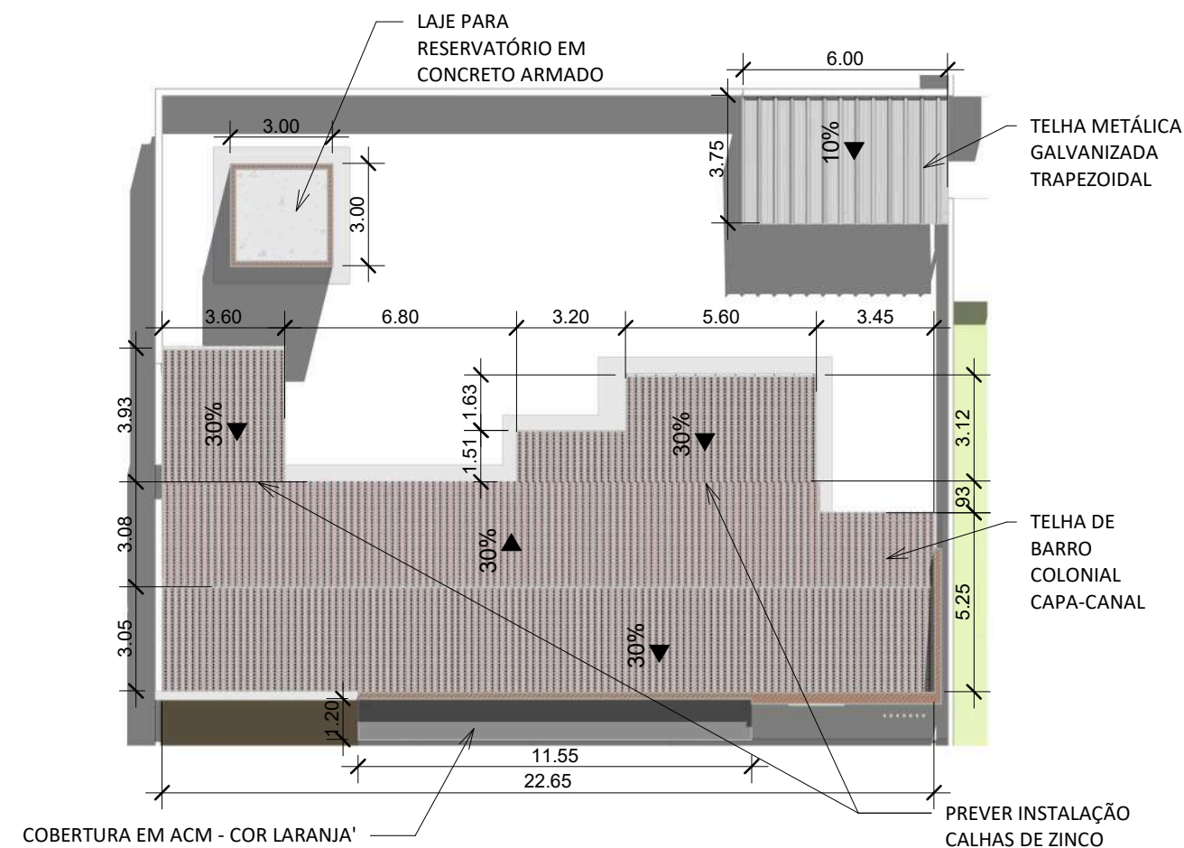
2 PLANTA DE COBERTURA 1 : 200
