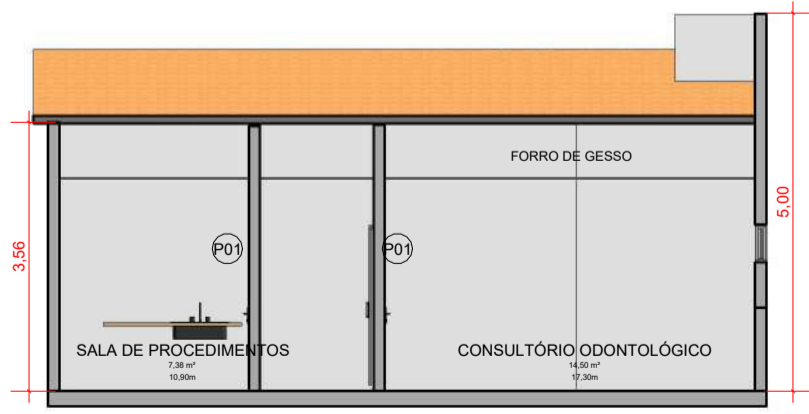
4 CORTE B Escala: 1 : 100
