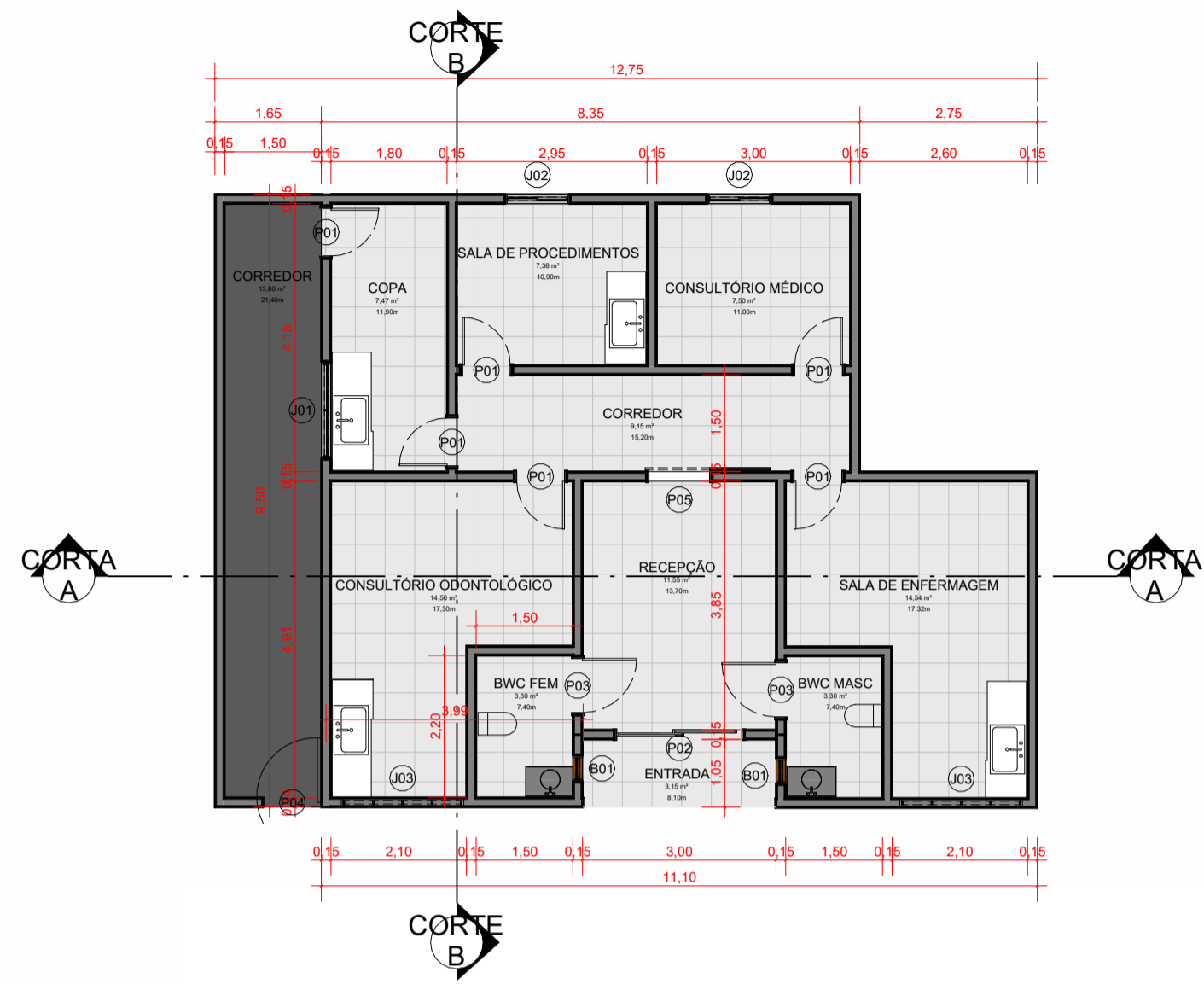
1 PLANTA BAIXA Escala: 1 : 100
