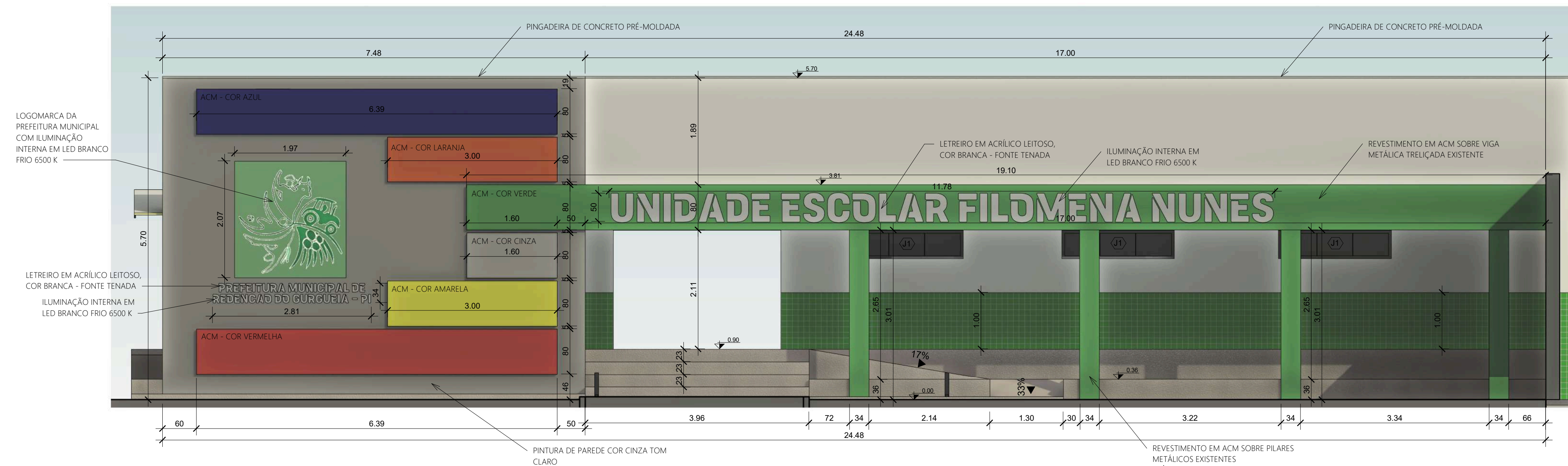
1 FACHADA 1 : 50
