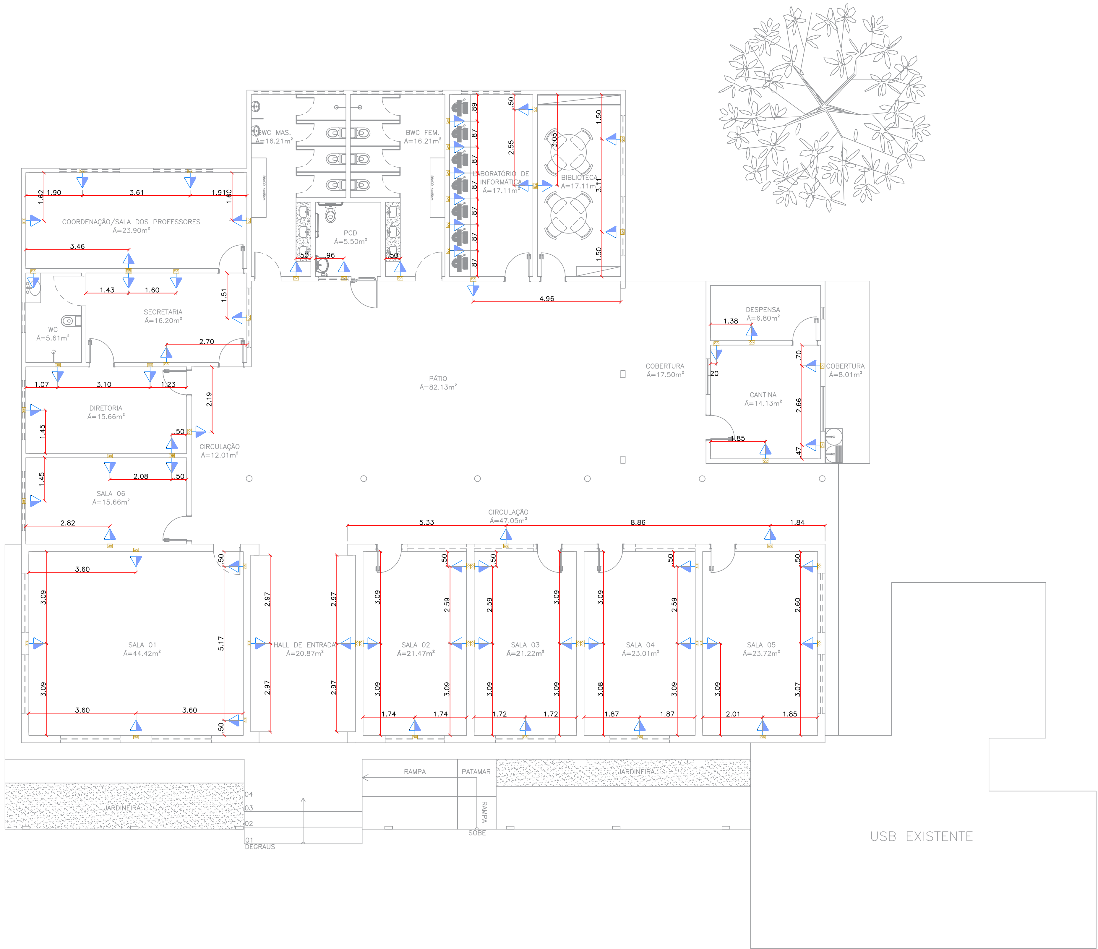
PLANTA DE PONTOS ELÉTRICOS esc 1:75
