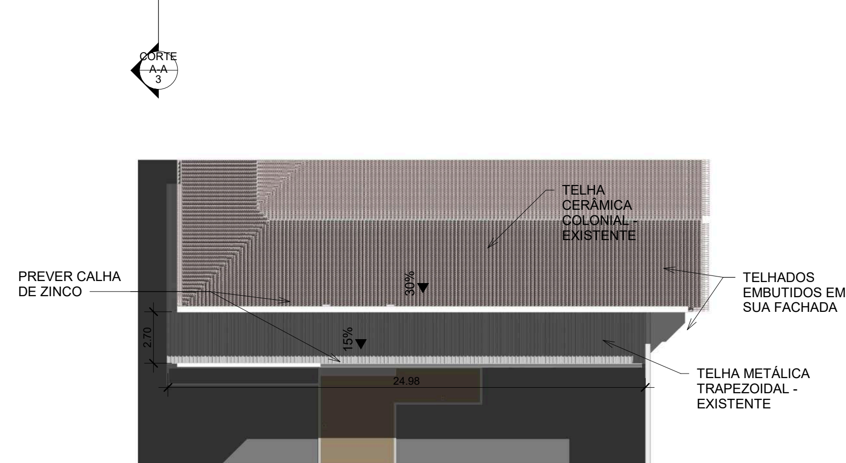
5 PLANTA DE COBERTURA 1 : 200
