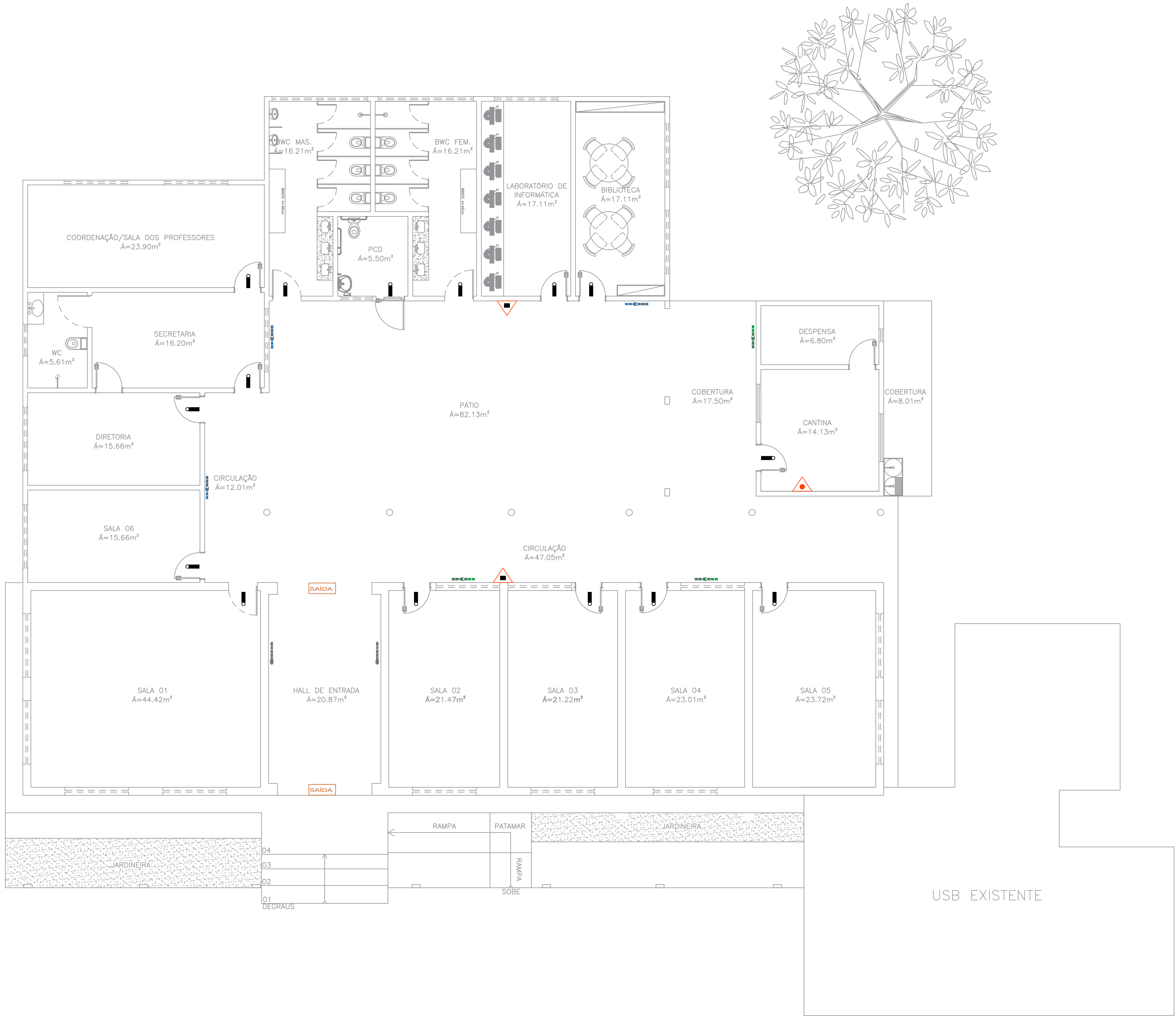
COMBATE A INCÊNDIO esc 1:75
