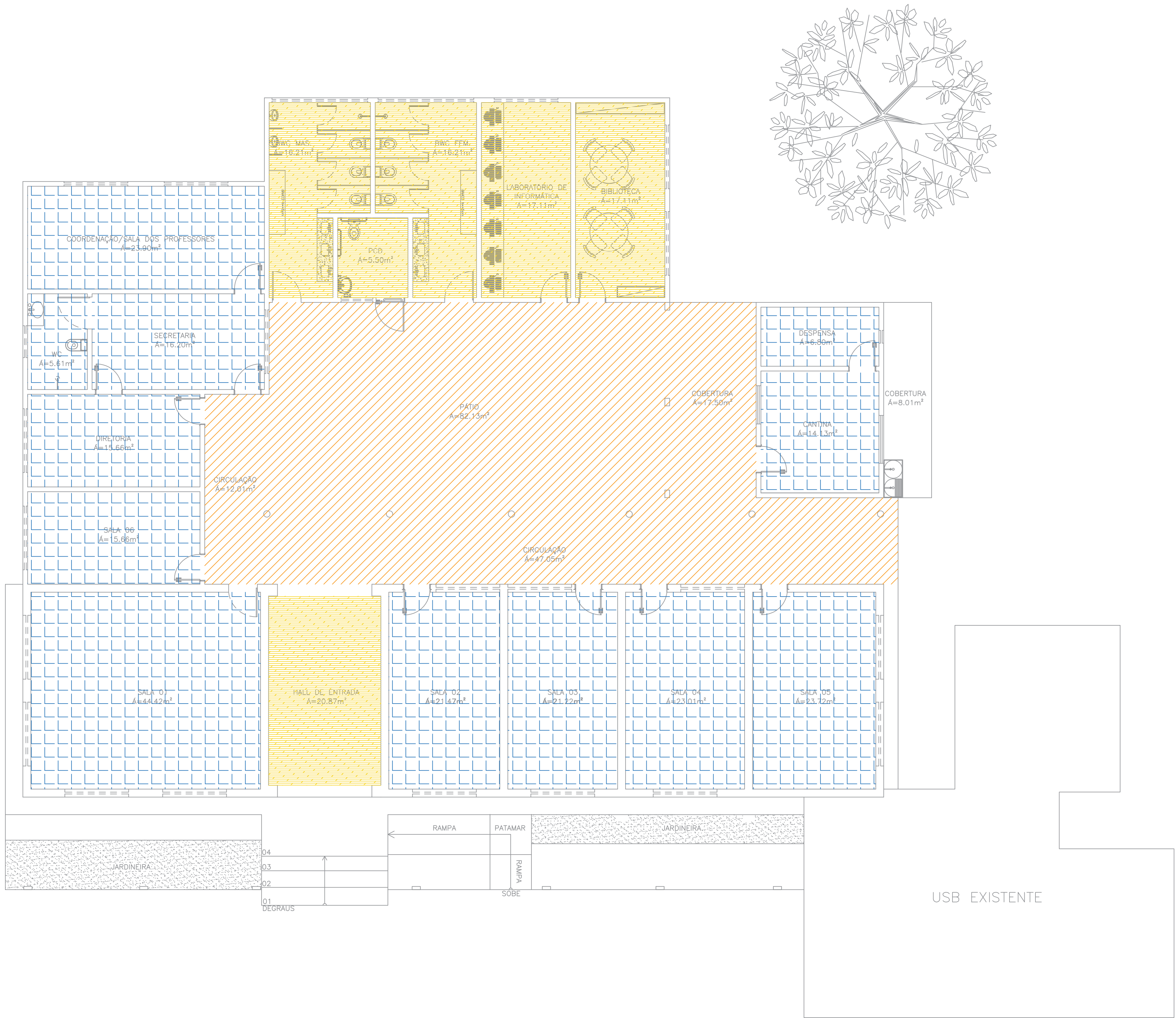
PLANTA DE FORRO esc 1:75
