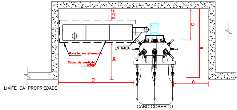
RECUO – Desenho 2; NT.00002.EQTL-10
