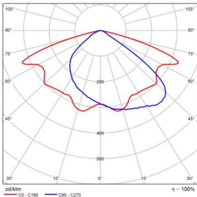
Figura 1 CDL LUMINÁRIA LED 23000LM
