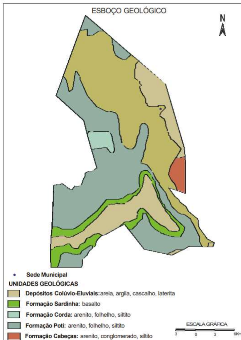
Figura 02 - Esboço Geológico do município
