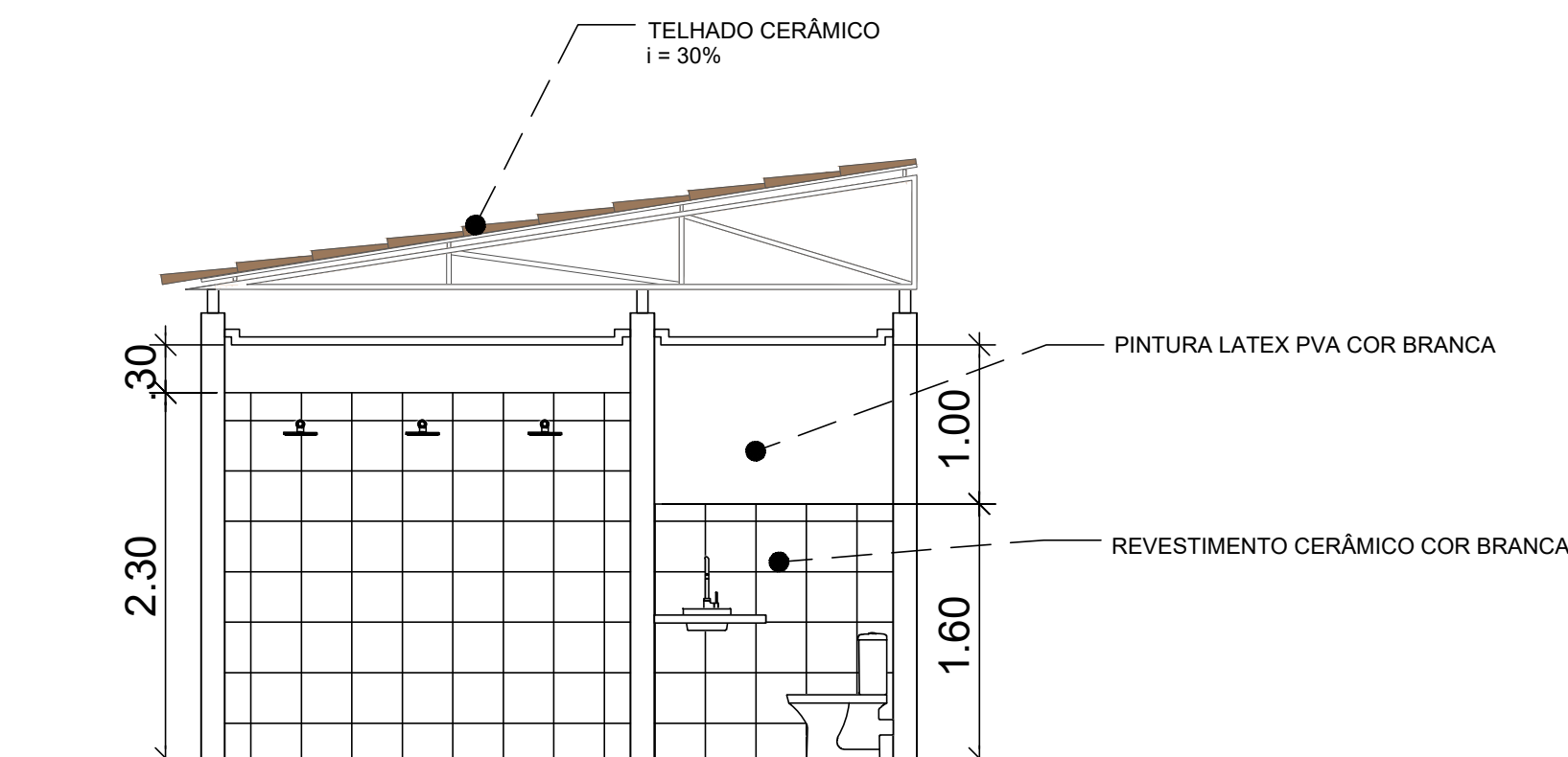
1 VESTIÁRIOS: CORTE AA ESCALA 1:50
