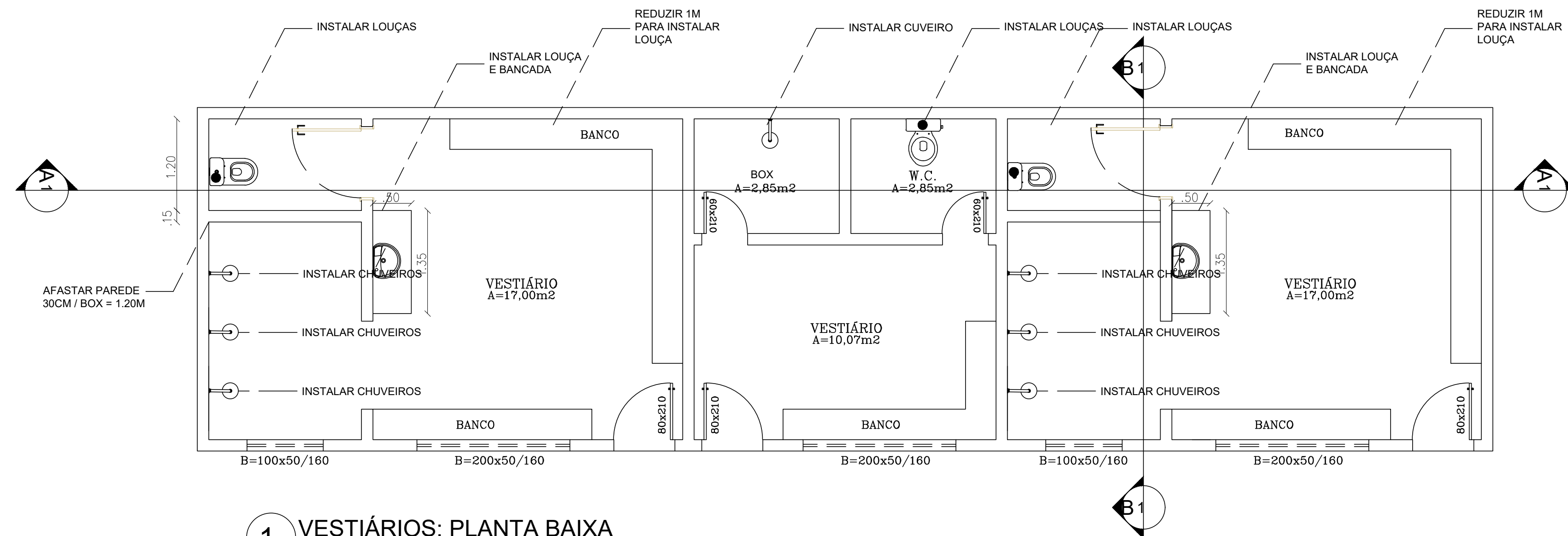
1 VESTIÁRIOS: PLANTA BAIXA ESCALA 1:50
