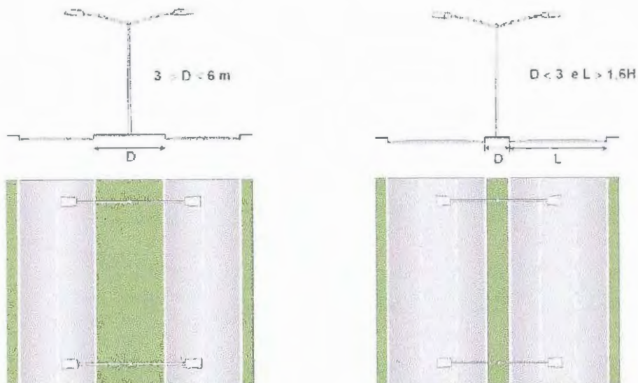
Posteação central com poste chicote
