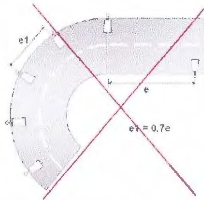
Posteação no lado externo da curva
