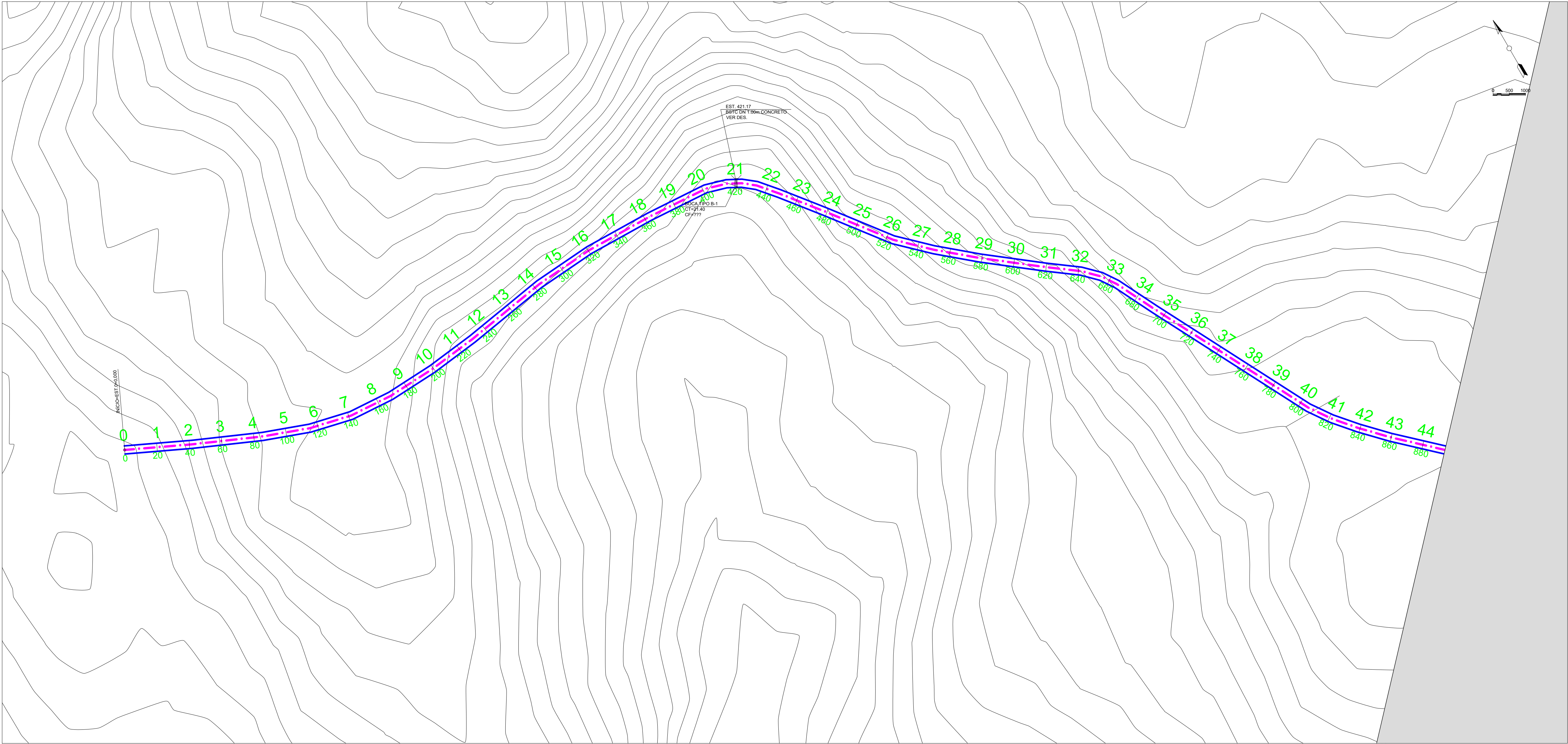
PLANTA DE ESTAQUEAMENTO - TRECHO 1 (PARTE 1)
