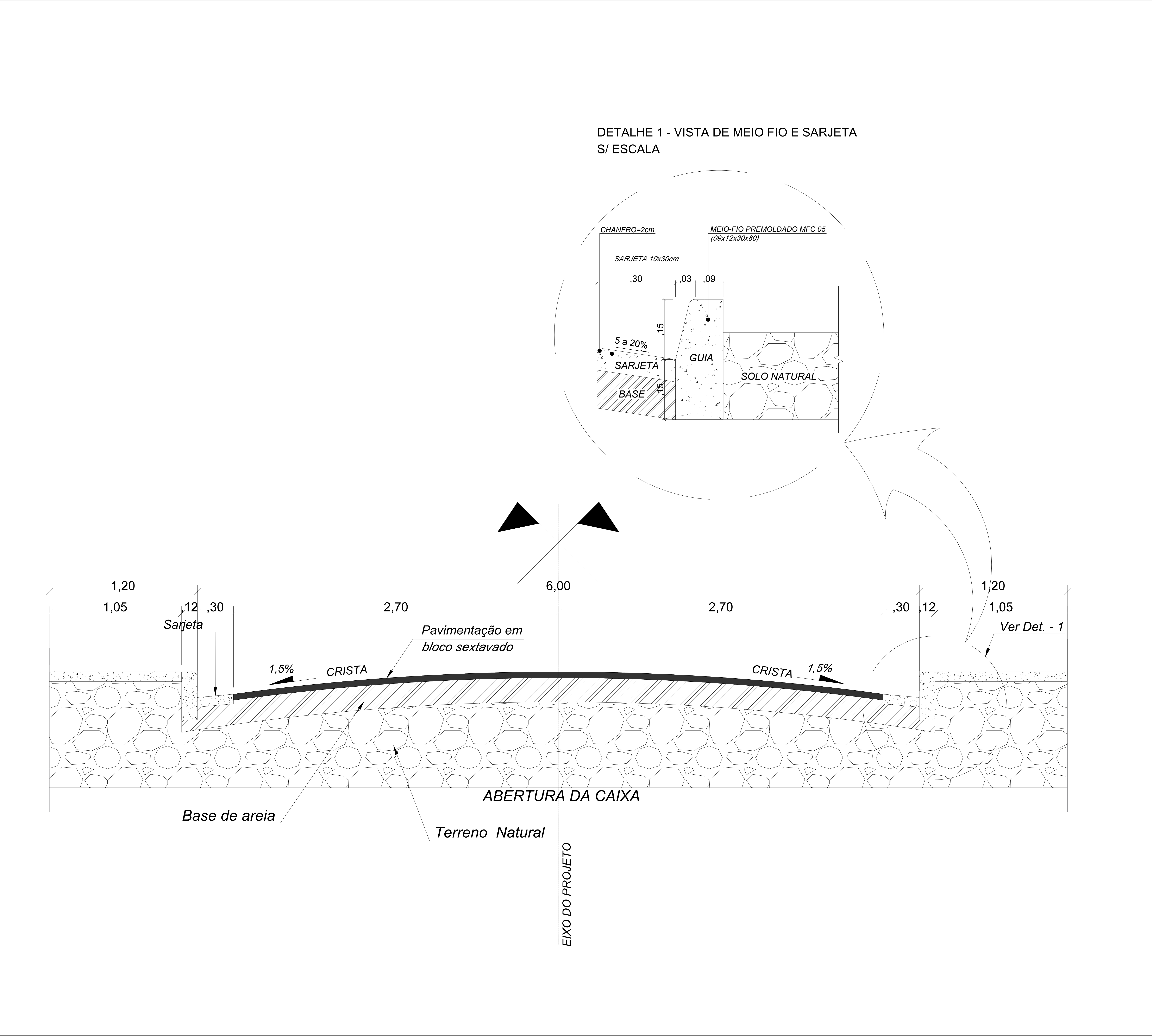
DETALHE – SECÇÃO TRANSVERSAL MEIO FIO, SARJETA E CALÇADA S/ESC.
