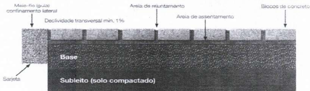
Figura 2: Estrutura típica dos pavimentos intertravados.
