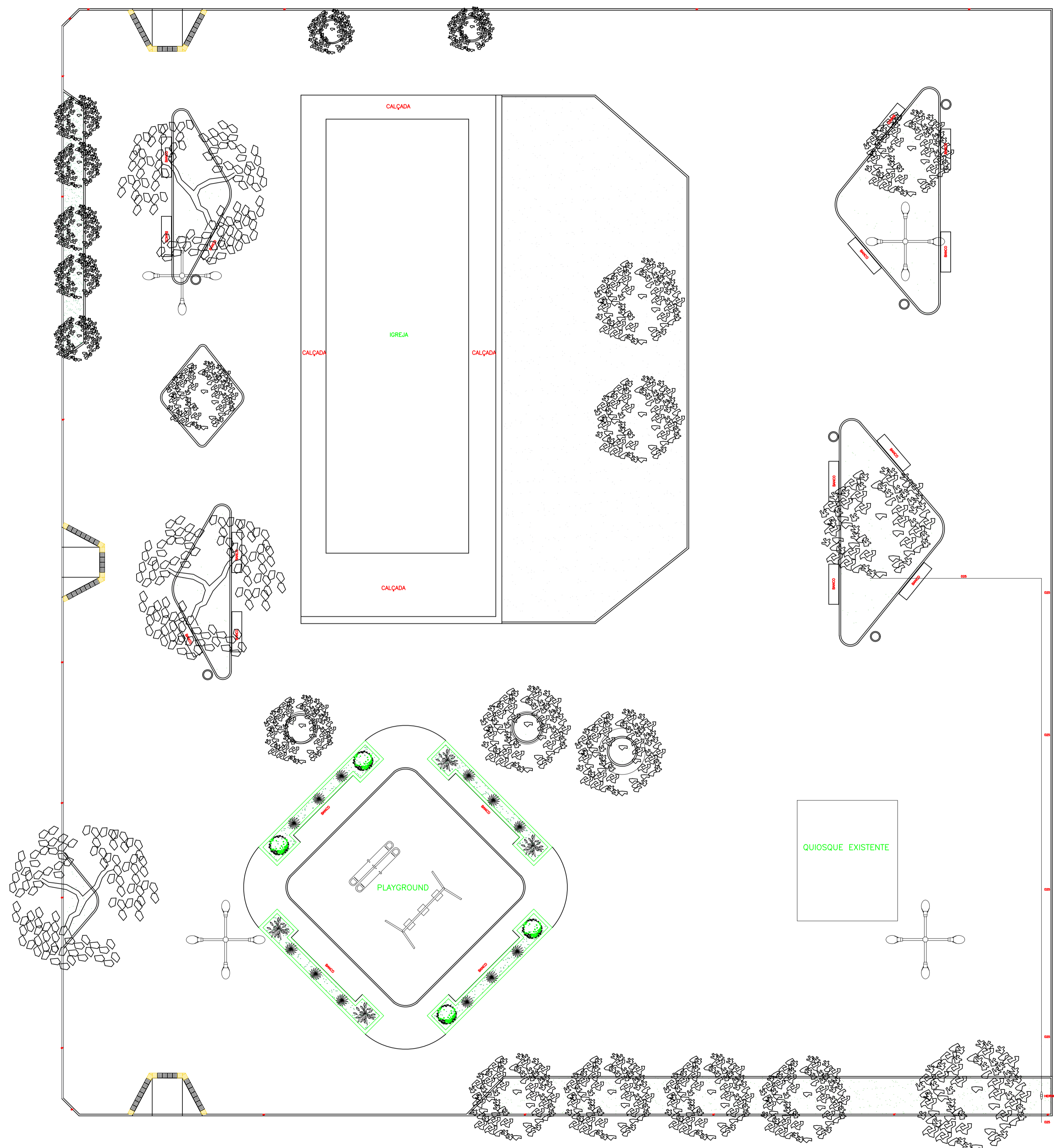
01 PLANTA PROJETO HIDRAULICO esc: 1:125
