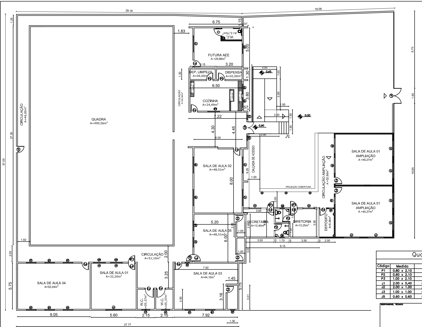
1 PLANTA BAIXA Escala: S/E
