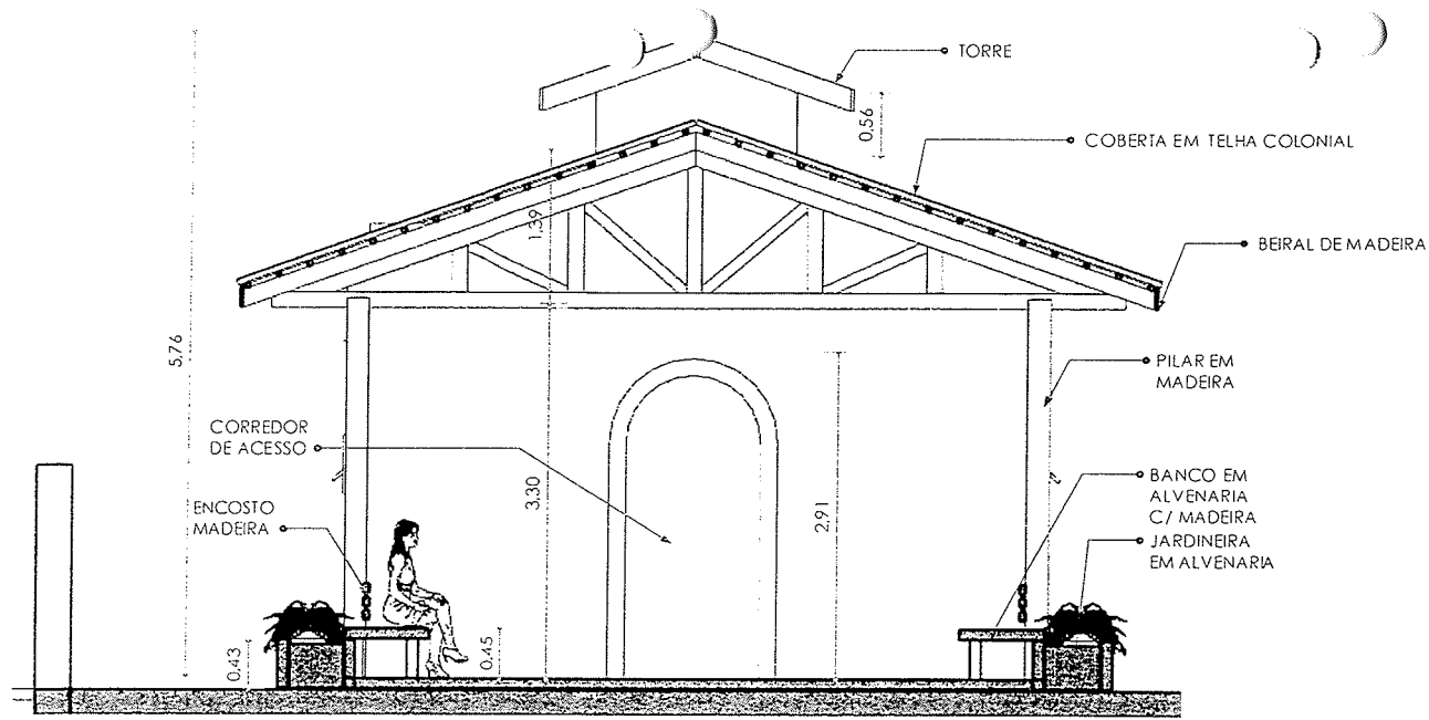
01 CORTE A Escala 1:50
