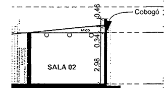
Corte BB Escala: 1:150
