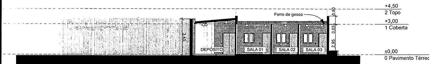
Corte AA Escala: 1:150
