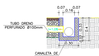
04 DETALHE CANALETA DE CONCRETO 5/ESC.
