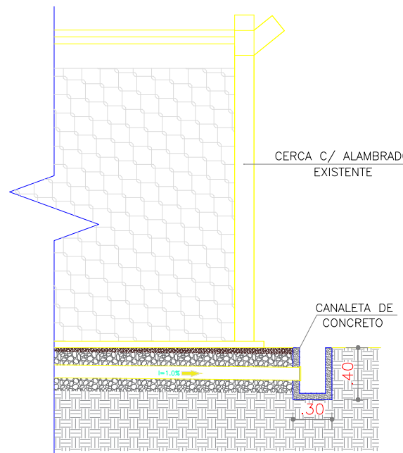
02 CORTE AA 5/ESC.
