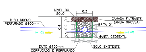
03 DETALHE SISTEMA DE DRENAGEM 5/ESC.
