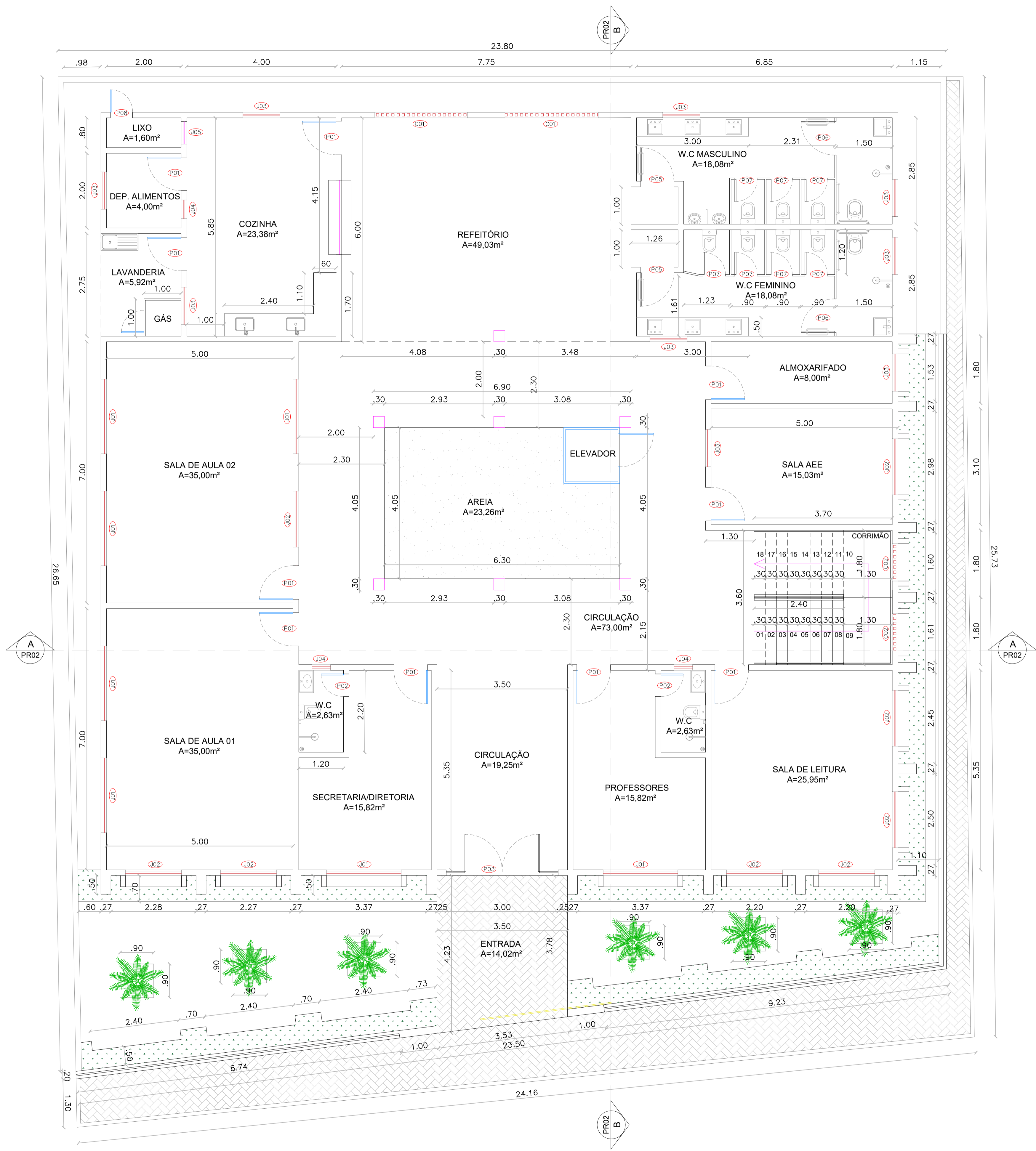
01 PAV. TÉRREO Escala 1:50
