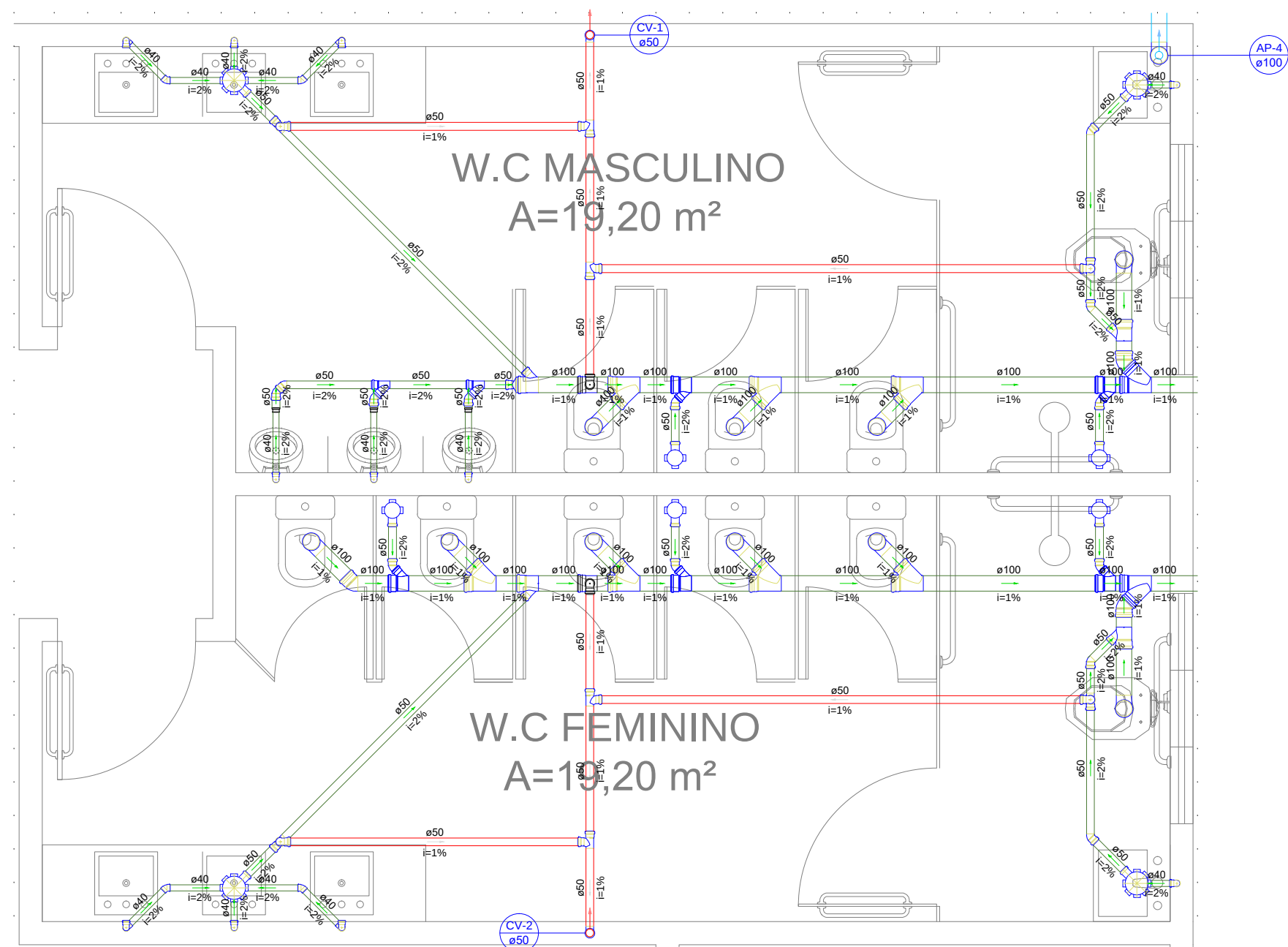
Detalhe SAN-2 Escala 1:25
