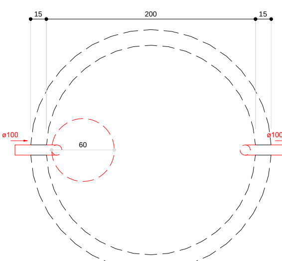
Tanque séptico - TERREO Planta baixa - ESC. 1:25
