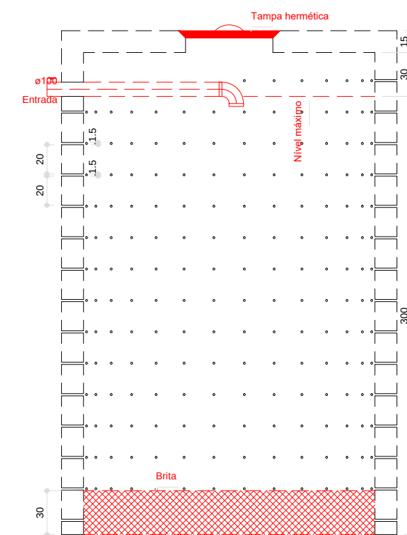
Sumidouro - TERREO Corte 1 - ESC. 1:25
