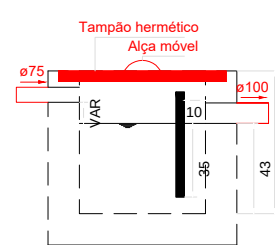
Caixa de gordura - TERREO Corte 1 - ESC. 1:25
