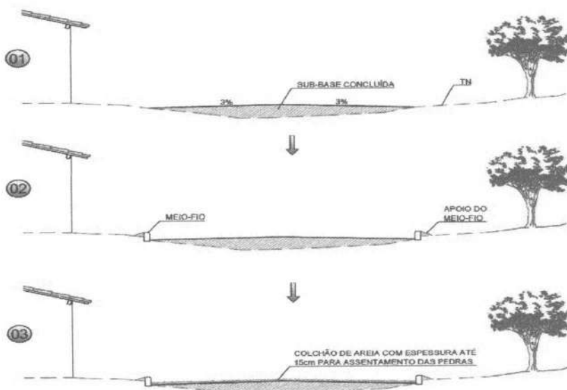
MÉTODO CONSTRUTIVO DE PAVIMENTO EM PEDRA TOSCA SEGUNDO A ESPECIFICAÇÃO DER-ES-P 18/94
