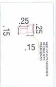
14 DETALHE 7 - MEIO FIO ESCALA 1:200
