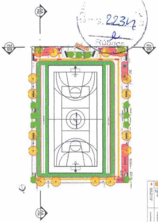
7 LUMINOTÉCNICO ESCALA 1:100
