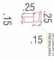
10 DETALHE 6 - MEIO FIO ESCALA 1:20
