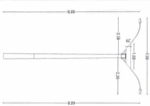
8 DETALHE 3 - POSTE E CRUZEIRO ESCALA 1:20
