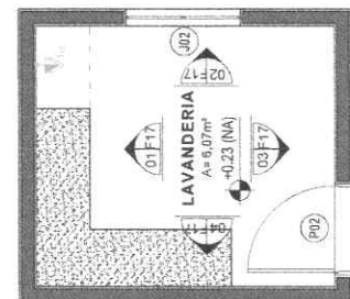
1 VISTA 1 ESCALA: 1/25
