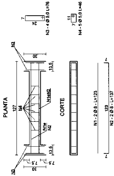
NERVURAS (Esc. 1:20)
