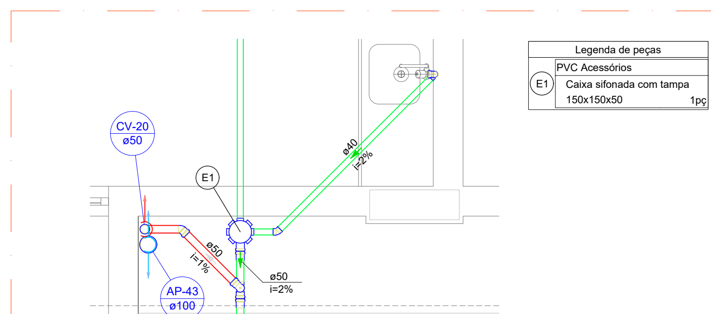
12 DETALHE S12 ESCALA 1/25
