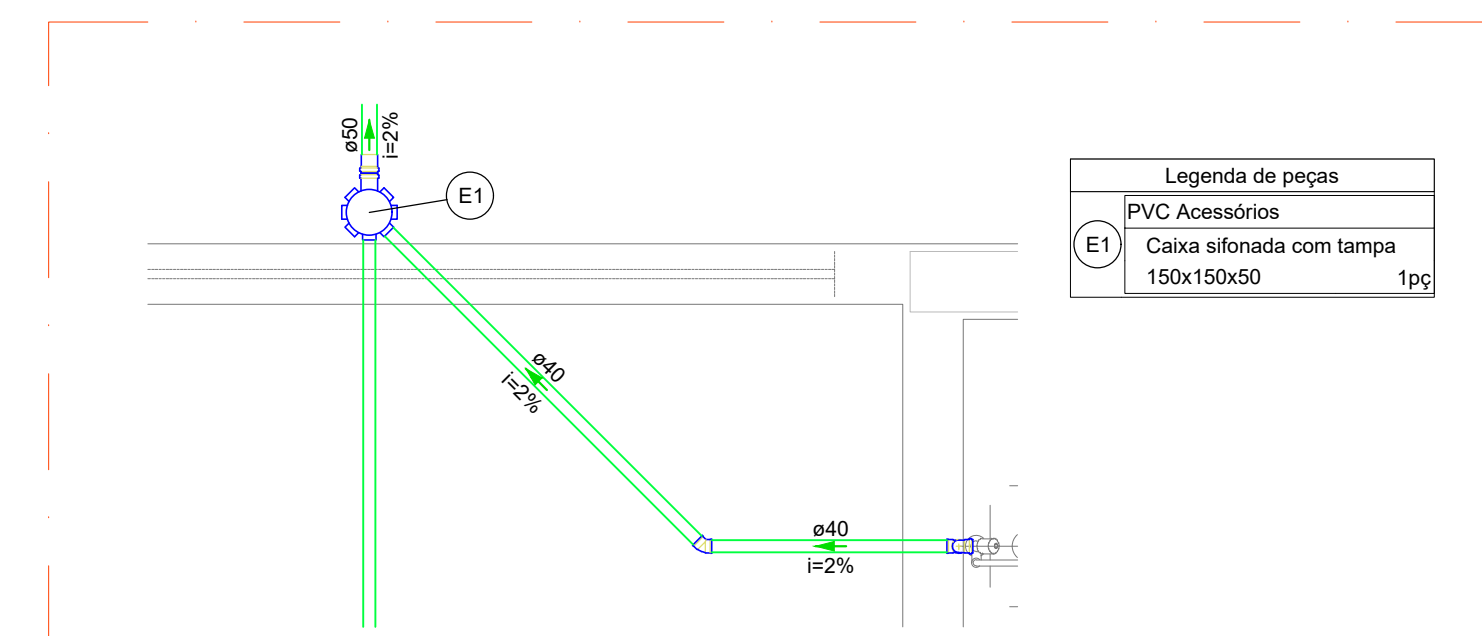
16 DETALHE S16 ESCALA 1/25
