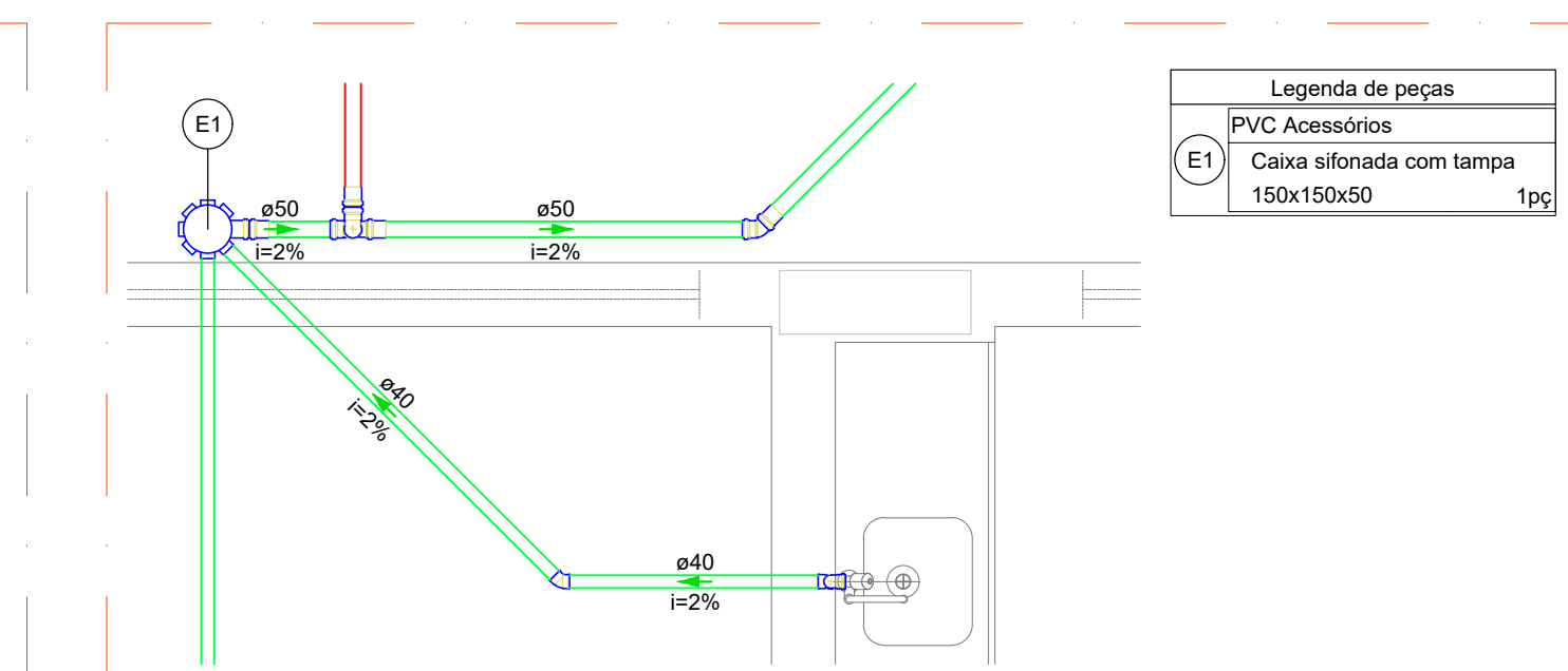
15 DETALHE S15 ESCALA 1/25
