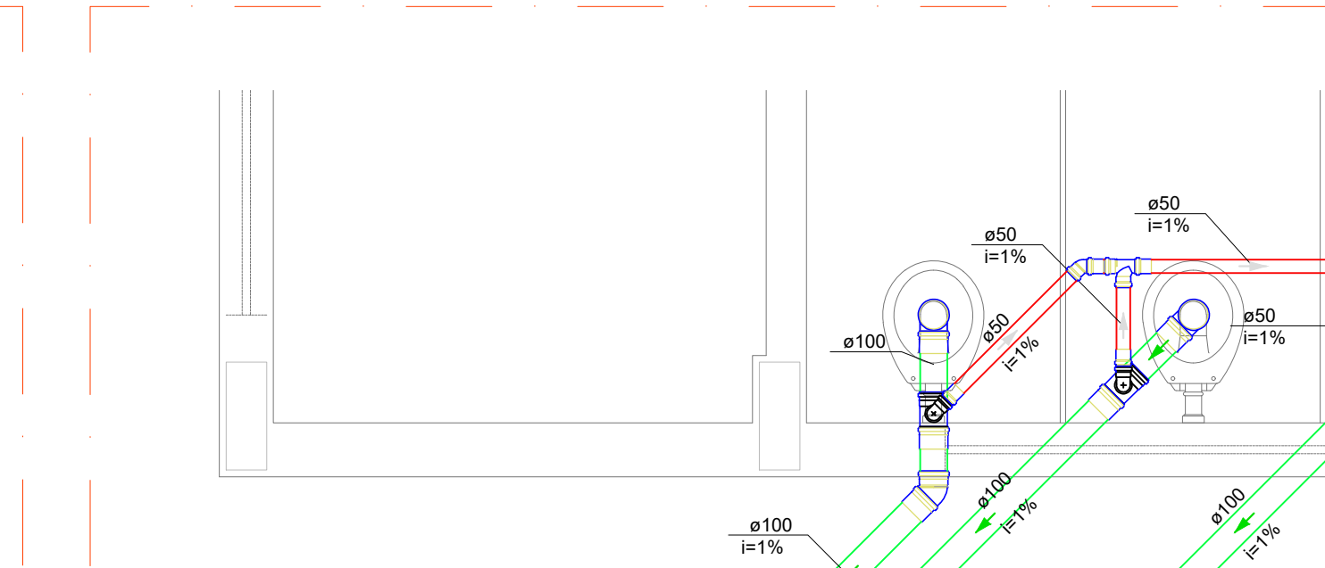
19 DETALHE S19 ESCALA 1/25
