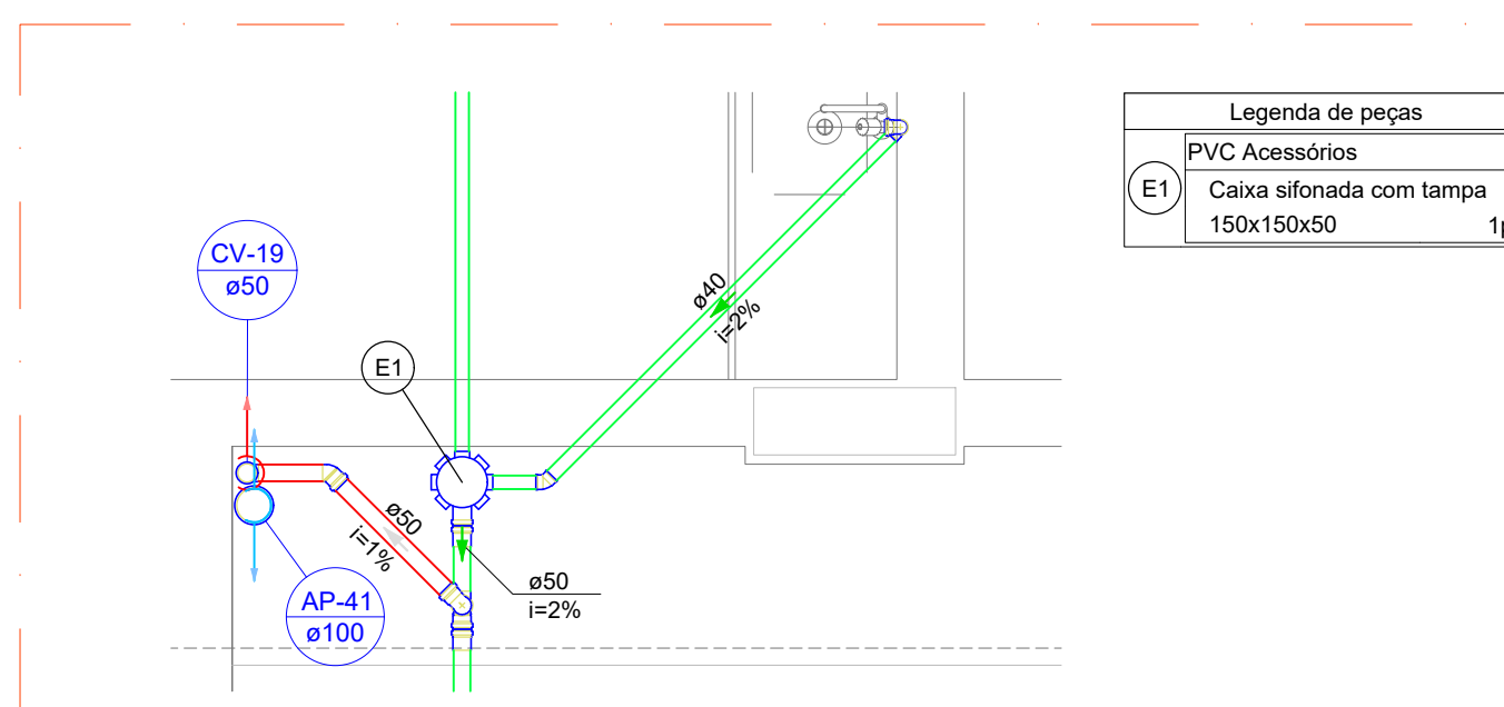
13 DETALHE S13 ESCALA 1/25
