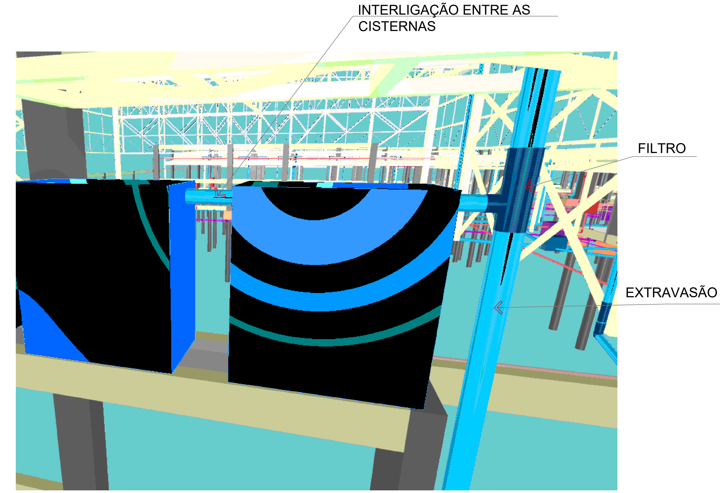
21 INTERLIGAÇÃO DAS CISTERNAS SEM ESCALA
