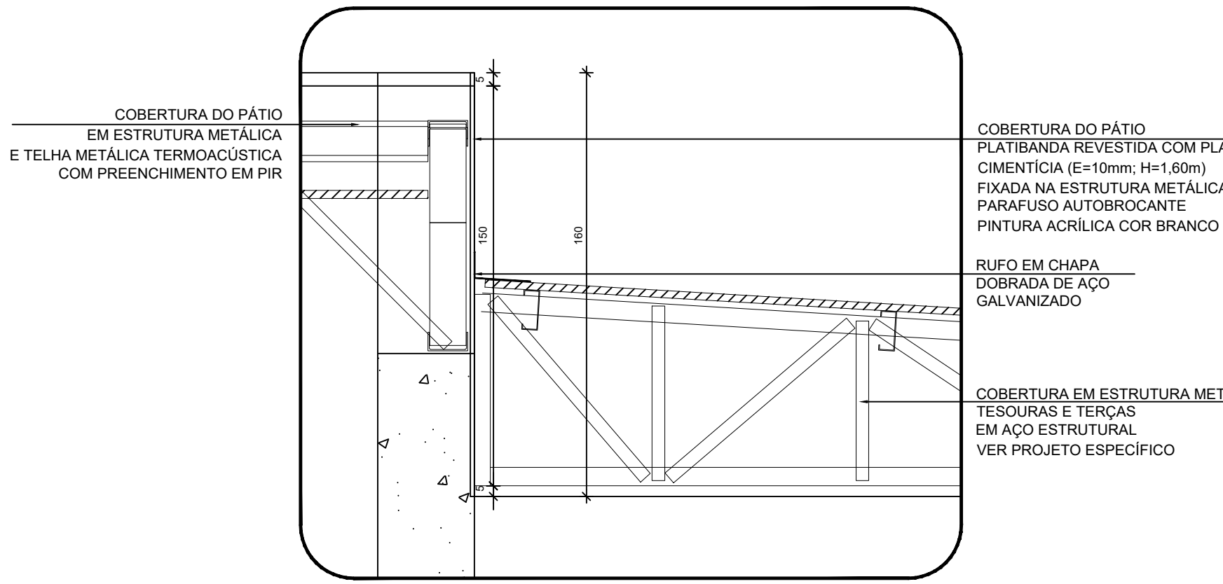
7 DETALHE 3 - PÁTIO COBERTO ESCALA 1/25
