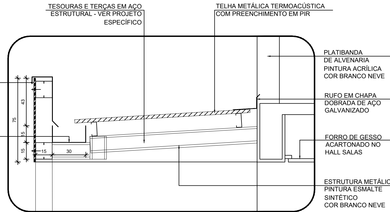
6 DETALHE 2 - PASSARELAS ESCALA 1/20
