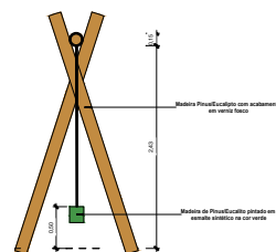
⑥ Corte 5 1 : 25
