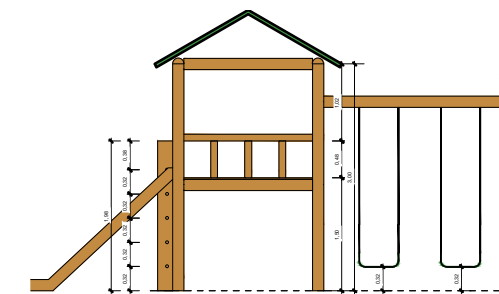
③ Vista 2 1 : 25
