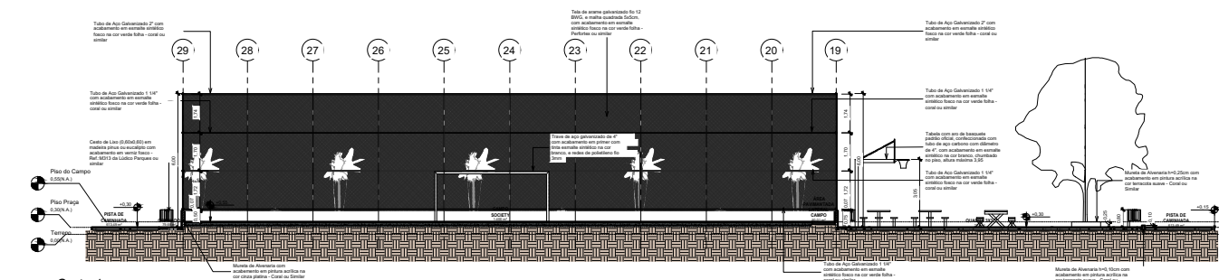
1 Corte 1 1:75
