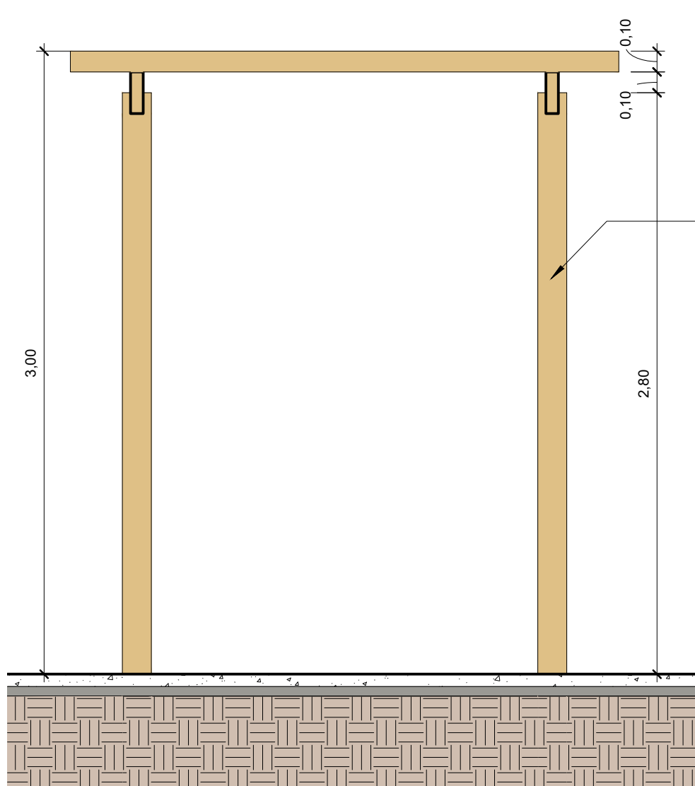
4 Corte 4 1 : 25
