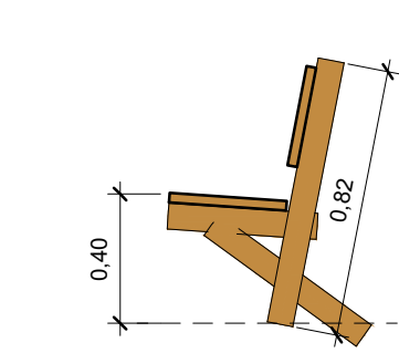
7 Corte 7 1 : 25
