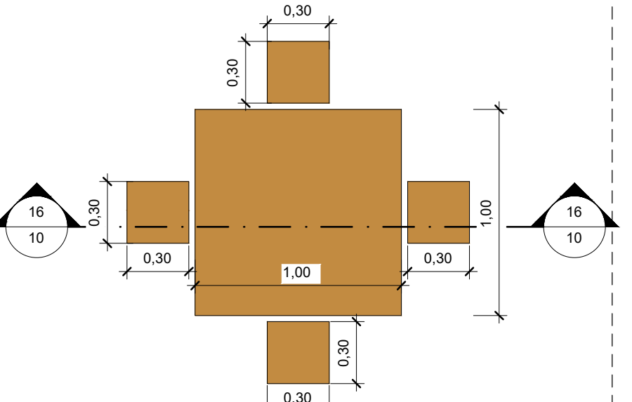
17 Planta Baixa 1 : 25
