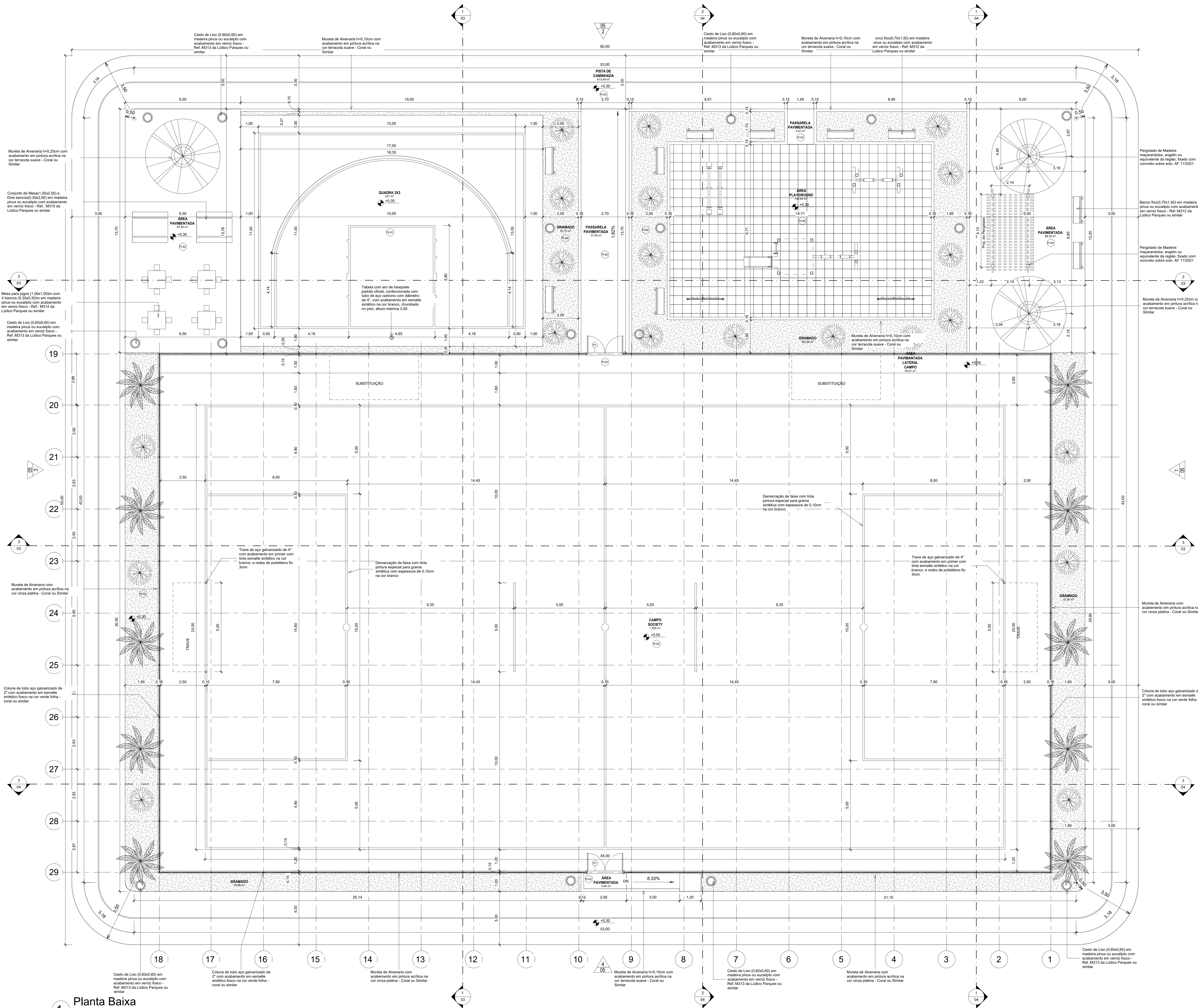
1 Planta Baixa 1 : 75
