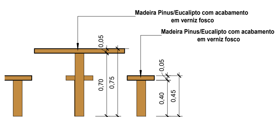
16 Corte 16 1 : 25
