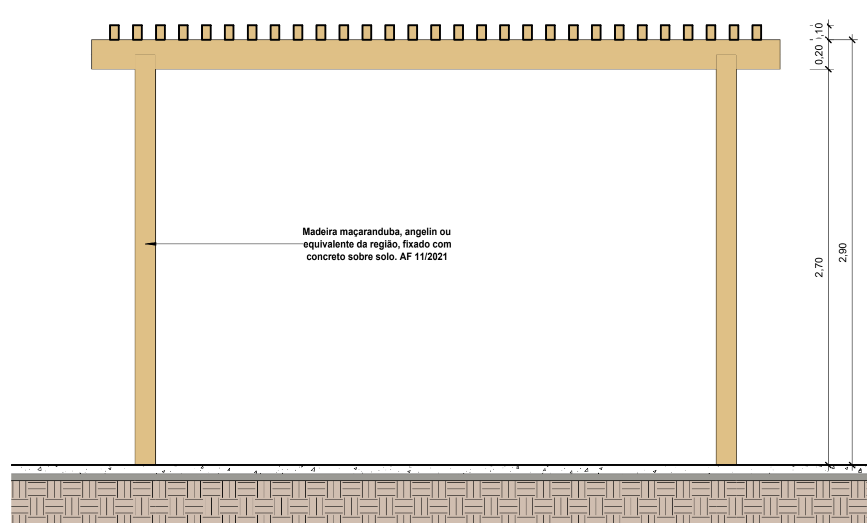
5 Corte 5 1 : 25
