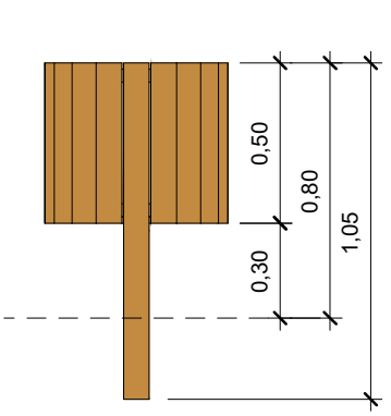
10 Vista 10 1 : 25
