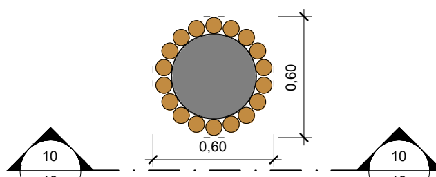
11 Planta Baixa 1 : 25
