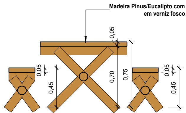
13 Corte 13 1 : 25
