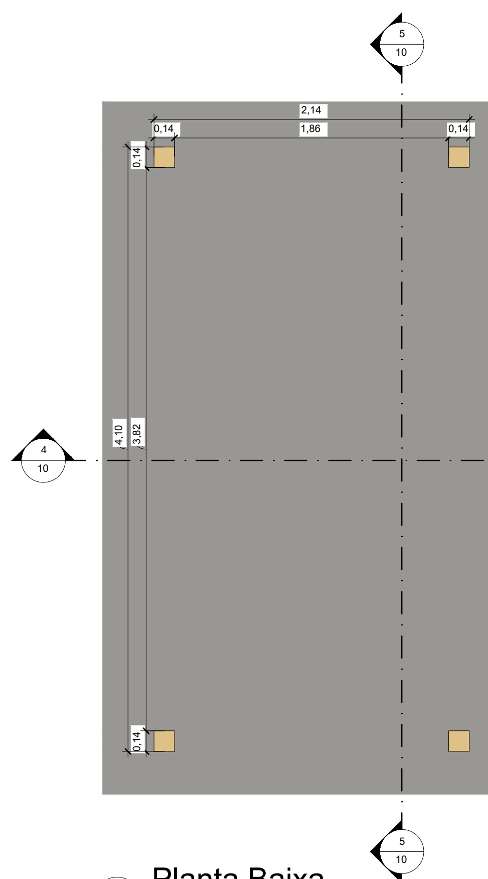
2 Planta Baixa 1 : 25
