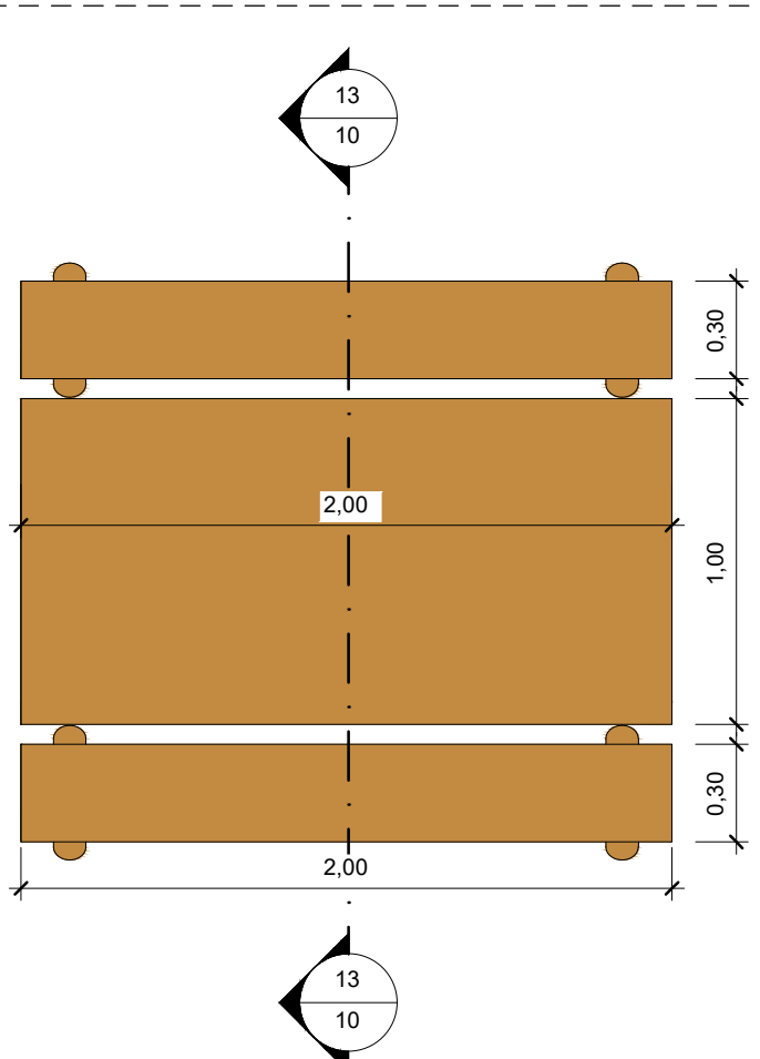
14 Planta Baixa 1 : 25
