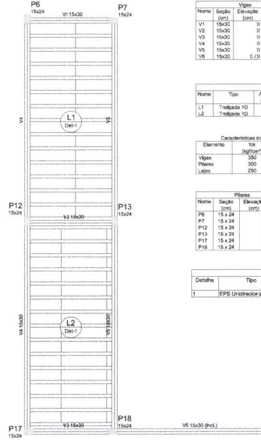
Forma do pavimento Topo do muro de contorno (superior)
