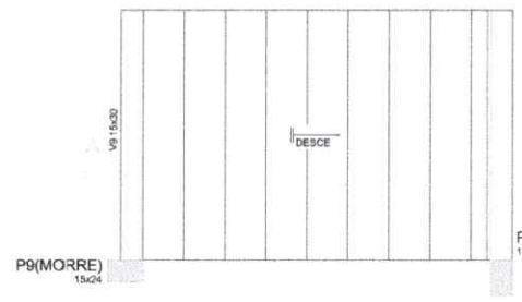
Armação positiva da escada E1
