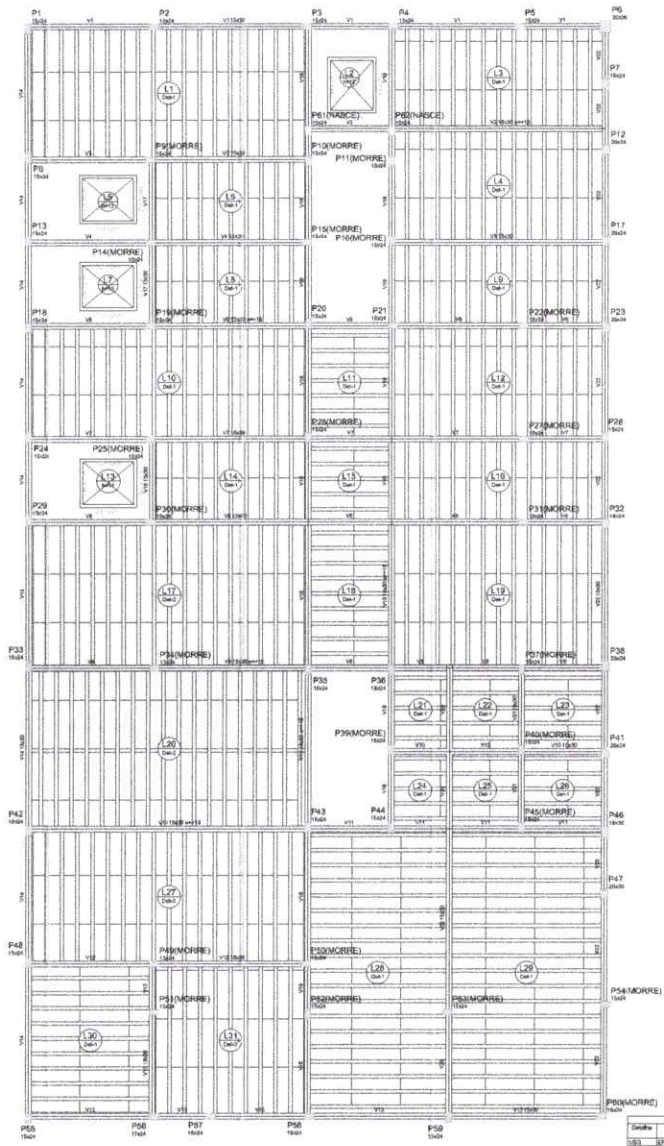
Forma do pavimento COBERTURA escala 1:30
