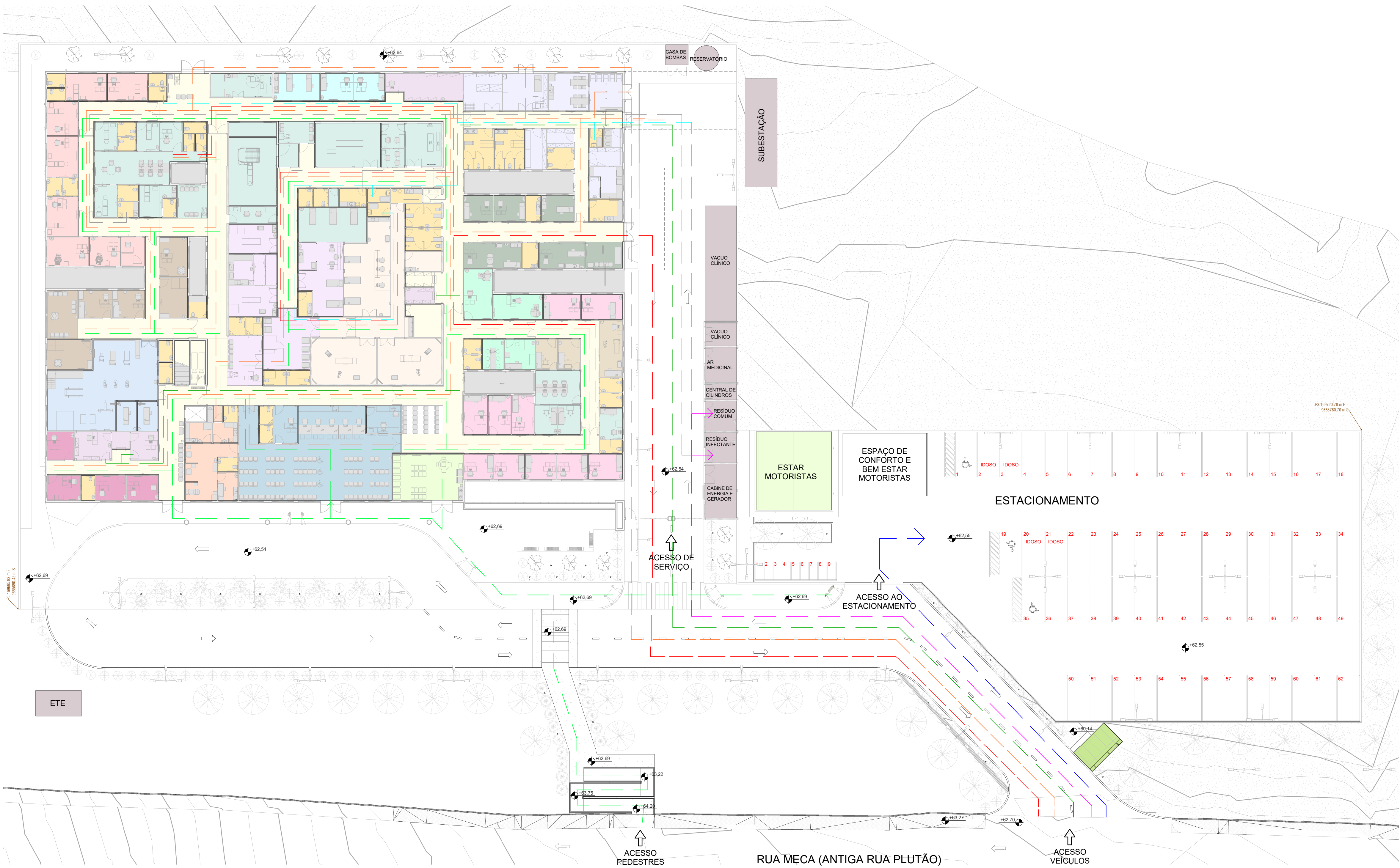
1 IMPLANTAÇÃO - PLANTA DE FLUXOS ESCALA: 1 : 250
