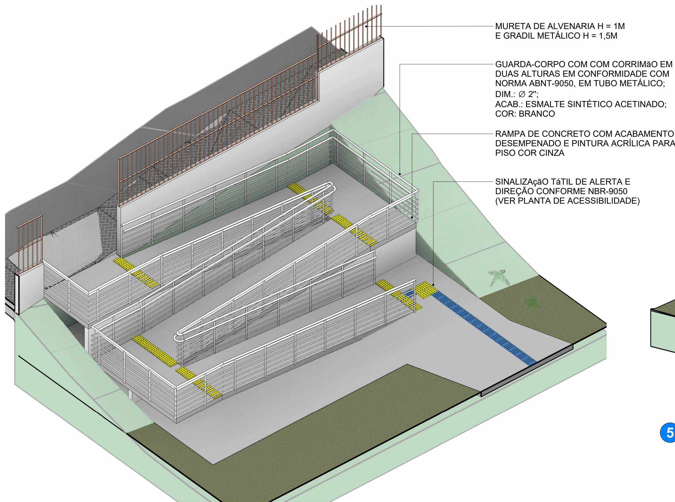
2 PERSPECTIVA - RAMPA DE ACESSO ESCALA:
