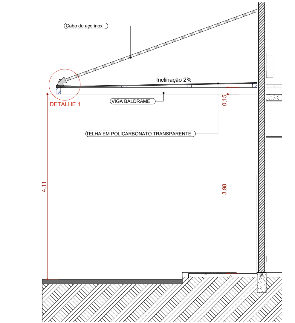
Det 1 1:50
