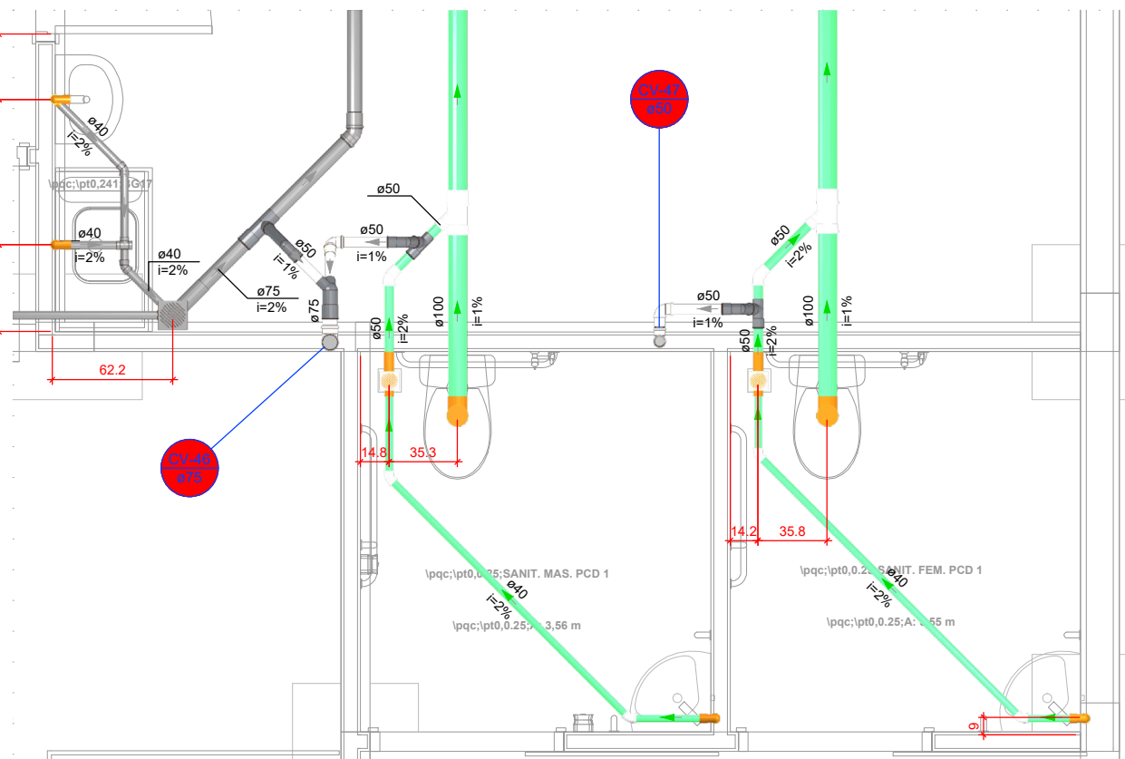
DETALHE SAN-19 1:25
