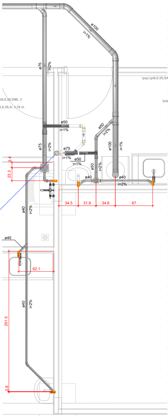
DETALHE SAN-10 1:25
