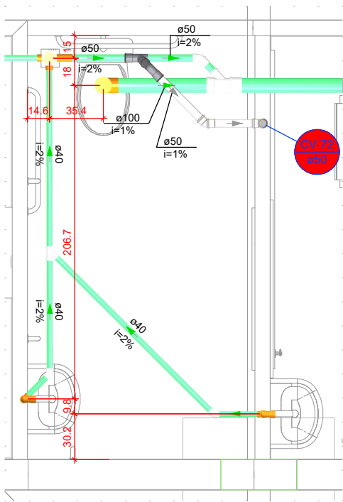
DETALHE SAN-32 1:25
