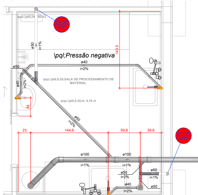
DETALHE SAN-18 1:25
