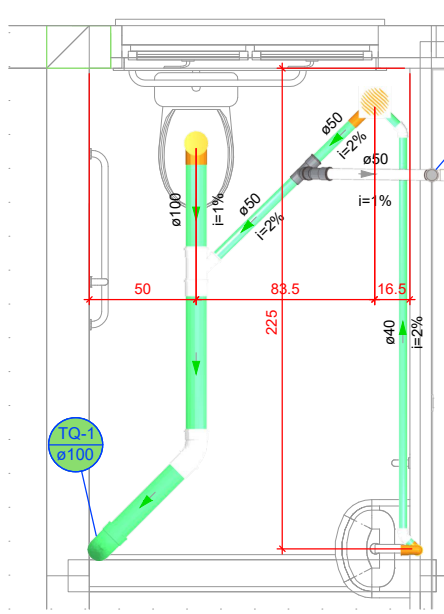
DETALHE SAN-36 1:25
