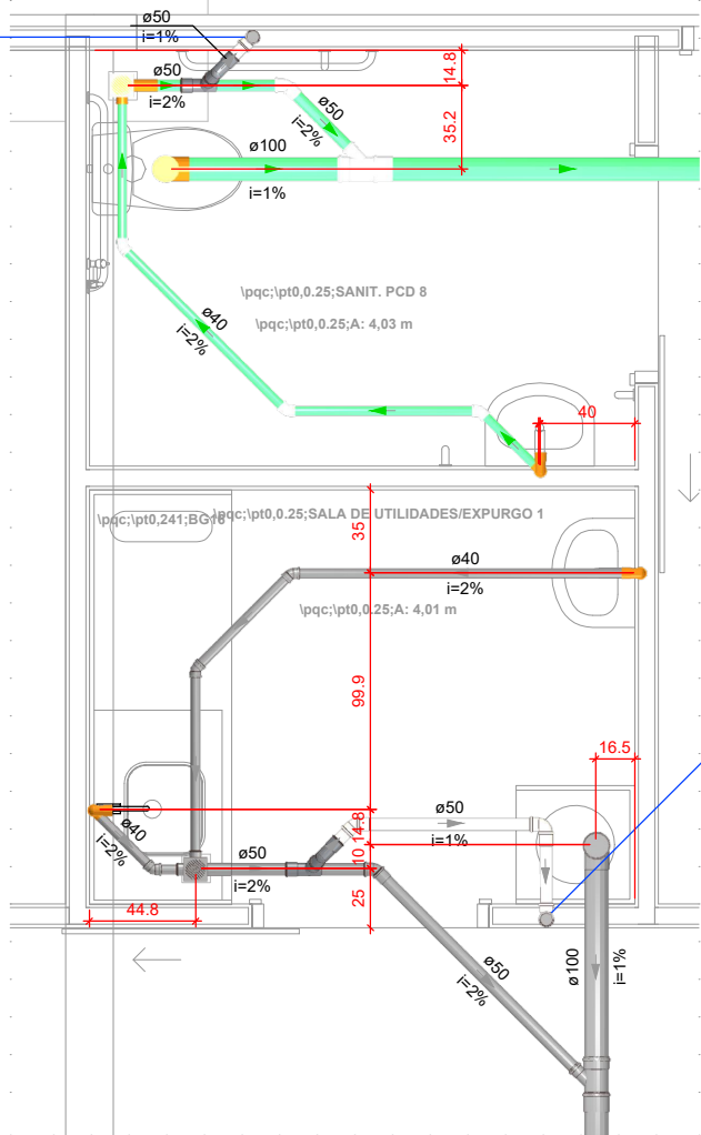
DETALHE SAN-11 1:25
