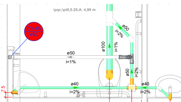
DETALHE SAN-20 1:25
