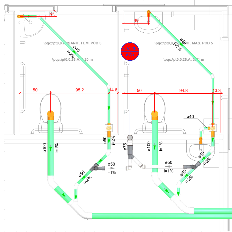
DETALHE SAN-12 1:25
