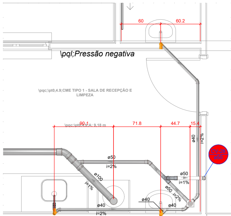
DETALHE SAN-15 1:25
