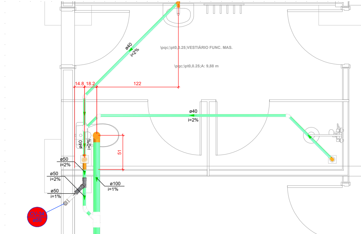
DETALHE SAN-17 1:25
