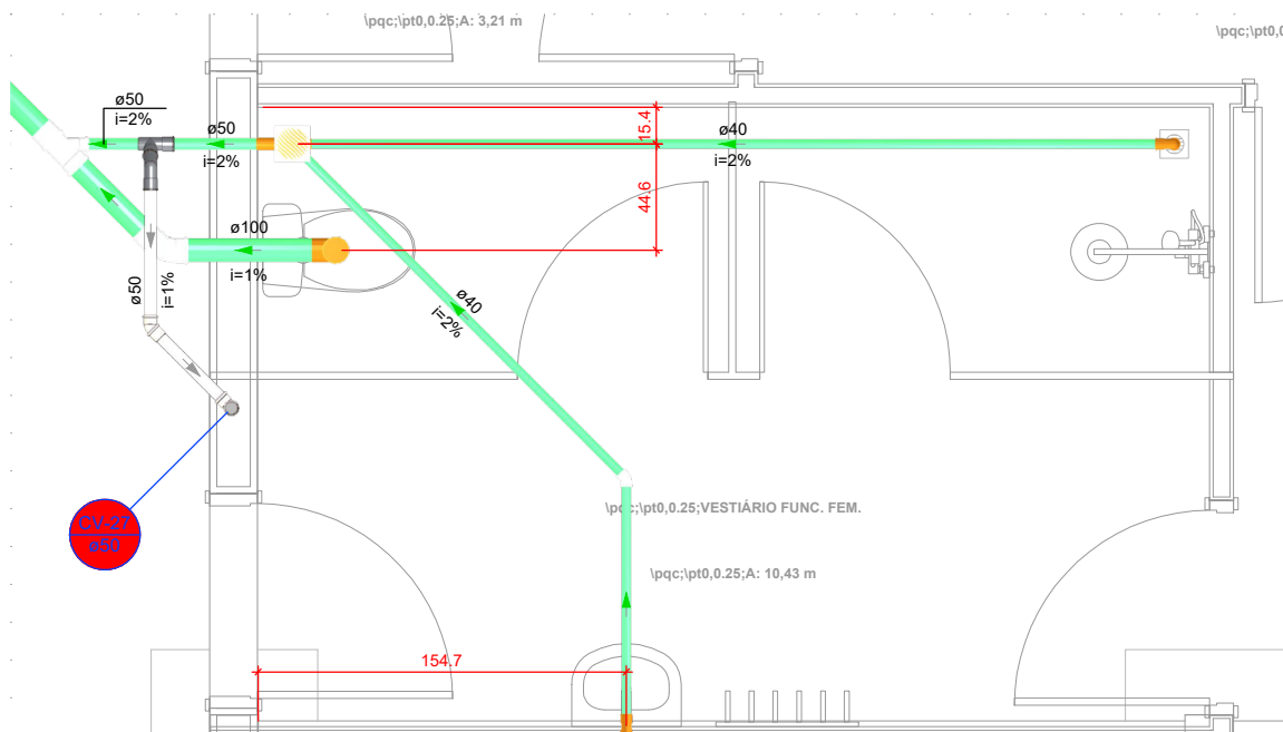
DETALHE SAN-16 1:25
