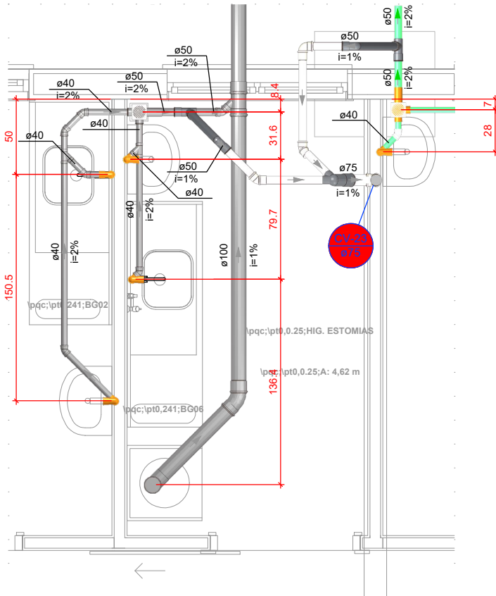
DETALHE SAN-14 1:25
