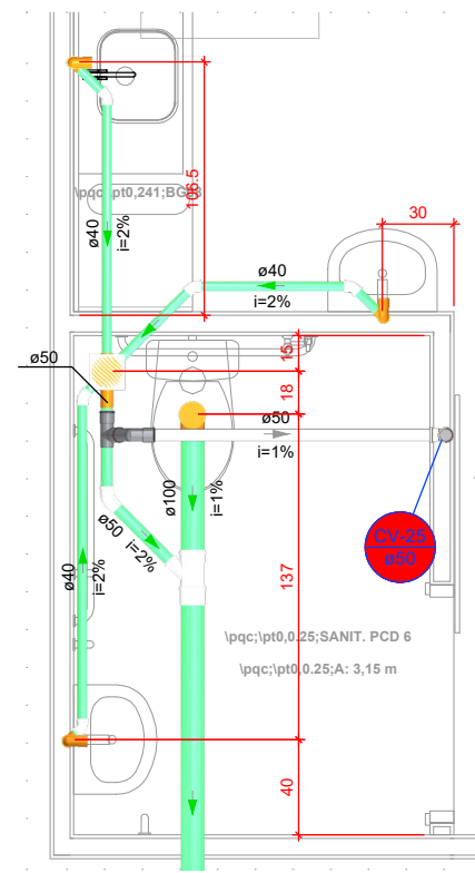
DETALHE SAN-13 1:25
