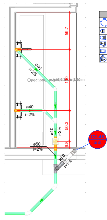
DETALHE SAN-21 1:25
