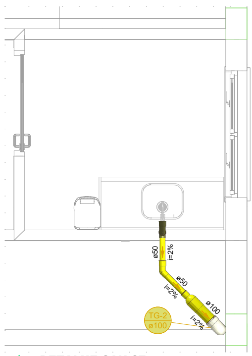
DETALHE SAN-37 1:25
