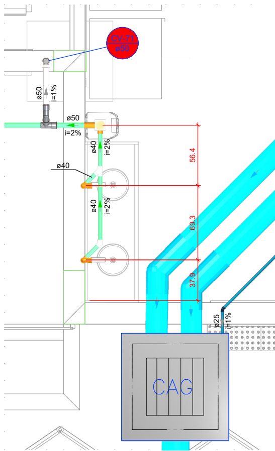
DETALHE SAN-33 1:25
