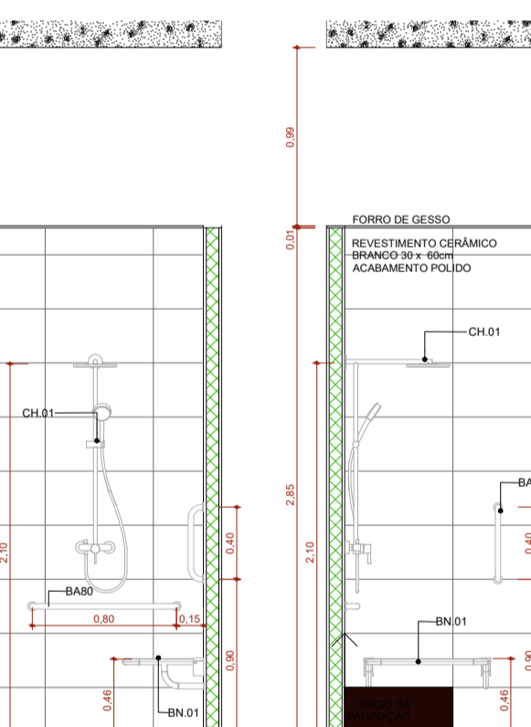
Ban. Quartos Internação VISTA 2 Escala: 1:25
