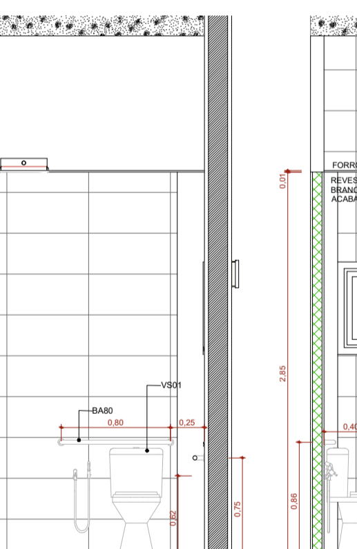
Ban. Quartos Internação VISTA 3 Escala: 1:25
