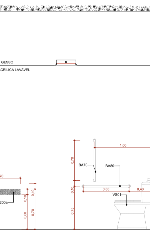
San. Familiar VISTA 2 Escala: 1:25
