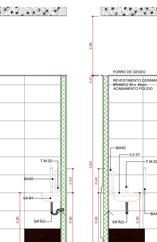
Ban. Quartos Internação VISTA 1 Escala: 1:25
