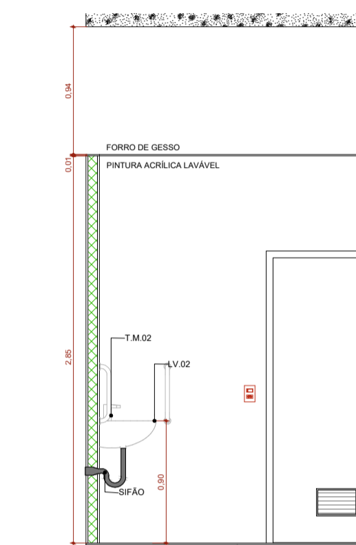
San. Familiar VISTA 4 Escala: 1:25
