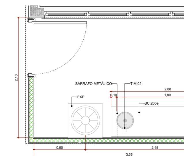
Sala de Utilidades Escala: 1:25
