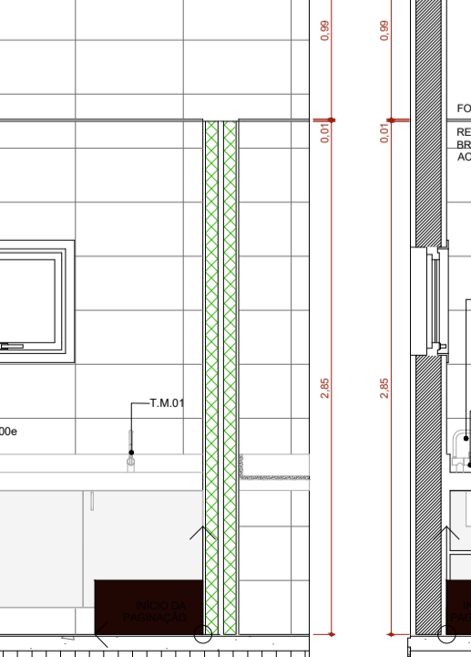
Sala de Utilidades VISTA 1 Escala: 1:25
