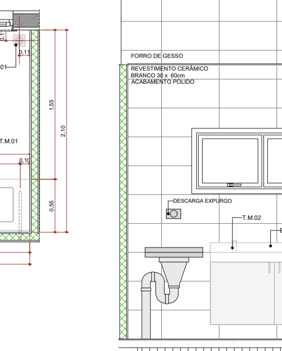
Sala de Utilidades VISTA 1 Escala: 1:25
