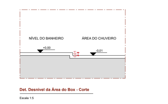
Det. Detalhe da Área do Box - Corte Escala: 1:5
