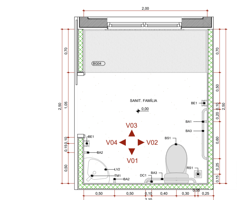
PLANTA BAIXA - SANITÁRIO FAMÍLIA 1:25
