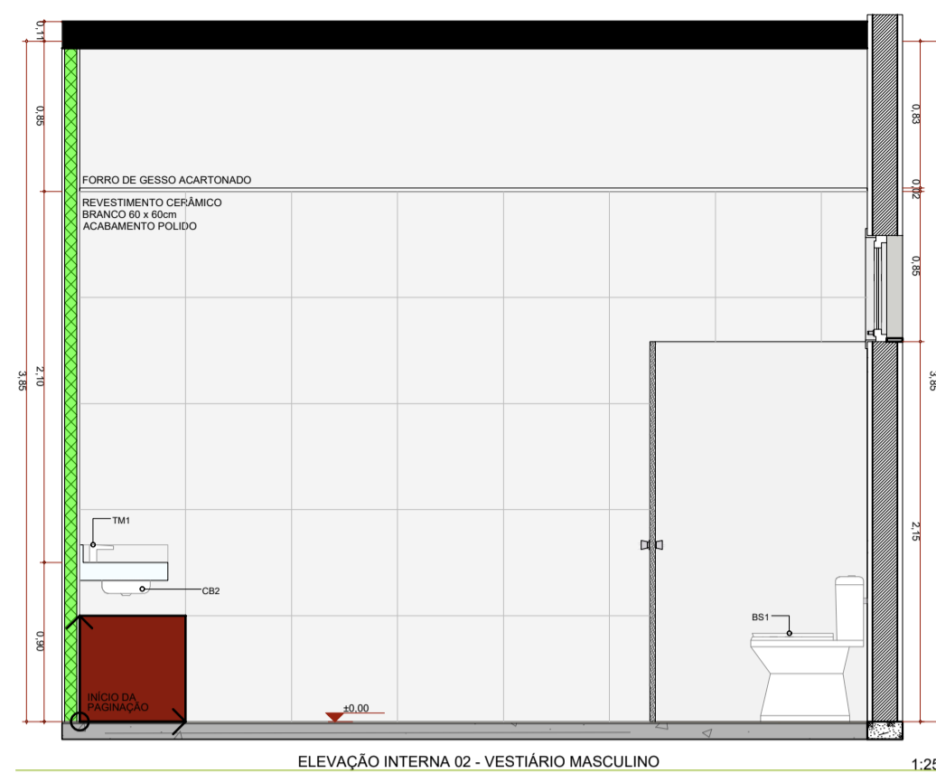
ELEVAÇÃO INTERNA 02 - VESTIÁRIO MASCULINO 1:25
