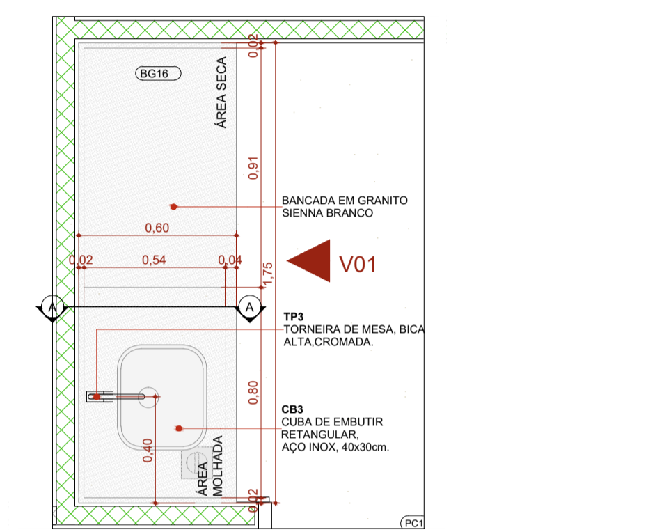
PLANTA BAIXA - BG16 1:20
