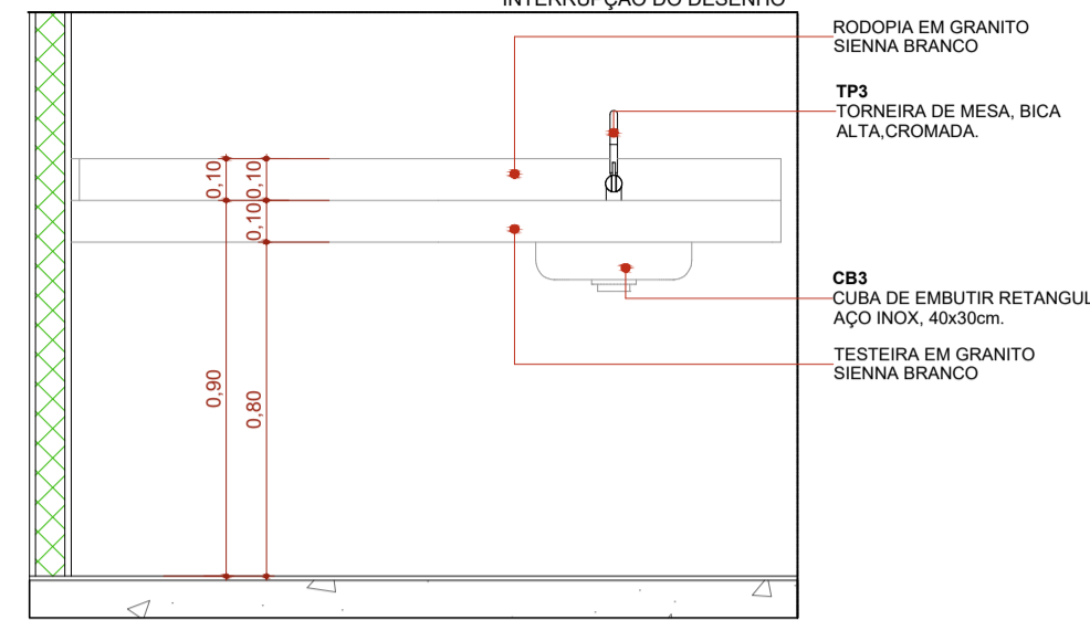
ELEVAÇÃO 01 - BG15 1:20
