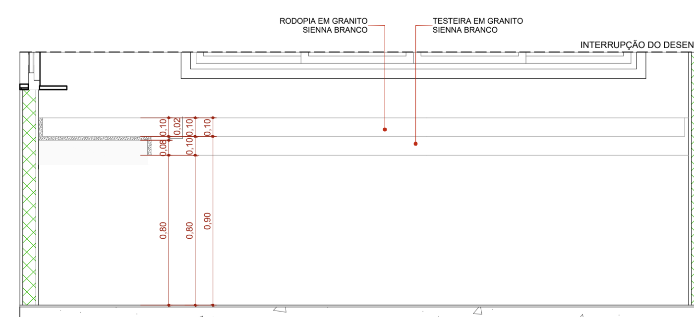
ELEVÇÃO 01 - BG14
