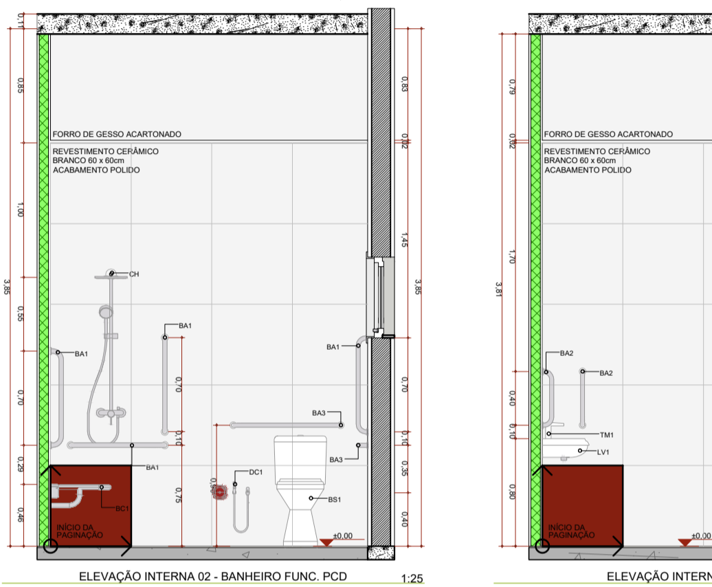
ELEVAÇÃO INTERNA 02 - BANHEIRO FUNC. PCD 1:25
