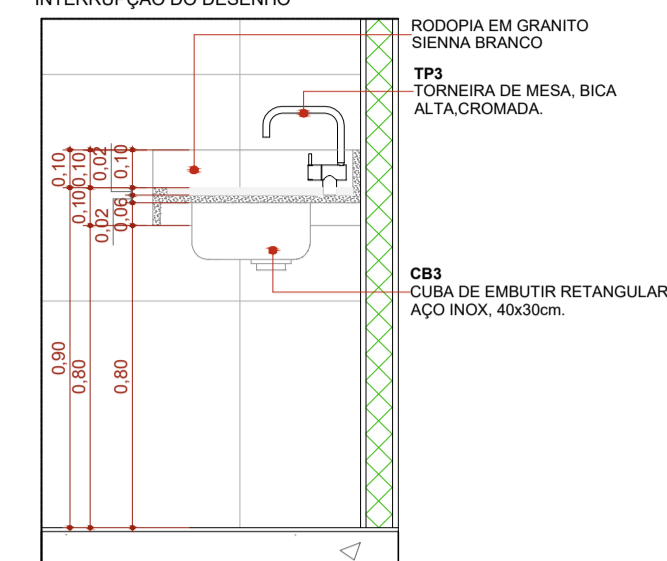
CORTE A - BG15 1:20
