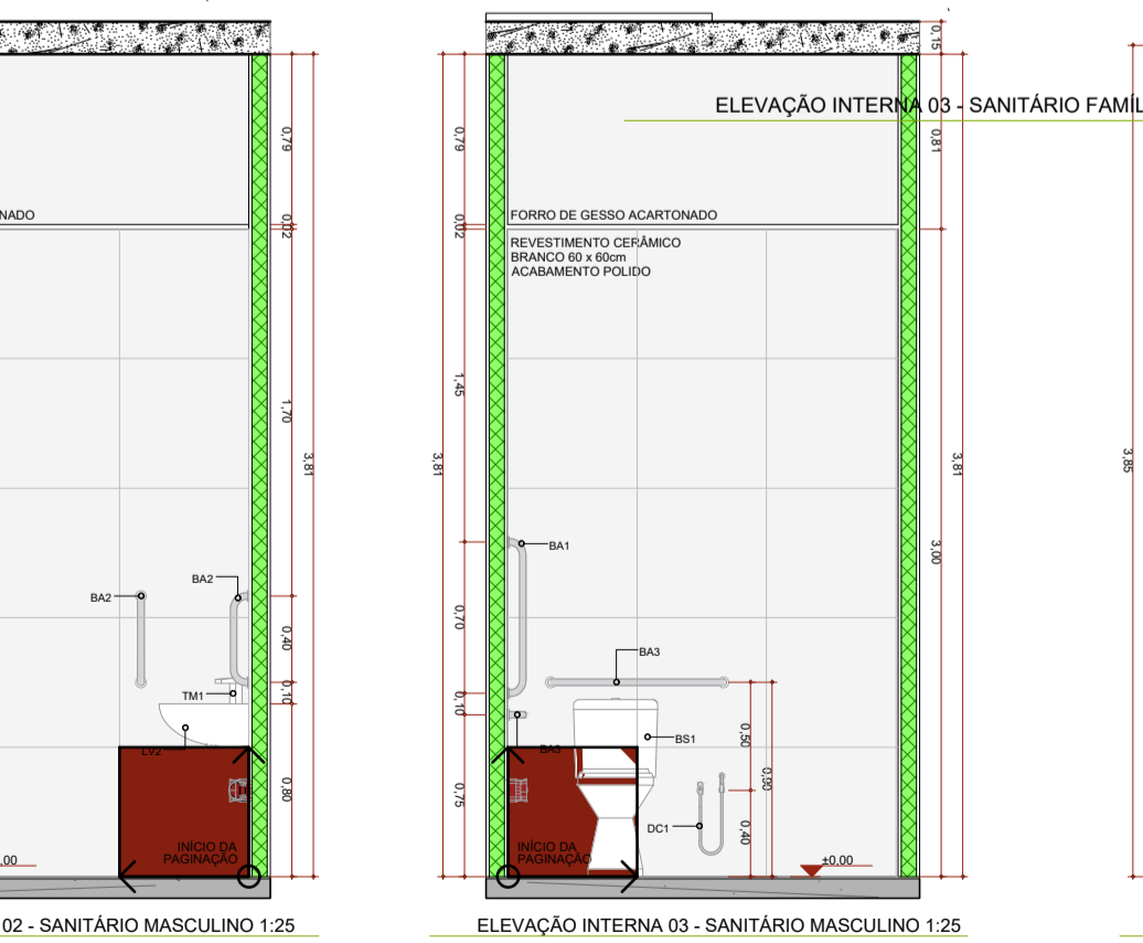
ELEVAÇÃO INTERNA 02 - SANITÁRIO MASCULINO 1:25
