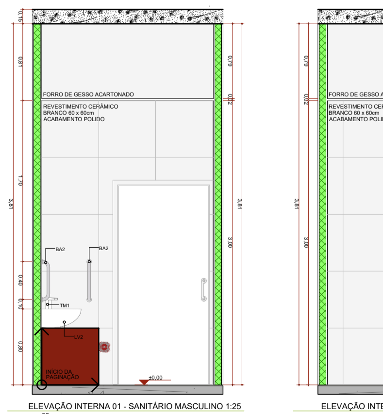
ELEVAÇÃO INTERNA 01 - SANITÁRIO MASCULINO 1:25
