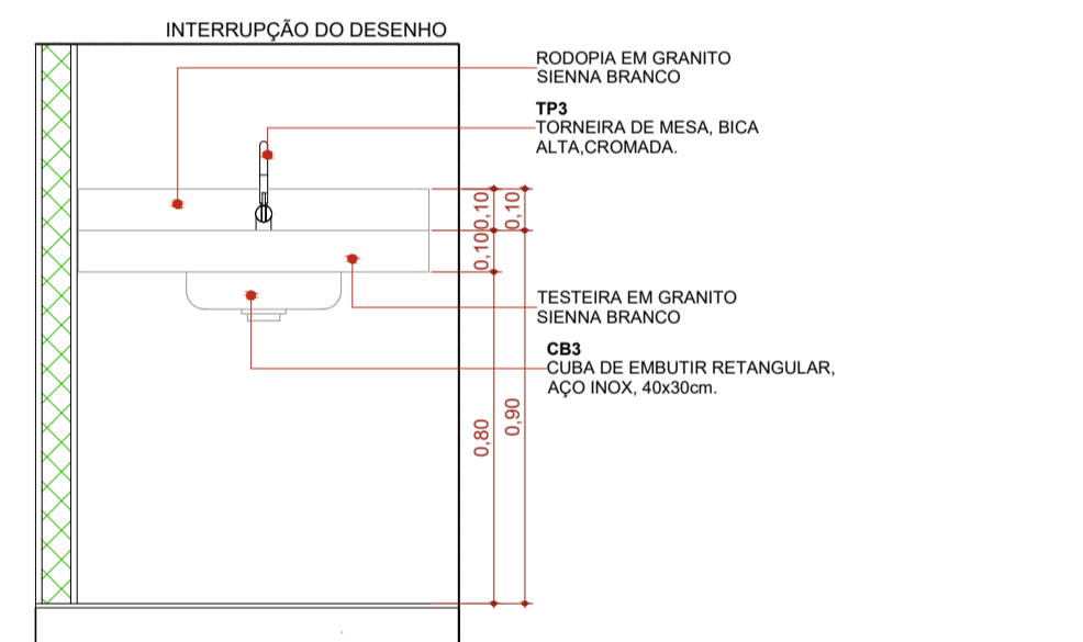
ELEVAÇÃO 01 - BG17 1:20
