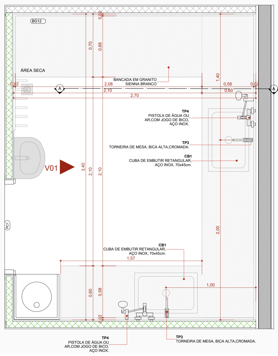
PLANTA BAIXA - BG12
