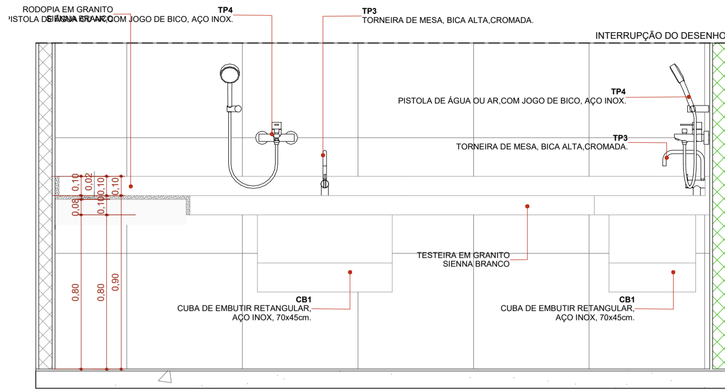
ELEVÇÃO 01 - BG12
