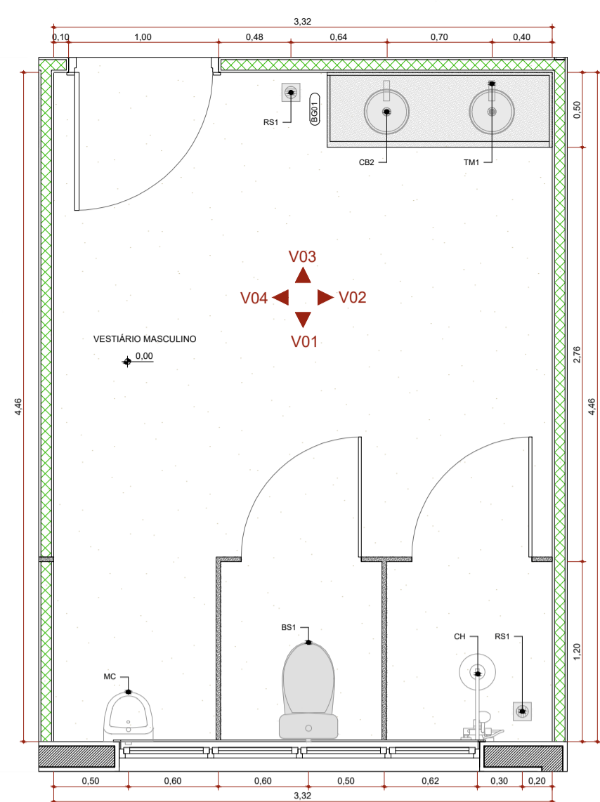
PLANTA BAIXA - VESTIÁRIO MASCULINO 1:25
