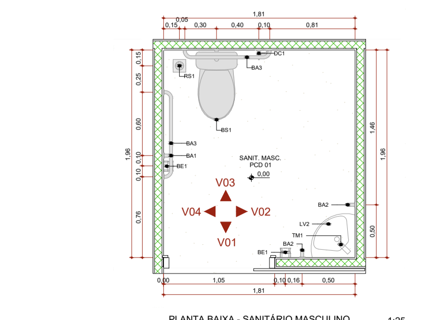
PLANTA BAIXA - SANITÁRIO MASCULINO 1:25
