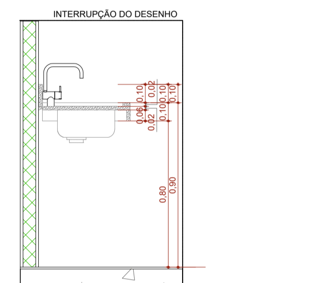
CORTE A - BG17 1:20
