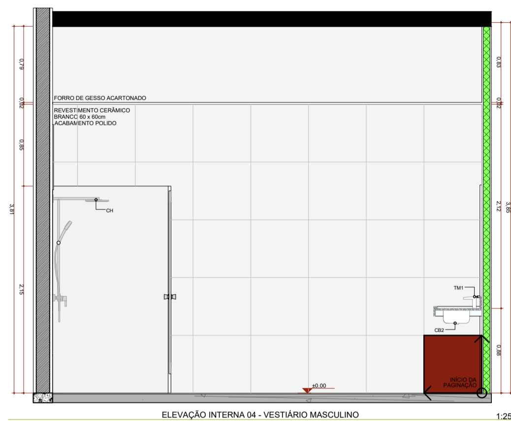
ELEVAÇÃO INTERNA 04 - VESTIÁRIO MASCULINO 1:25
