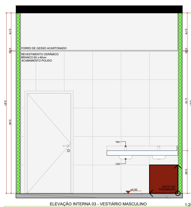
ELEVAÇÃO INTERNA 03 - VESTIÁRIO MASCULINO 1:25
