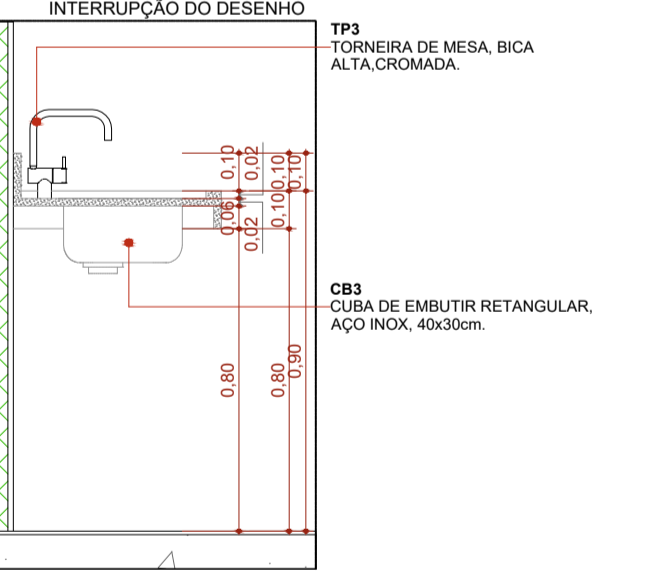
CORTE A - BG18 1:20
