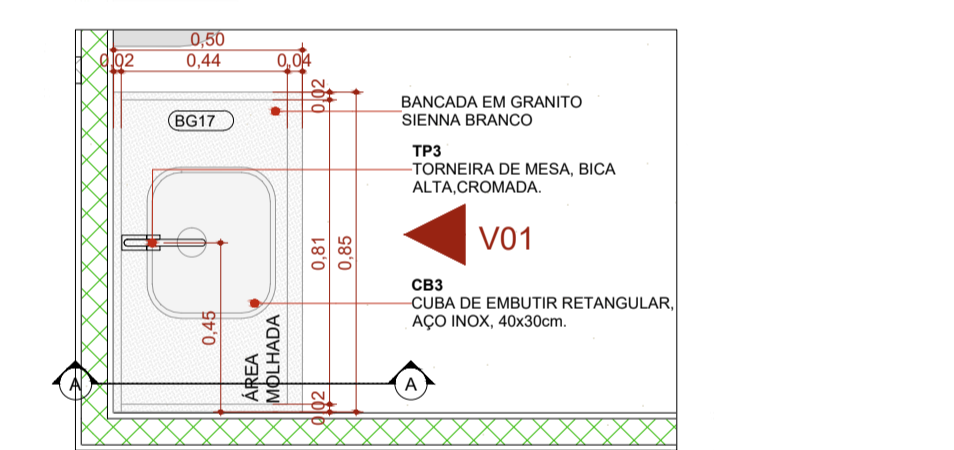
PLANTA BAIXA - BG17 1:20
