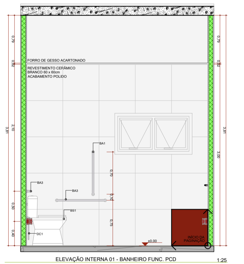
ELEVAÇÃO INTERNA 01 - BANHEIRO FUNC. PCD 1:25
