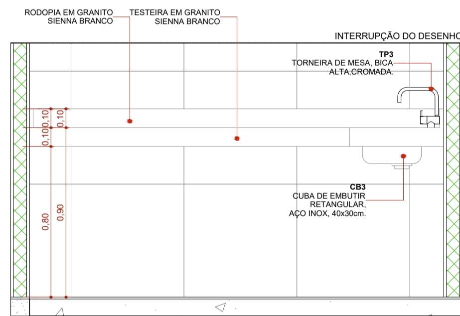
ELEVÇÃO 01 - BG11 1:20
