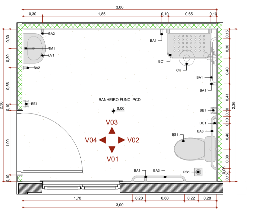
PLANTA BAIXA - BANHEIRO FUNC. PCD 1:25
