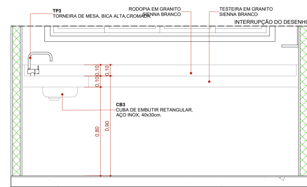
ELEVÇÃO 01 - BG13
