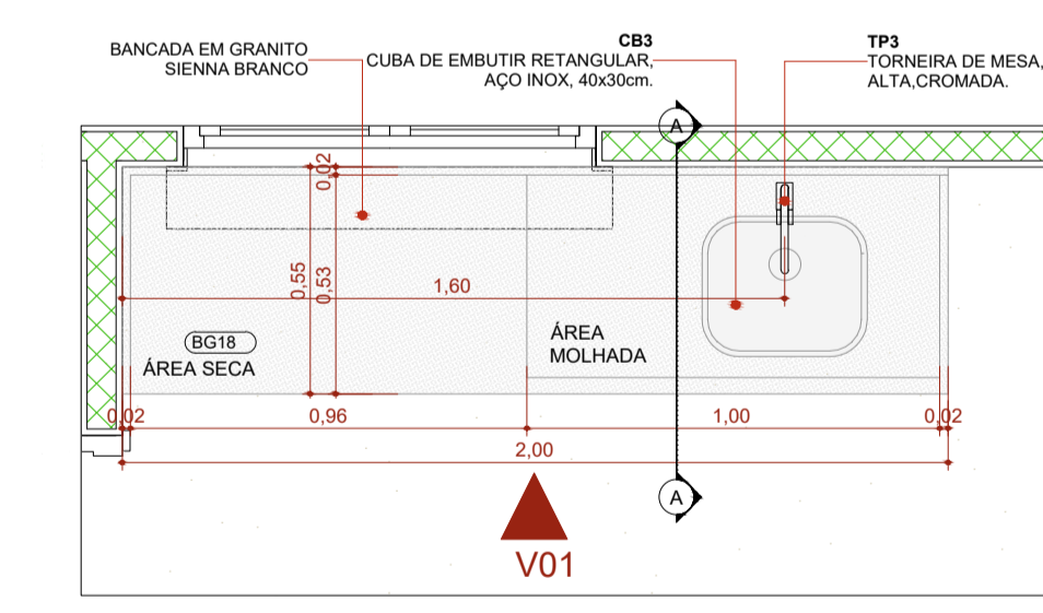
PLANTA BAIXA - BG18 1:20
