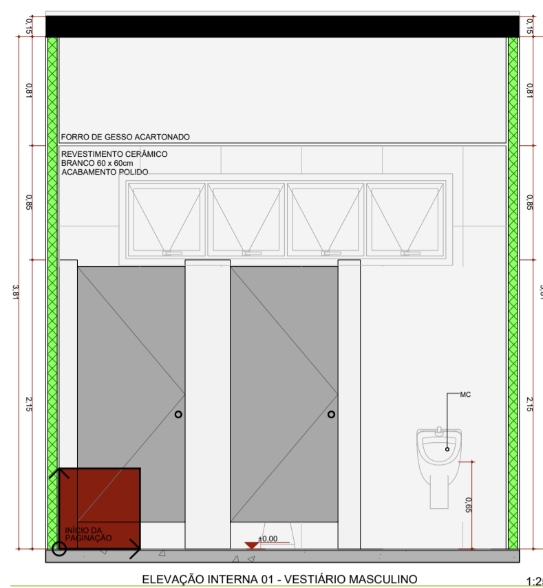
ELEVAÇÃO INTERNA 01 - VESTIÁRIO MASCULINO 1:25
