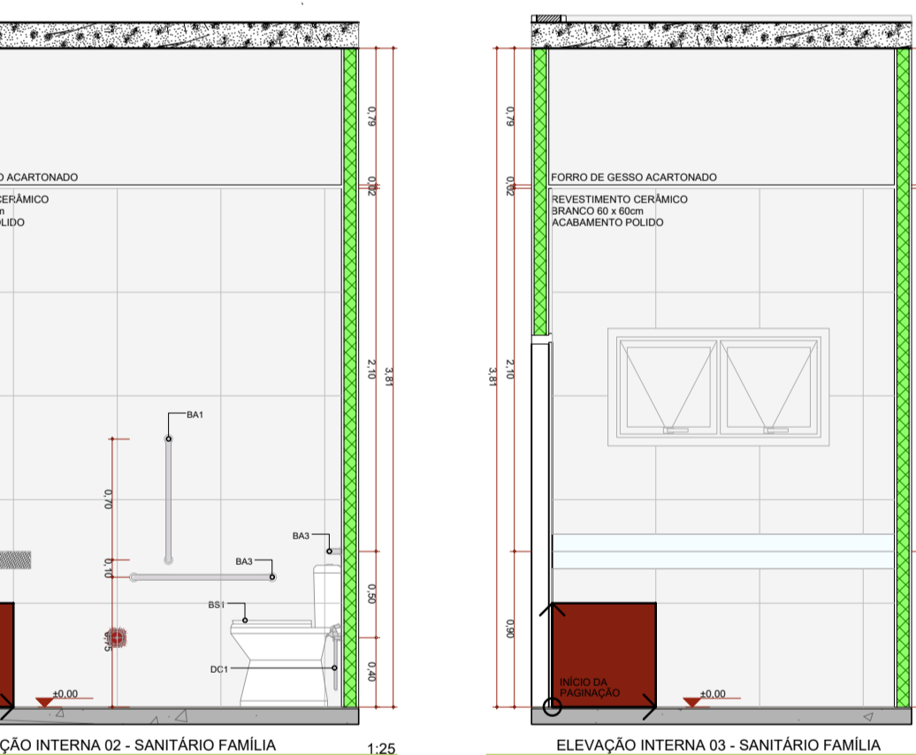
ELEVAÇÃO INTERNA 02 - SANITÁRIO FAMÍLIA 1:25
