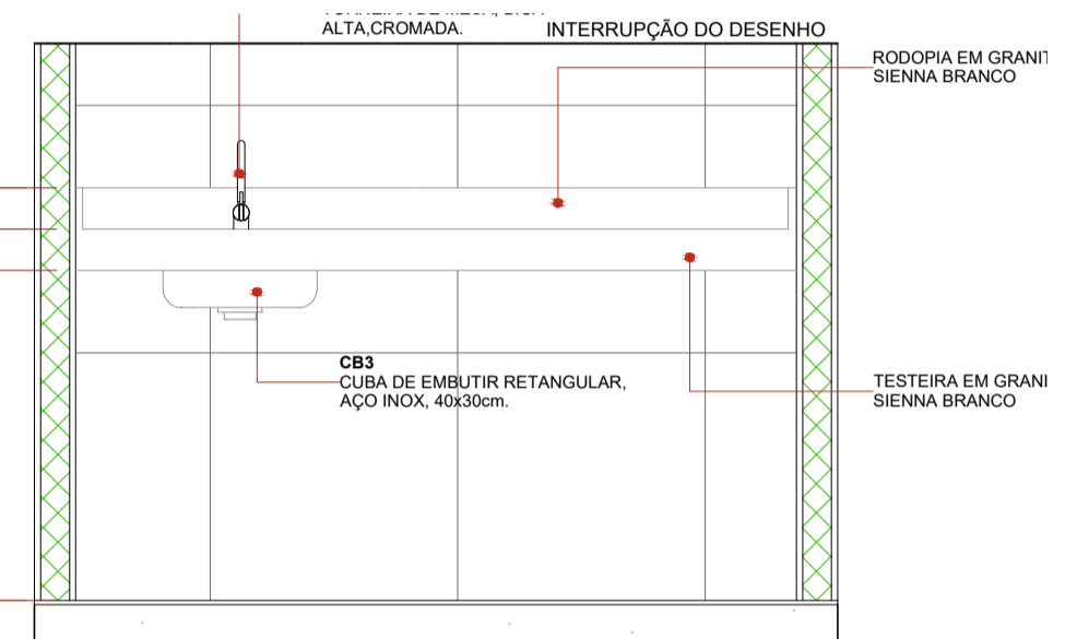
ELEVAÇÃO 01 - BG16 1:20
