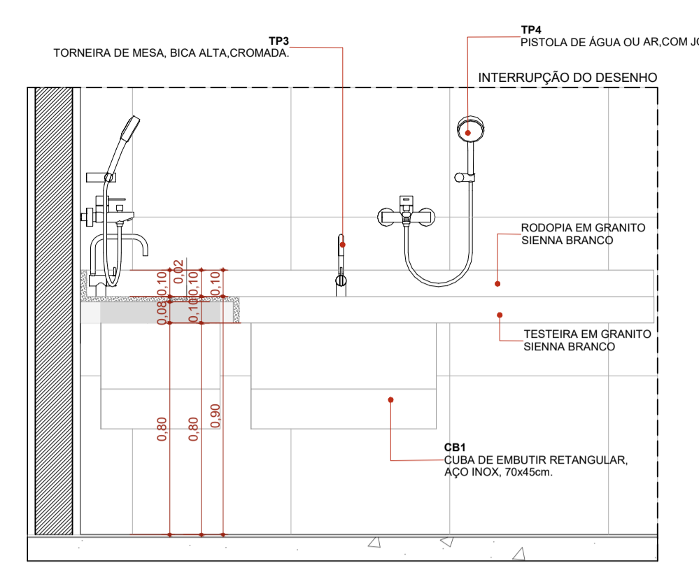
CORTE A - BG12
