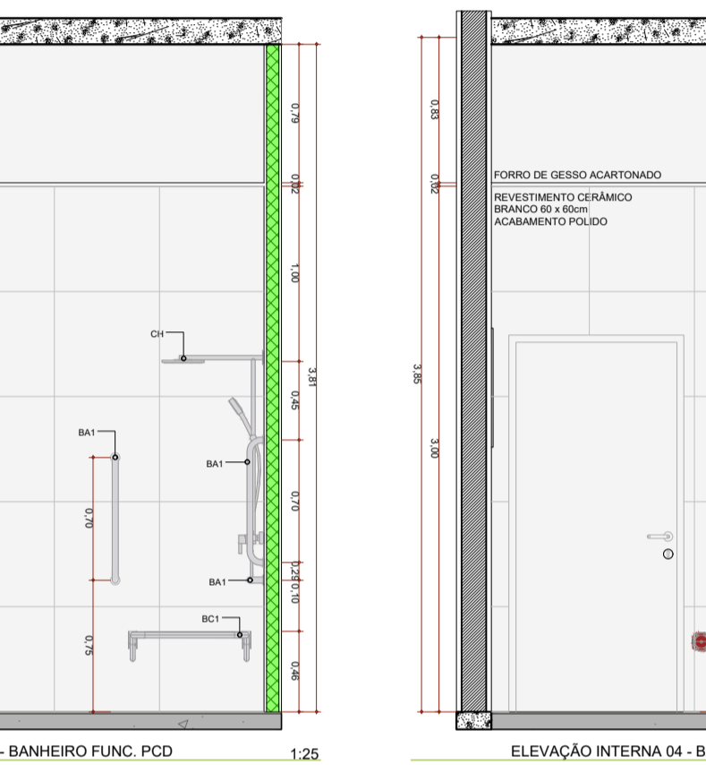
ELEVAÇÃO INTERNA 03 - BANHEIRO FUNC. PCD 1:25
