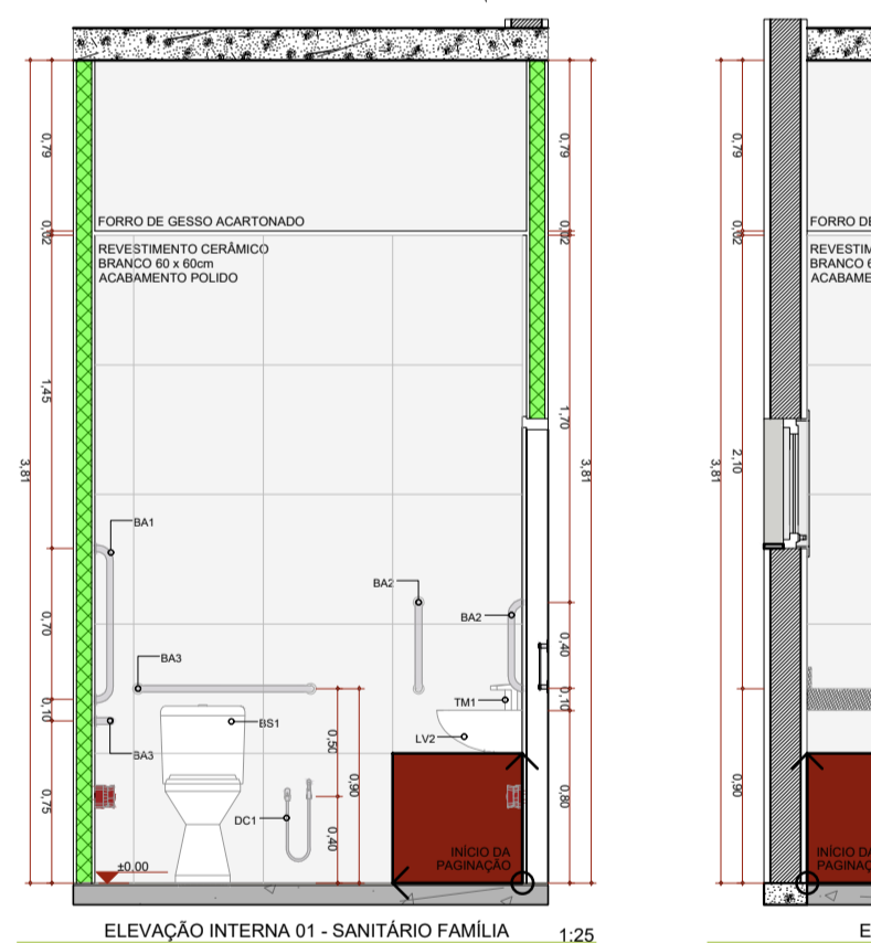
ELEVAÇÃO INTERNA 01 - SANITÁRIO FAMÍLIA 1:25
