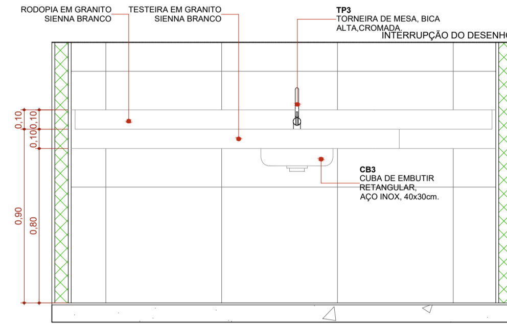
ELEVÇÃO 01 - BG10 1:20
