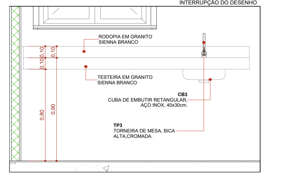
ELEVAÇÃO 01 - BG18 1:20
