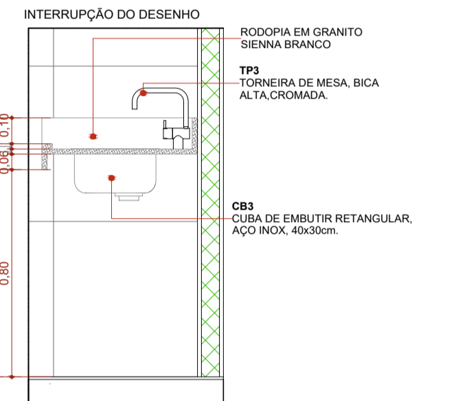
CORTE A - BG16 1:20
