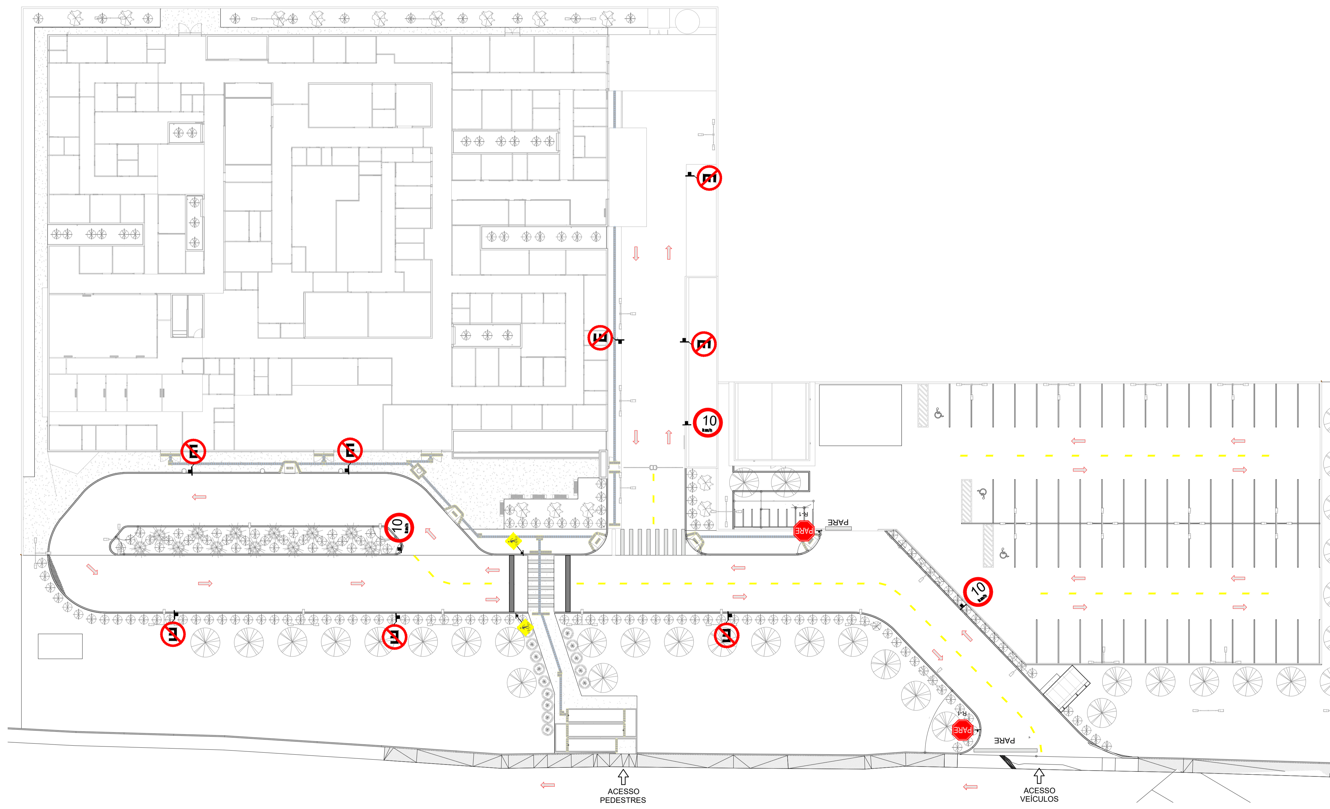
1 ESQUEMA GERAL ESCALA: 1 : 500
