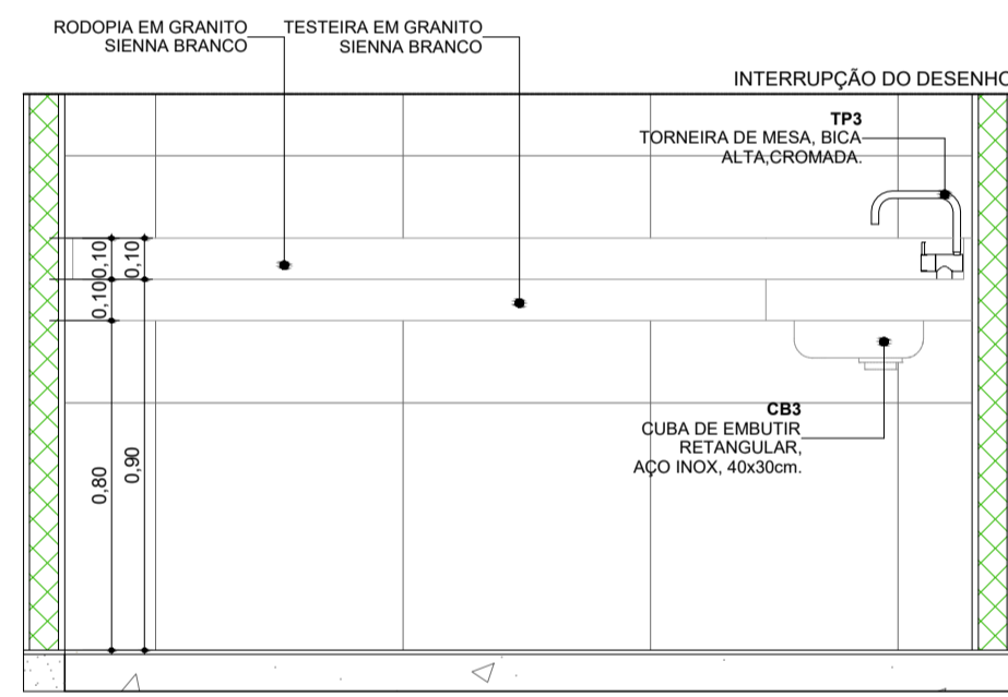
ELEVÇÃO 01 - BG11 1:20
