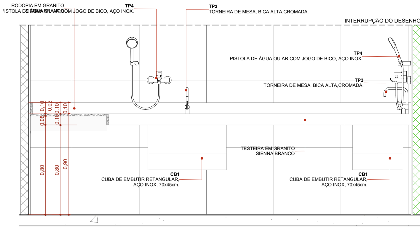
ELEVÇÃO 01 - BG12 1:20
