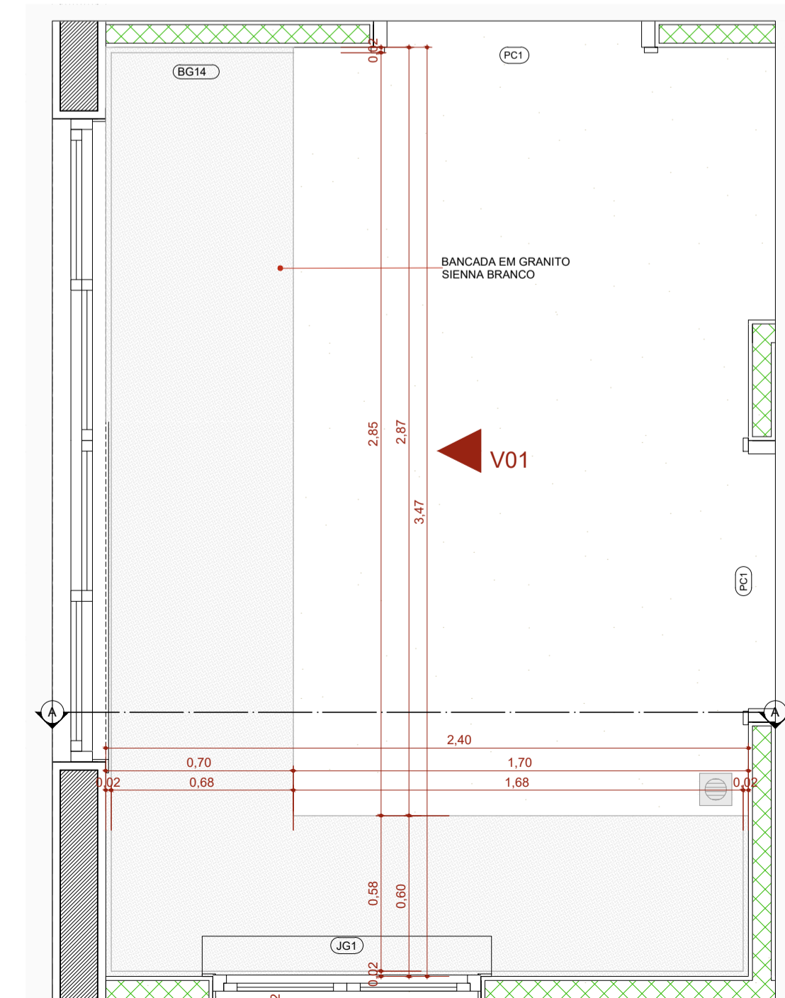
PLANTA BAIXA - BG14 1:20
