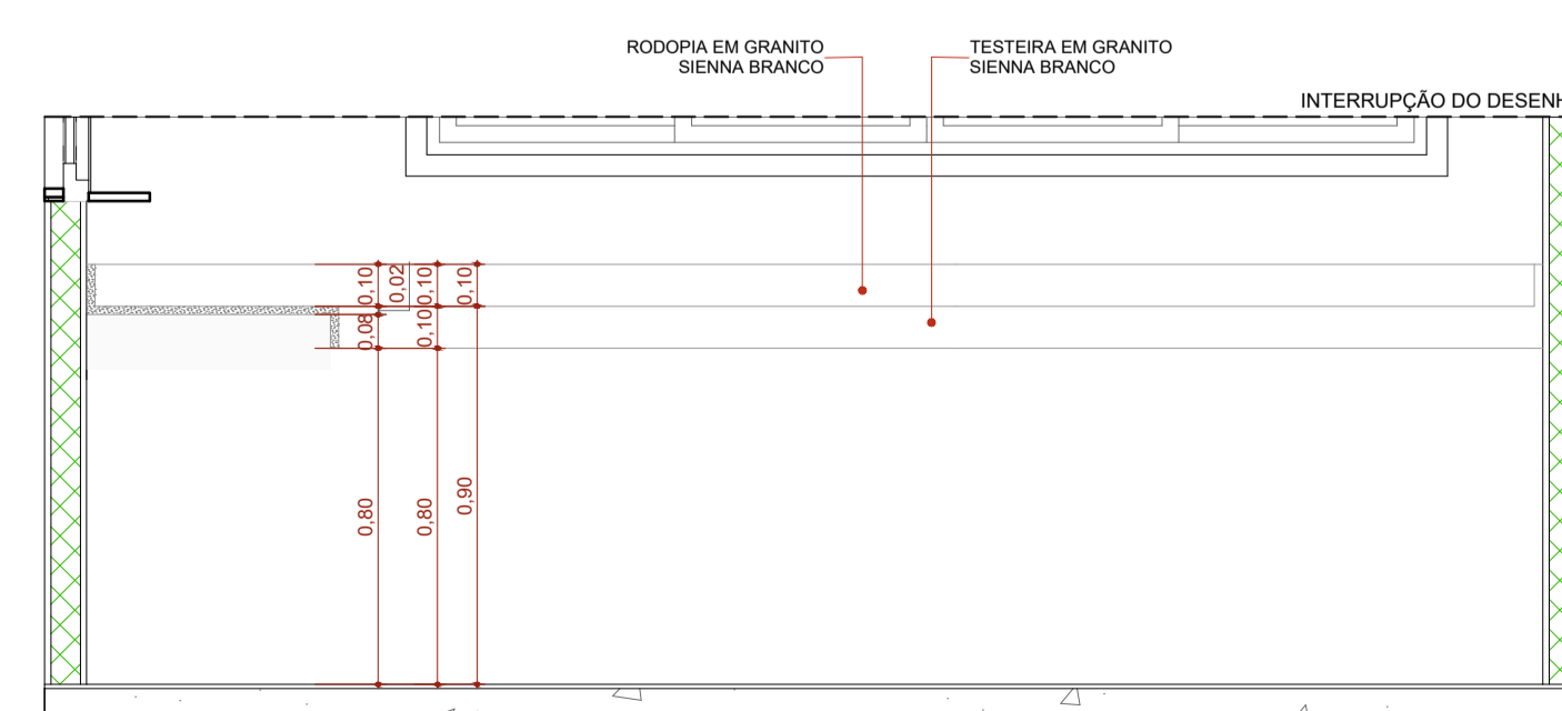
ELEVÇÃO 01 - BG14 1:20
