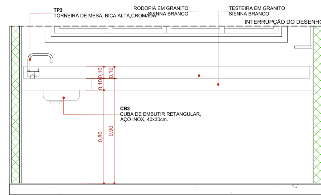
ELEVÇÃO 01 - BG13 1:20
