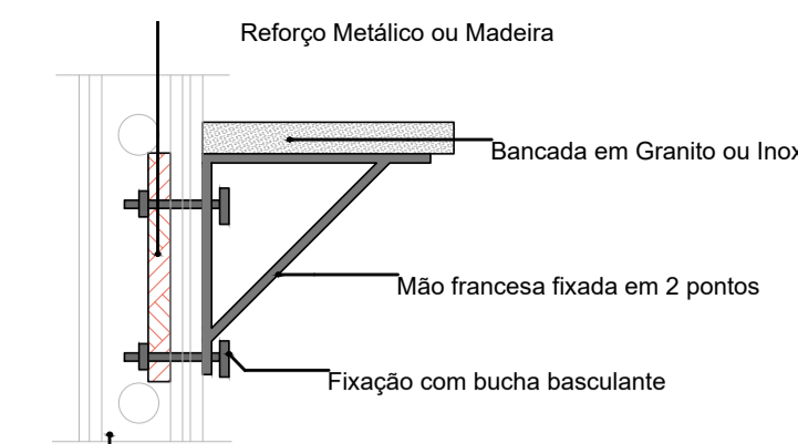
DETALHE 01: REFORÇO EM DRYWALL
