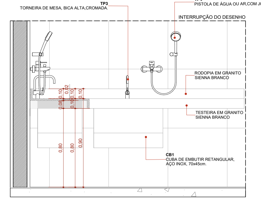
CORTE A - BG12 1:20
