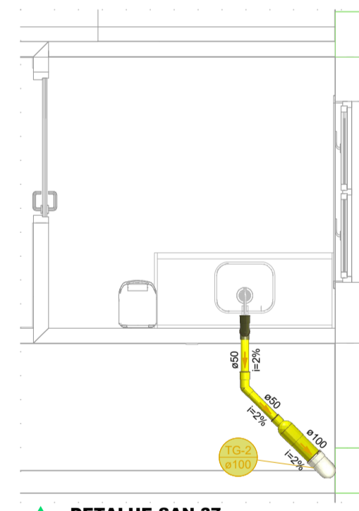
DETALHE SAN-37 1:25
