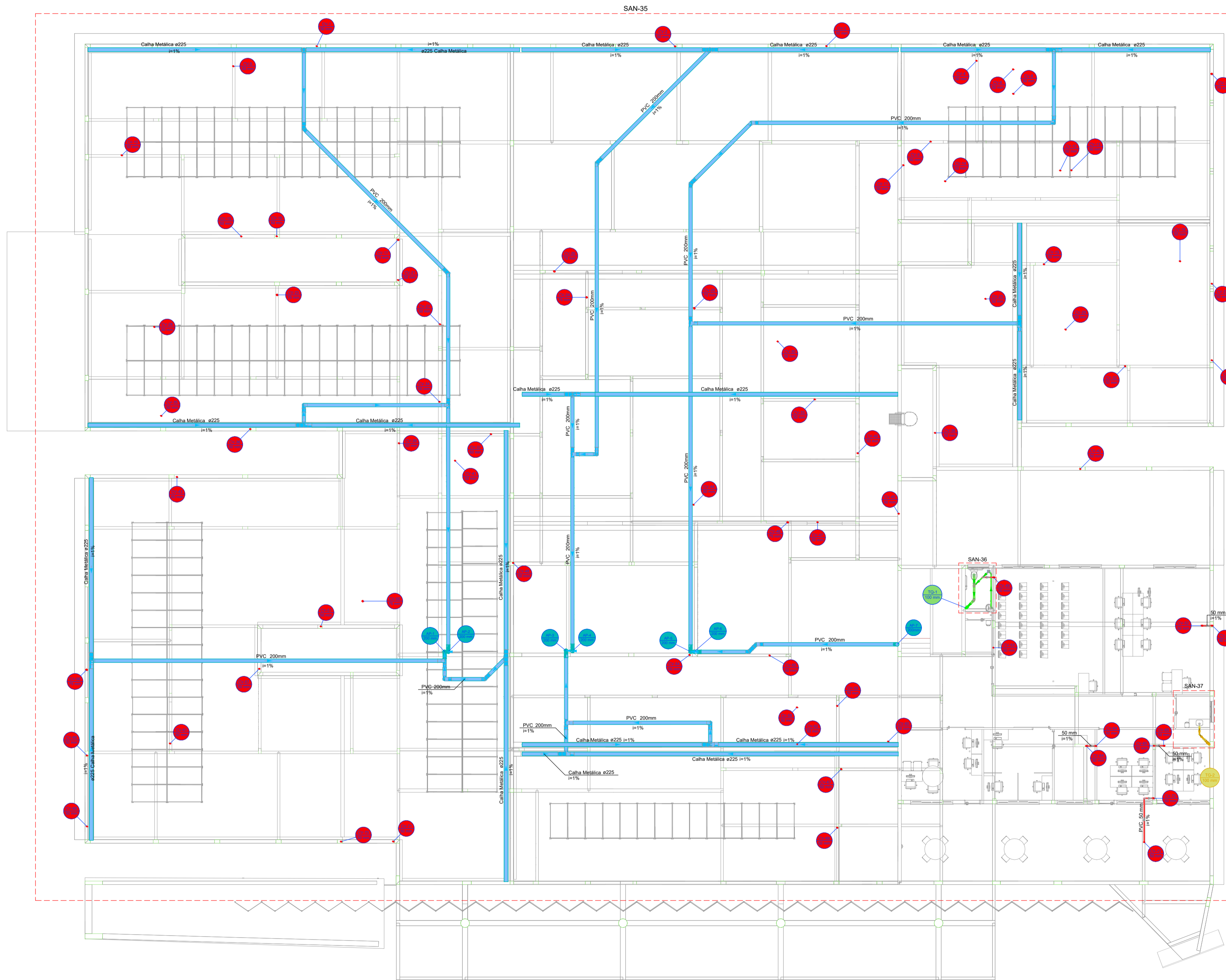
PLANTA - SANITÁRIO - MEZANINO ESC. 1/100
