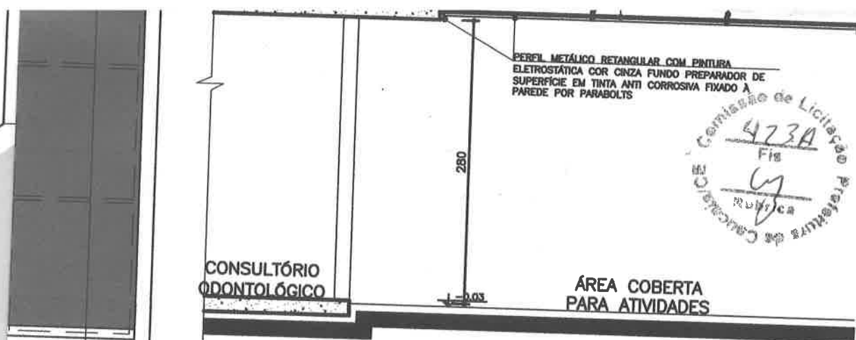
06 Seção A A'-Marquise Sala de Atividades Esc.: 1:50
