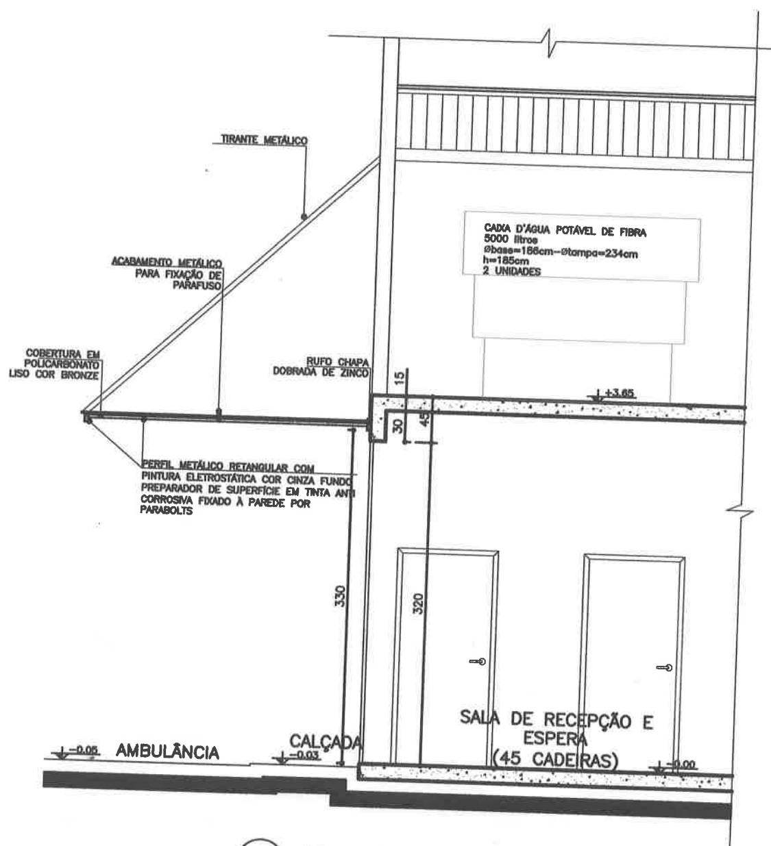
03 Seção A A'- Marquise Entrada Principal Esc.: 1:50
