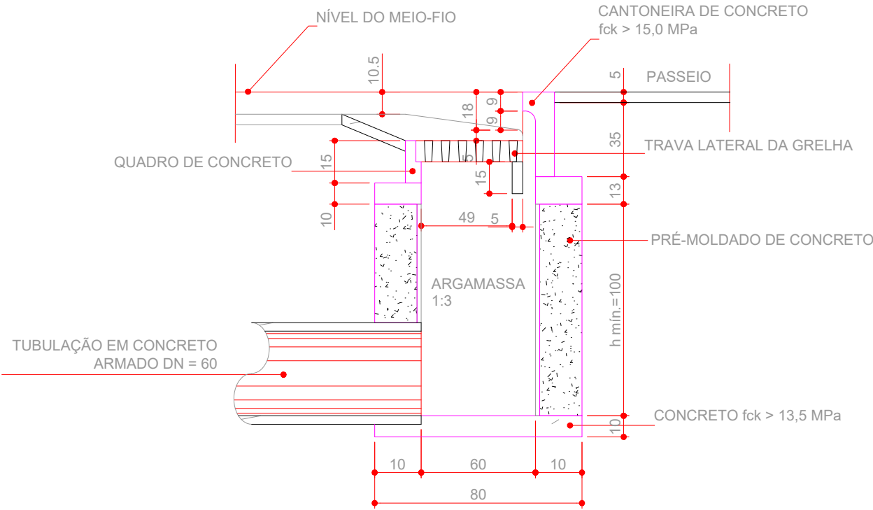
CORTE BB SEM ESCALA
