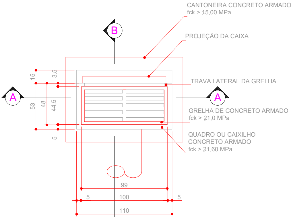
PLANTA SEM ESCALA
