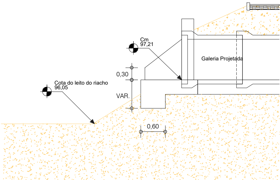
CORTE - AA'
