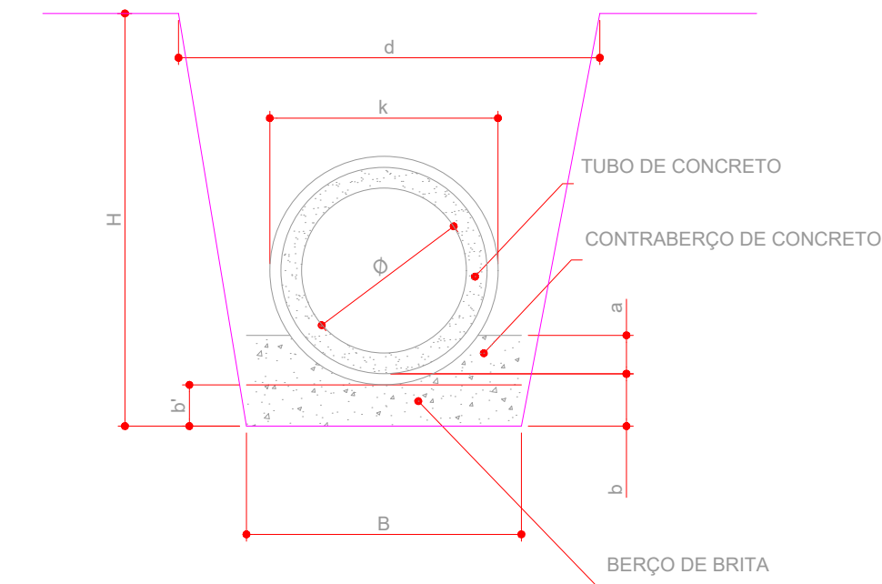
CORTE TRANSVERSAL SEM ESCALA
