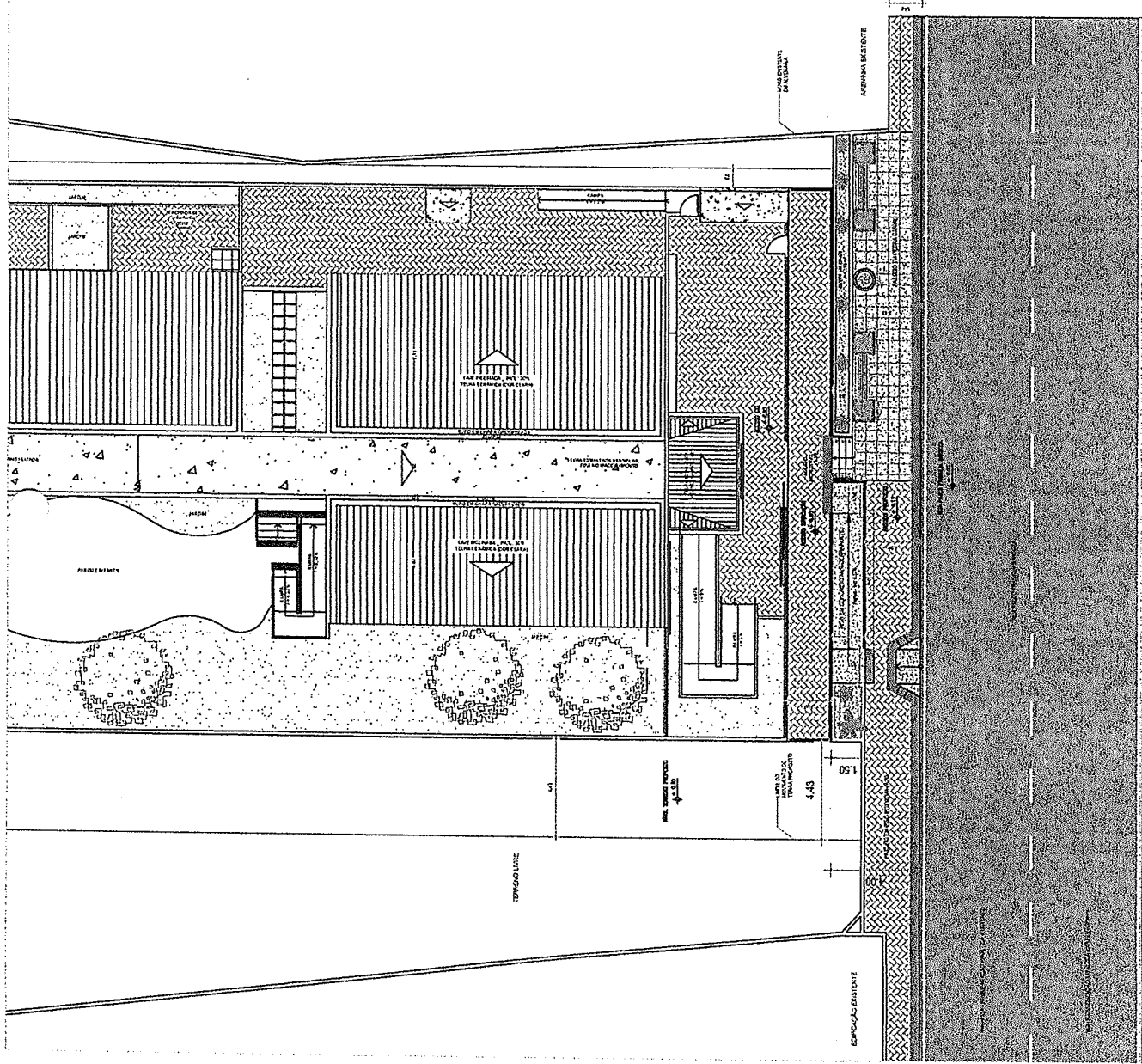
01 PLANTA DE IMPLANTAÇÃO ESCALA: 1/200
