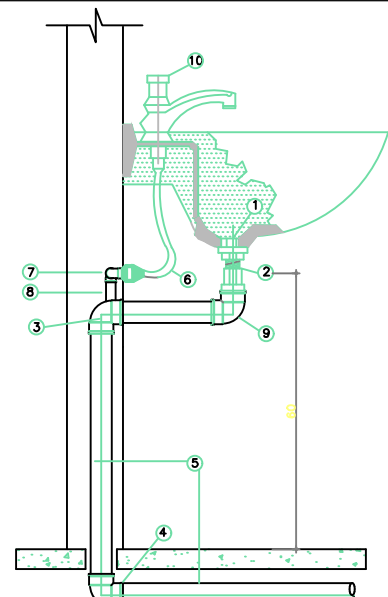
DETALHE LIGAÇÃO DE LAVATÓRIO SEM ESCALA
