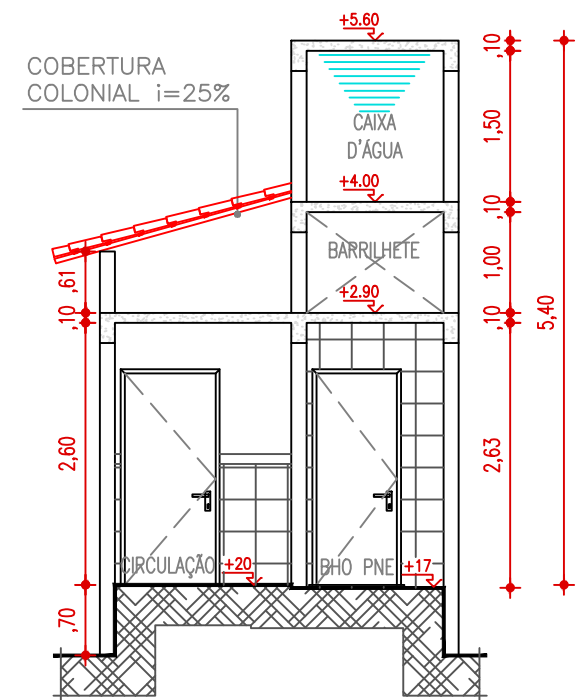
CORTE EE ESC. 1:75
