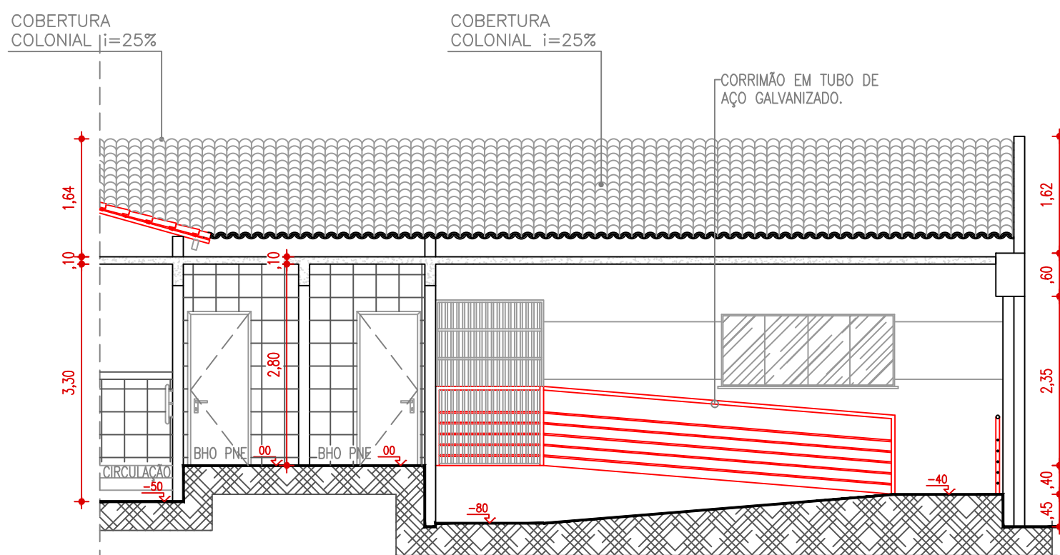
CORTE DD ESC. 1:75
