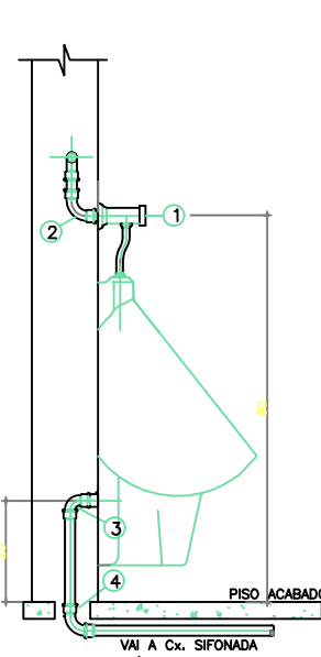
DETALHE LIGAÇÃO DO MICTÓRIO INFANTIL SEM ESCALA
