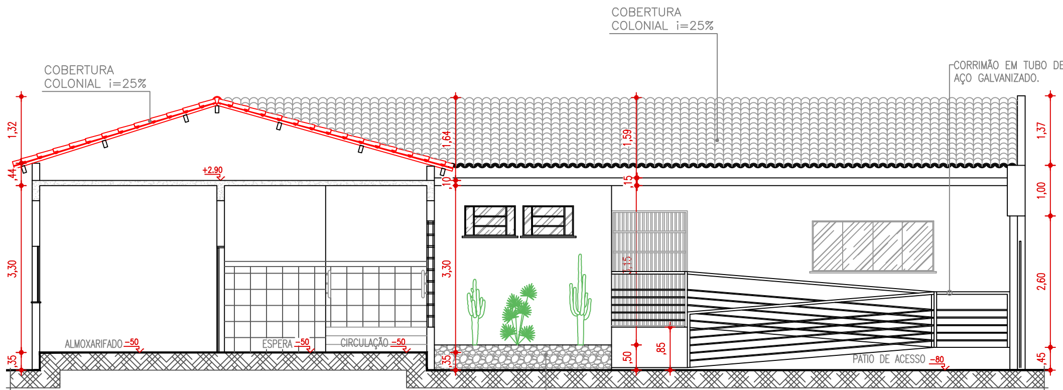
CORTE CC ESC. 1:75
