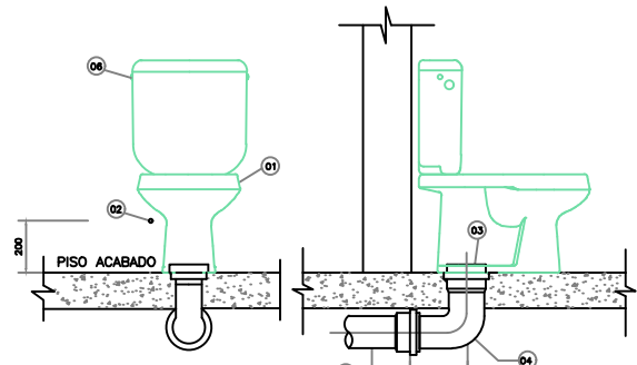
DETALHE VASO SANITÁRIO SEM ESCALA
