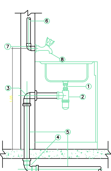
DETALHE PIA COM SIFAO SEM ESCALA
