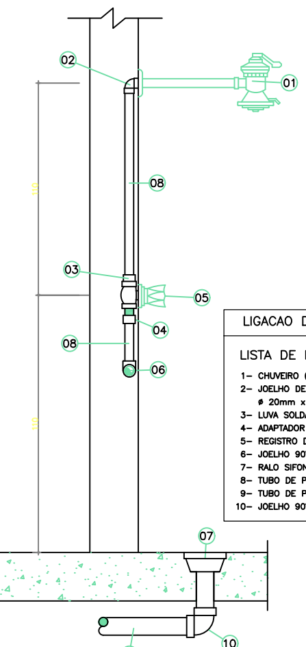
DETALHE LIGAÇÃO DO CHUVEIRO SEM ESCALA
