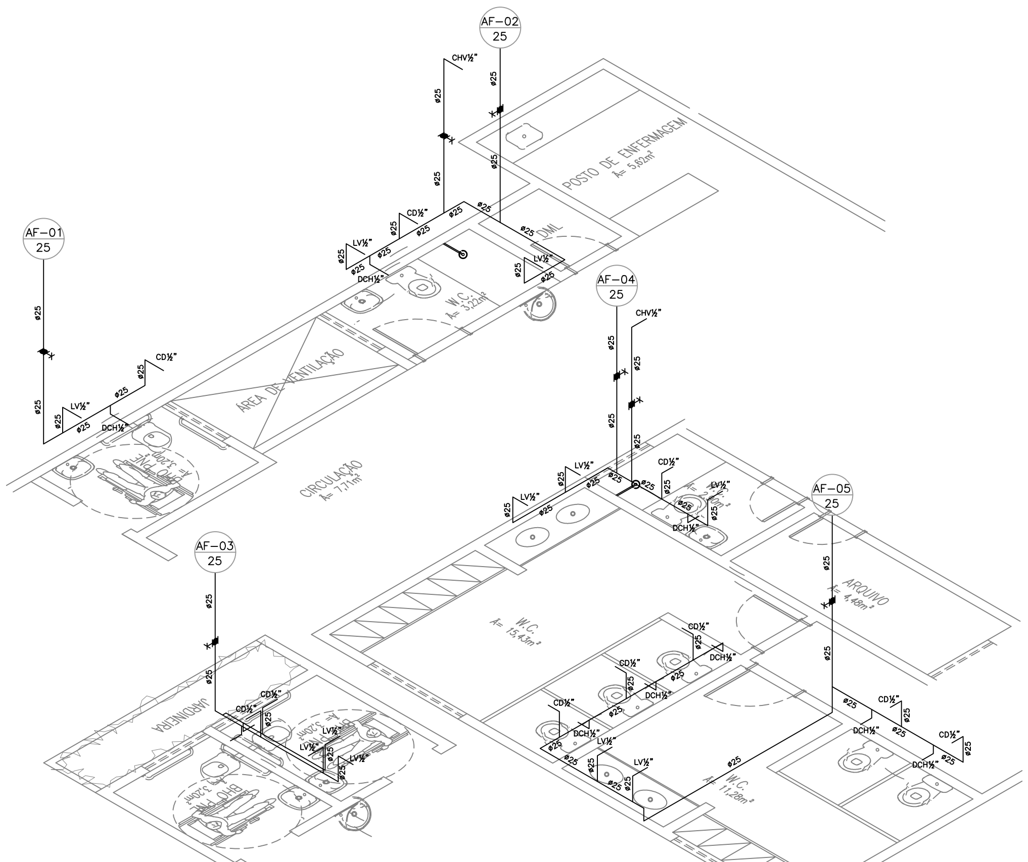
ISOMÉTRICO SEM ESCALA
