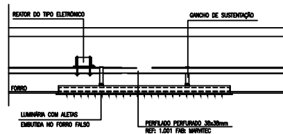
DET. FIXAÇÃO DE LUM. FLUORESCENTE ESCALA 1/8
