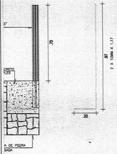
FIXAÇÃO DAS BALIZAS
