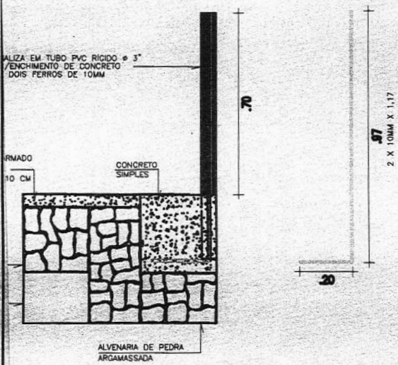
DETALHE DE FIXAÇÃO DAS BALIZAS ESC.: 1/10
