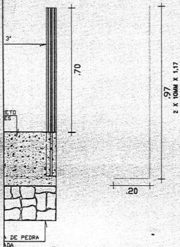
FIXAÇÃO DAS BALIZAS
