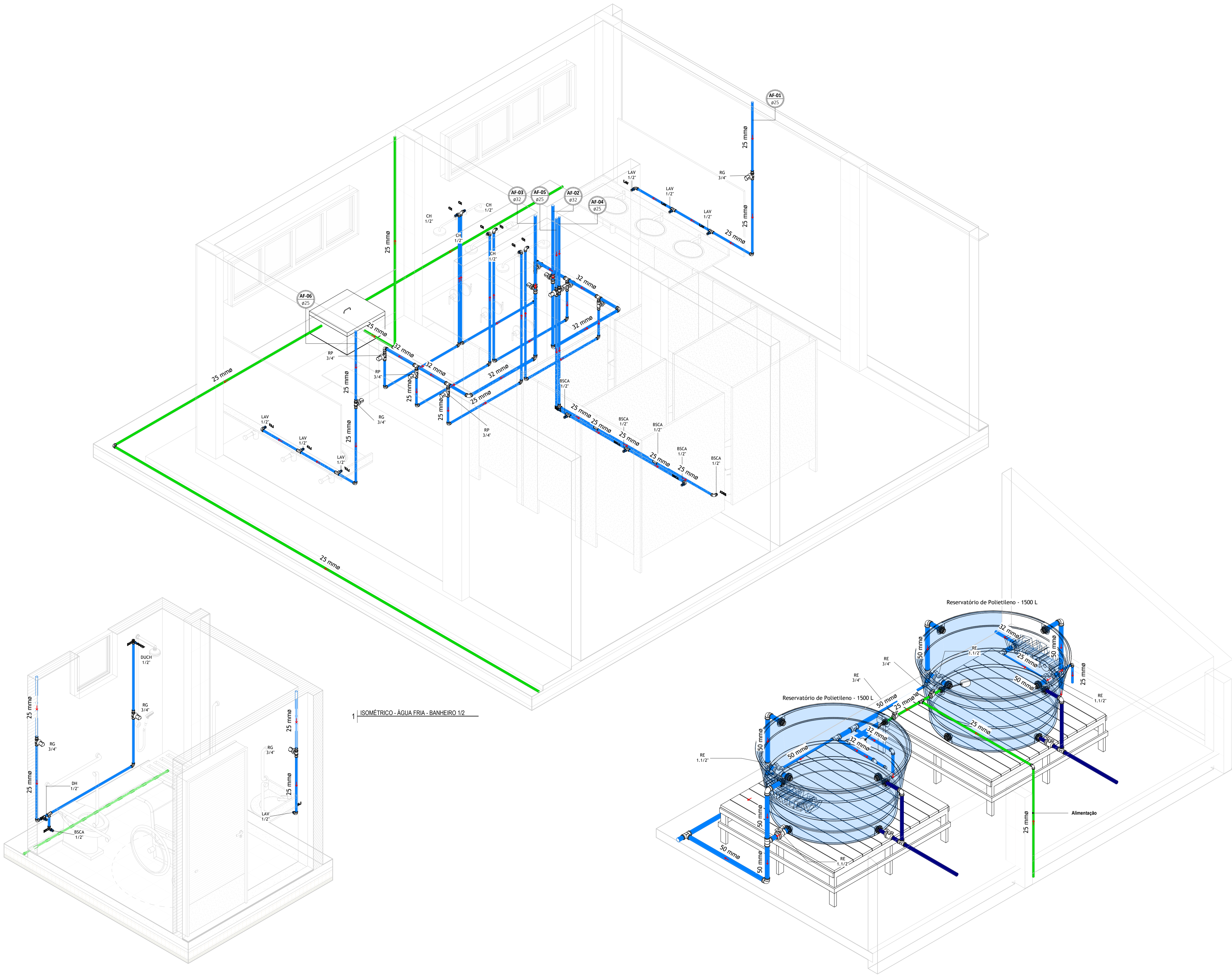
3 | ISOMÉTRICO - ÁGUA FRIA - CAIXA D'ÁGUA 01
