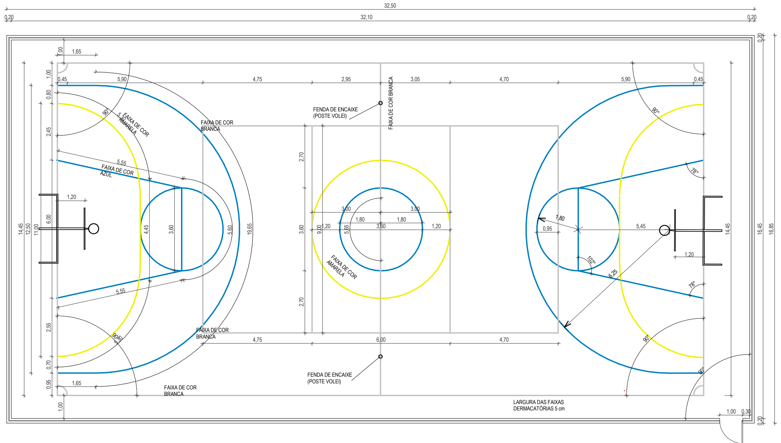
1 DETALHE PINTURA QUADRA POLIESPORTIVA 1:100
