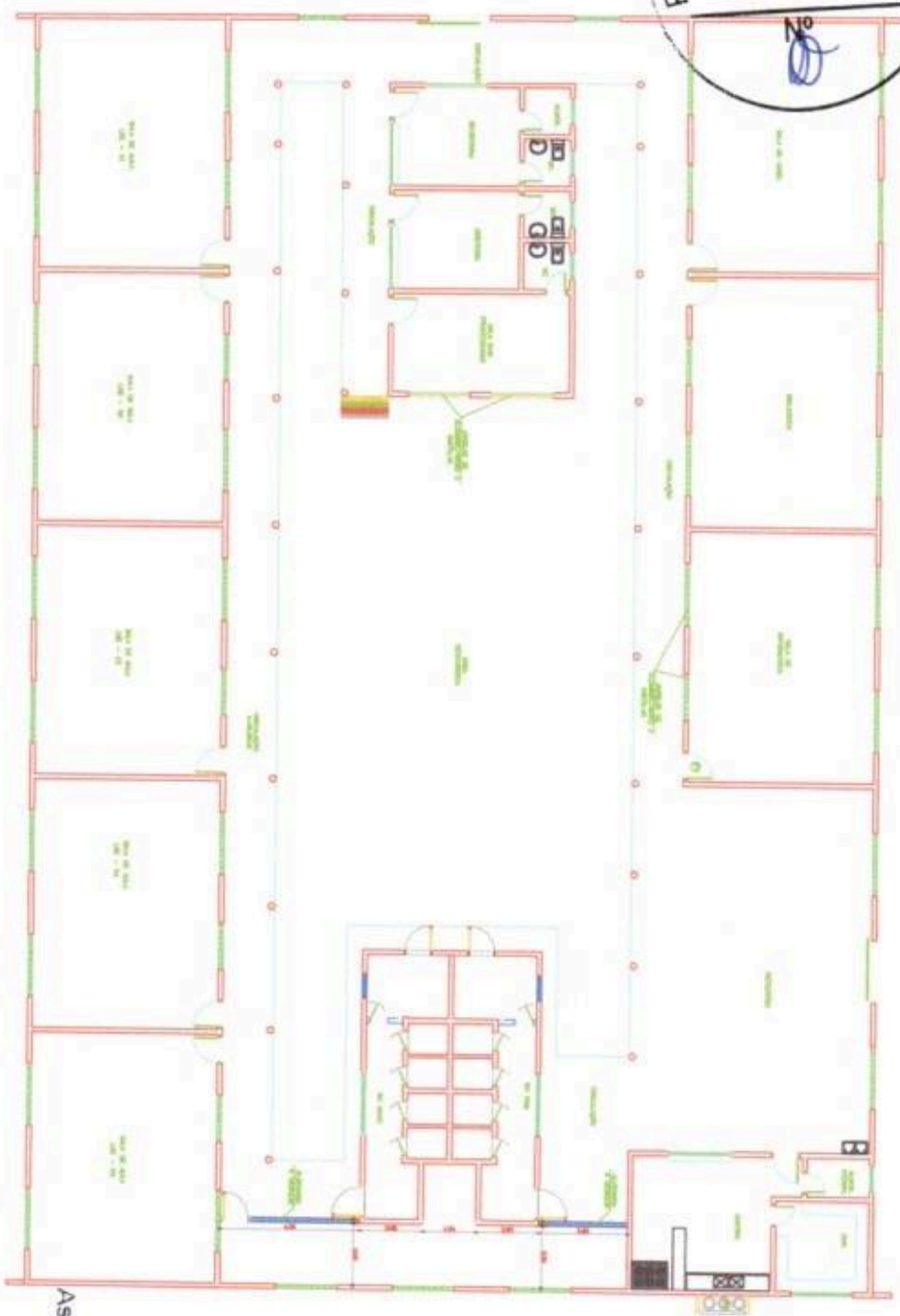
01 PLANTA BAIXA EXISTENTE ESCOLA - 1 : 100
