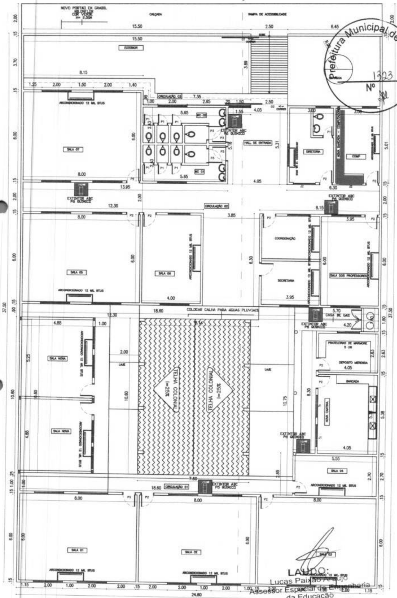
1 - PLANTA DE REFORMA
