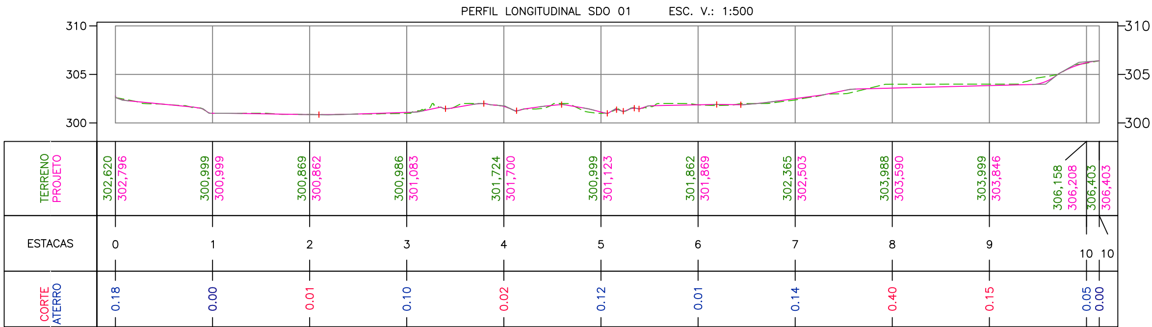
2 PERFIL LONGITUDINAL SDO 01 ESC 1:500
