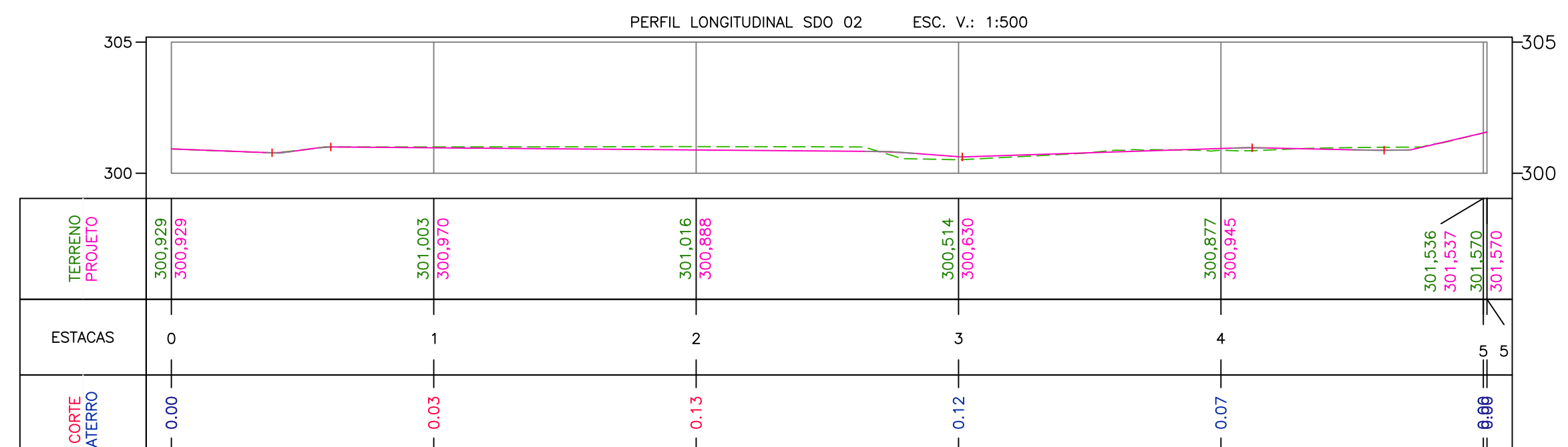
3 PERFIL LONGITUDINAL SDO 02 ESC 1:500
