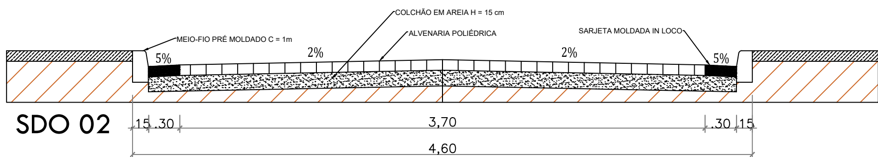
2 CORTE TRANSVERSAL DA PAVIMENTAÇÃO SEM ESC
