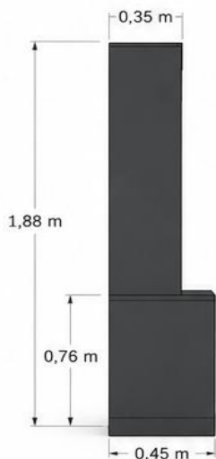
VISTA LATERAL (PROFUNDIDADE)
