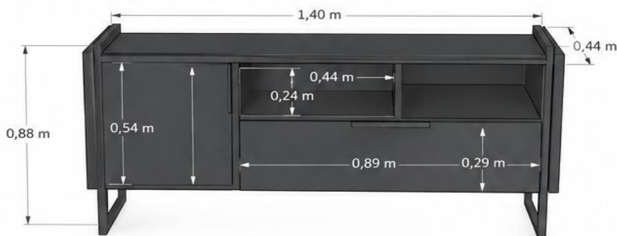
APARADOR COM ESTRUTURA METÁLICA - VISTA FRONTAL
