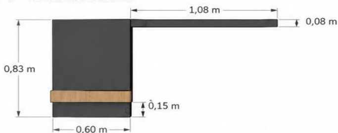
APARADOR COM ESTRUTURA METÁLICA - VISTA FRONTAL
