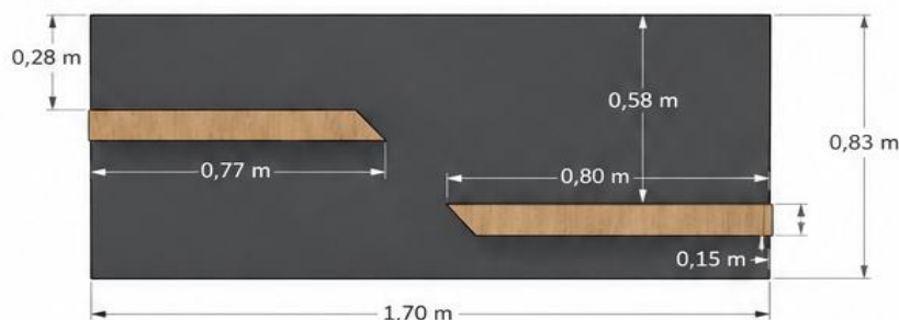
PRATELEIRA EM "L" - VISTA LATERAL DIREITA
